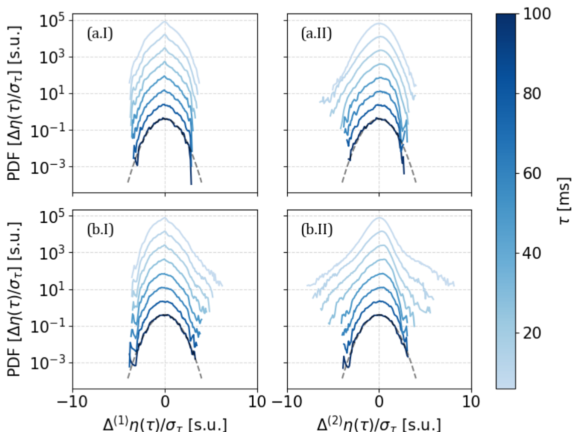
Figura 4.17: PDFs normalizadas (—) para las primeras (n.I) y segundas diferencias (n.II), con diferente delay \tau , de una señal con no linealidad baja (a) y alta (b). Las curvas se desplazaron verticalmente por claridad. Se muestra además para todos los casos la distribución Gaussiana de media cero y desviación unidad como referencia (---).
