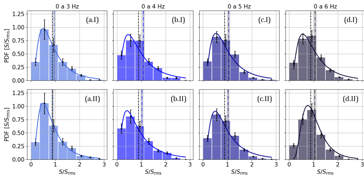
Figura 4.6: PDFs para la pendiente de las ondas normalizada ( S/S_{rms} ) de varias mediciones. Cada columna se corresponde a un rango de frecuencias, siendo (a) 0-3 Hz (b) 0-4 Hz (c) 0-5 Hz y (d) 0-6 Hz. La fila superior (n.I) se corresponde a la amplitud de 80 % y la inferior (n.II) a 120 %. Para cada una se muestra el ajuste por el modelo log-normal (—), el valor medio obtenido (---) con su incerteza y el valor teórico esperado de \sqrt{\pi}/2 (---).
