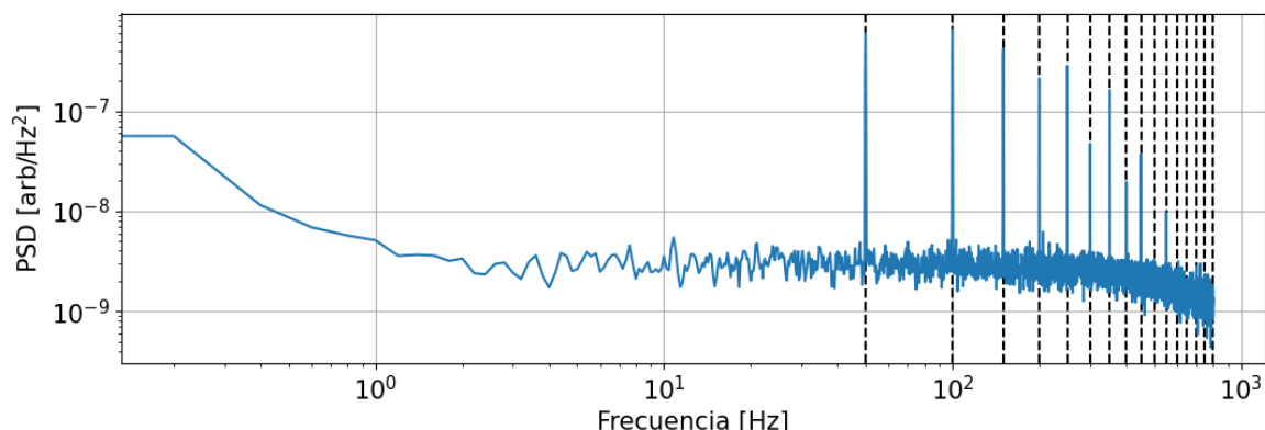
Figura 3.14: Densidad espectral de potencias para el ruido del sensor (—). Se marcan los múltiplos enteros de 50 Hz (---), que coincide con los picos.
