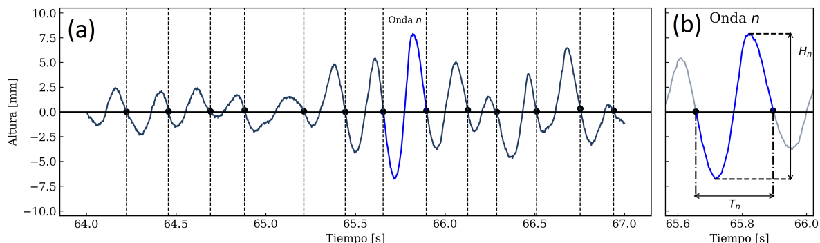
Figura 4.5: (a) Definición de ondas individuales para una medición típica, a partir de dos cruces de cero consecutivos en el mismo sentido. (b) Definición de la altura H_n y período T_n para la n -ésima onda individual de la señal.
