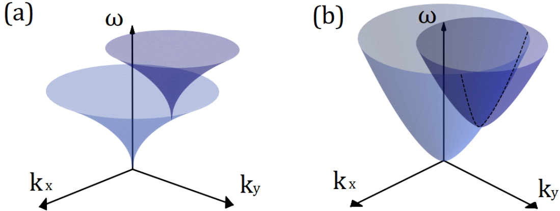
Figura 2.2: Método gráfico para hallar soluciones simultáneas a las condiciones de resonancia en el caso de triadas. (a) \alpha = 1/2 para gravedad, existe únicamente la solución trivial. (b) \alpha = 3/2 para capilar, existe una familia de soluciones (---).
