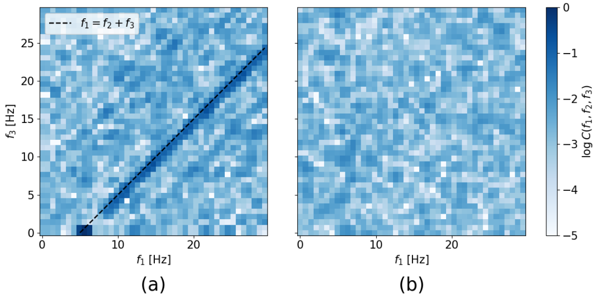
Figura 4.15: (a) Corte del volumen mostrado en la Figura 4.14 con f_2 = 5 \text{ Hz} . La línea (---) muestra la condición de resonancia para triadas. (b) Misma correlación calculada para ruido Gaussiano de la misma longitud y dispersión que la señal.
