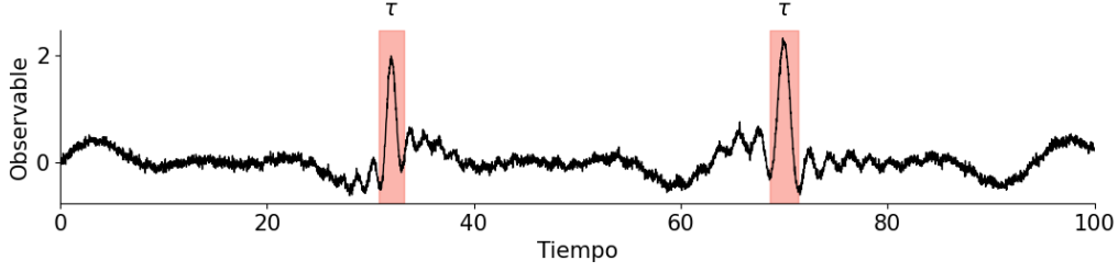
Figura 4.17: Esquema de un observable con comportamiento intermitente en escalas \tau . Adaptada de [40].
