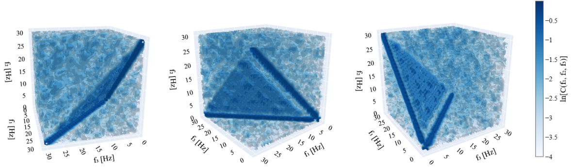
Figura 4.14: Distintas vistas de la correlación C(f_1, f_2, f_3) en escala logarítmica para la señal de 0-6 Hz y amplitud del 50%.
