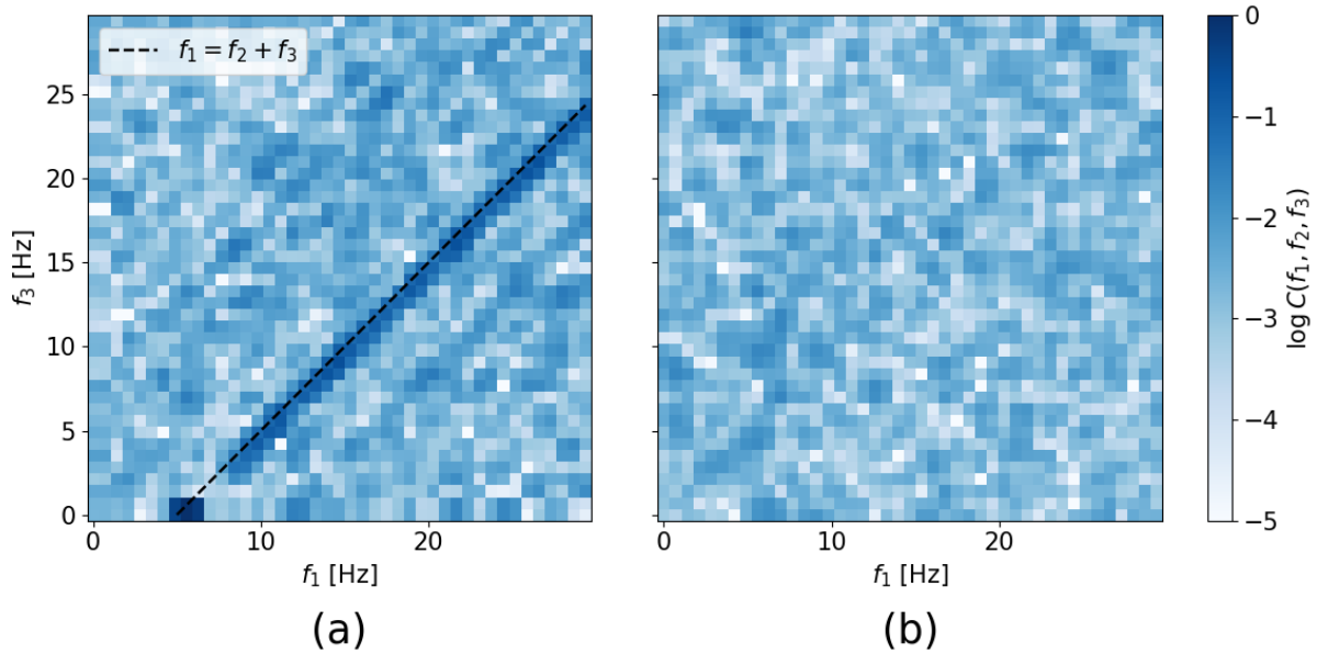
Figura 4.16: (a) Corte del volumen mostrado en la Figura 4.15 con f_2 = 5 Hz. La línea (---) muestra la condición de resonancia para triadas. (b) Misma correlación calculada para ruido Gaussiano de la misma longitud y dispersión que la señal.
