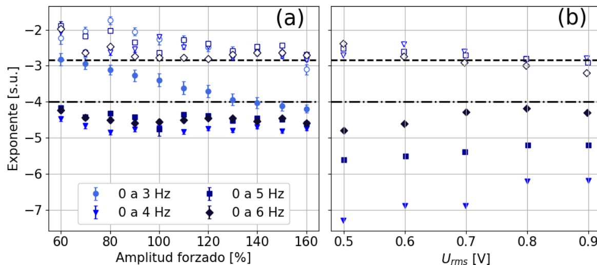
Figura 4.13: (a) Exponentes de la PSD obtenidos para ambos regímenes de la cascada de energía. En símbolos llenos (●) para el gravitatorio y en símbolos vacíos (○) para el capilar. Las líneas horizontales muestran la predicción teórica para los espectros de ZF, de -4 en gravedad (— · — ·) y -17/6 en capilar (---). (b) Resultados de la literatura para un experimento análogo en mercurio [38].
