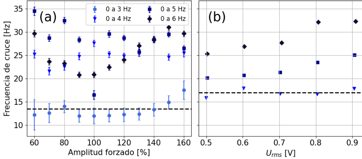
Figura 4.14: (a) Frecuencia de cruce de los regímenes de la PSD. La línea horizontal (---) muestra la predicción teórica para el agua destilada, de 13.5 Hz aproximadamente. (b) Resultados de la literatura para un experimento análogo en mercurio [38]. Aquí la frecuencia de cruce teórica está en 17 Hz aproximadamente.
