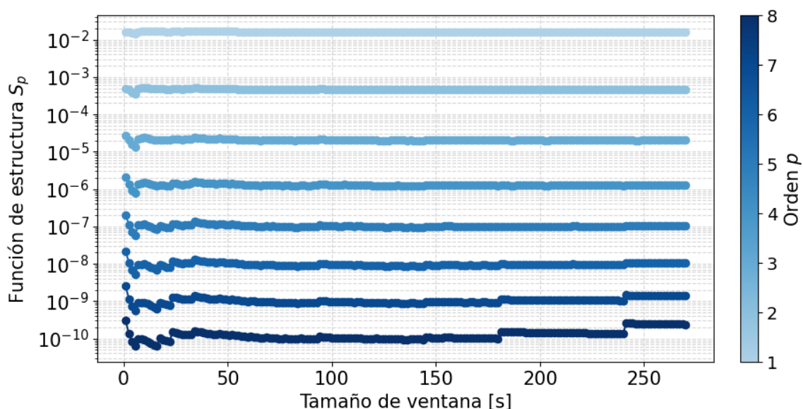
Figura 4.19: Funciones de estructura hasta el orden p = 8 para \tau = 8 ms con una longitud variable de la señal.
