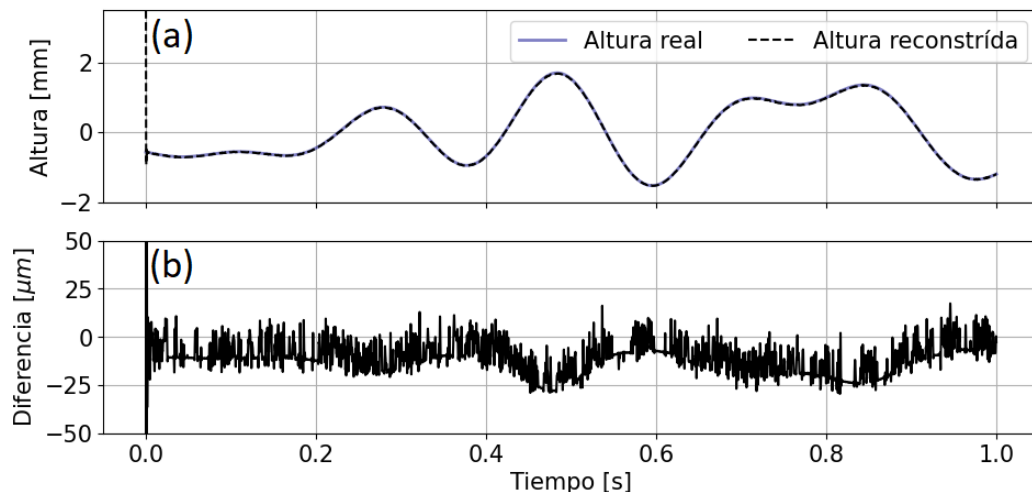
Figura 3.5: (a) Comparación de la altura sumergida, \Delta l , con la reconstruida, obtenida mediante la resolución numérica de la ecuación (3.7) y la técnica de demodulación homodina para el cálculo de la fase. (b) Diferencia entre ambas señales, de dos órdenes de magnitud menor.
