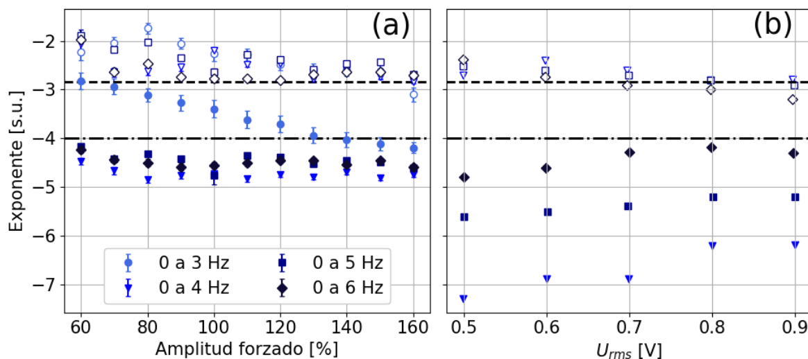
Figura 4.12: (a) Exponentes de la PSD obtenidos para ambos regímenes de la cascada de energía. En símbolos llenos (●) para el gravitatorio y en símbolos vacíos (○) para el capilar. Las líneas horizontales muestran la predicción teórica para los espectros de ZF de -4 en gravedad (— · —) y -17/6 en capilar (---). (b) Resultados de la literatura para un experimento análogo en mercurio [37].
