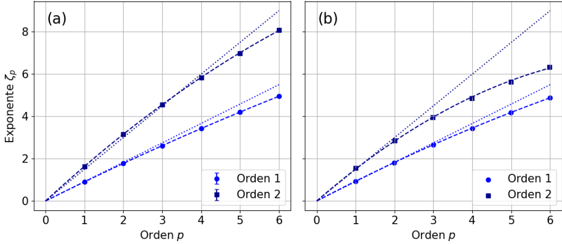
Figura 4.22: Exponentes \zeta_p obtenidos para las funciones de estructura S_p en el rango capilar (●) calculadas con las diferencias de orden uno y dos. (a) Este trabajo. (b) Falcon (2007) [37]. Se muestran además los ajustes realizados (---) por una función cuadrática \zeta_p = c_1 p - c_2 p^2/2 , cuyos resultados se encuentran en la Tabla 4.2, y el escalado esperado por análisis dimensional (.....).
