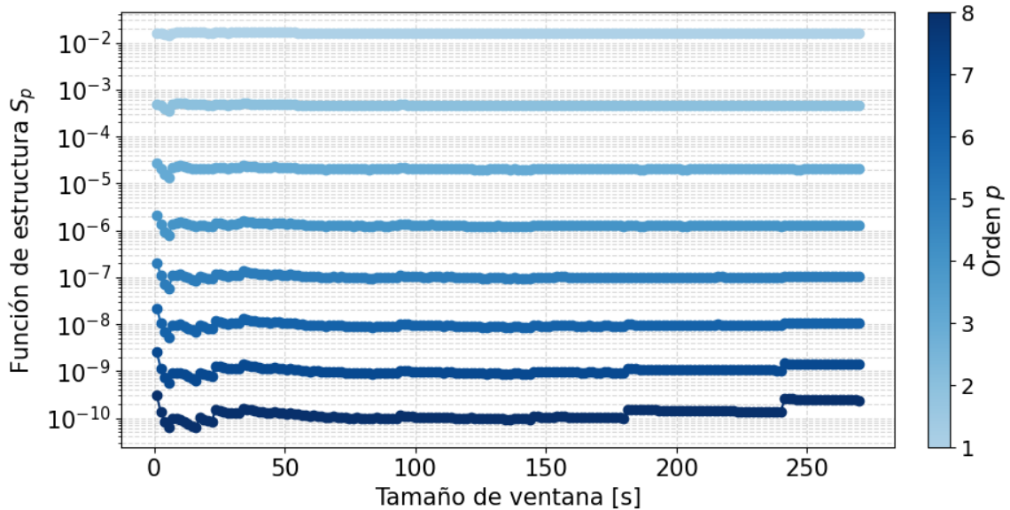
Figura 4.19: Funciones de estructura hasta el orden p = 8 para \tau = 8 ms con una longitud variable de la señal.
