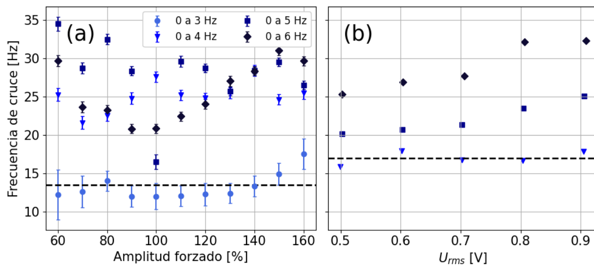
Figura 4.13: (a) Frecuencia de cruce de los regímenes de la PSD. La línea horizontal (---) muestra la predicción teórica para el agua destilada, de 13.5 Hz aproximadamente. (b) Resultados de la literatura para un experimento análogo en mercurio [37]. Aquí la frecuencia de cruce teórica está en 17 Hz aproximadamente.
