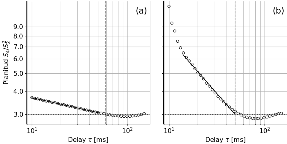
Figura 4.21: Planitud ( \circ ) en función del delay \tau para (a) las primeras diferencias y (b) las segundas diferencias. En ambos casos se muestra además un ajuste lineal para el rango donde se observa un comportamiento lineal (—). Las líneas punteadas (---) muestran el punto donde el ajuste interseca el valor 3, que se tomará como el tiempo de correlación. Los valores obtenidos son los de la Tabla 4.1.
