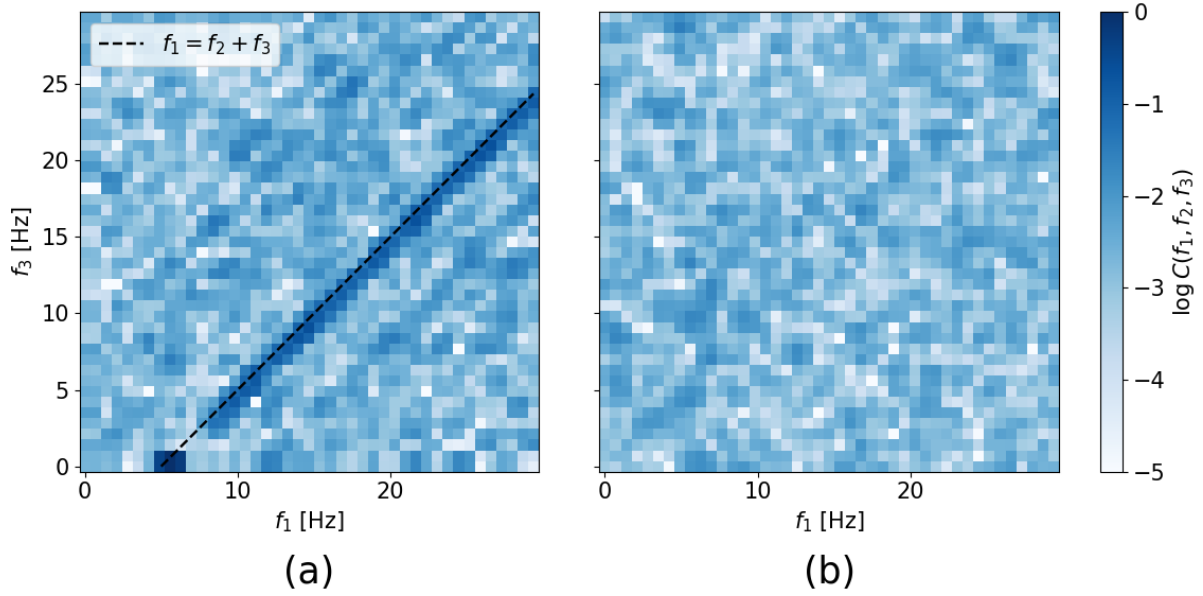
Figura 4.15: (a) Corte del volumen mostrado en la Figura 4.14 con f_2 = 5 Hz. La línea (---) muestra la condición de resonancia para triadas. (b) Misma correlación calculada para ruido Gaussiano de la misma longitud y dispersión que la señal.
