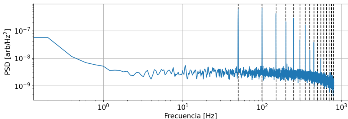
Figura 3.14: Densidad espectral de potencias para el ruido del sensor (—). Se marcan los múltiplos enteros de 50 Hz (---), que coincide con los picos.
