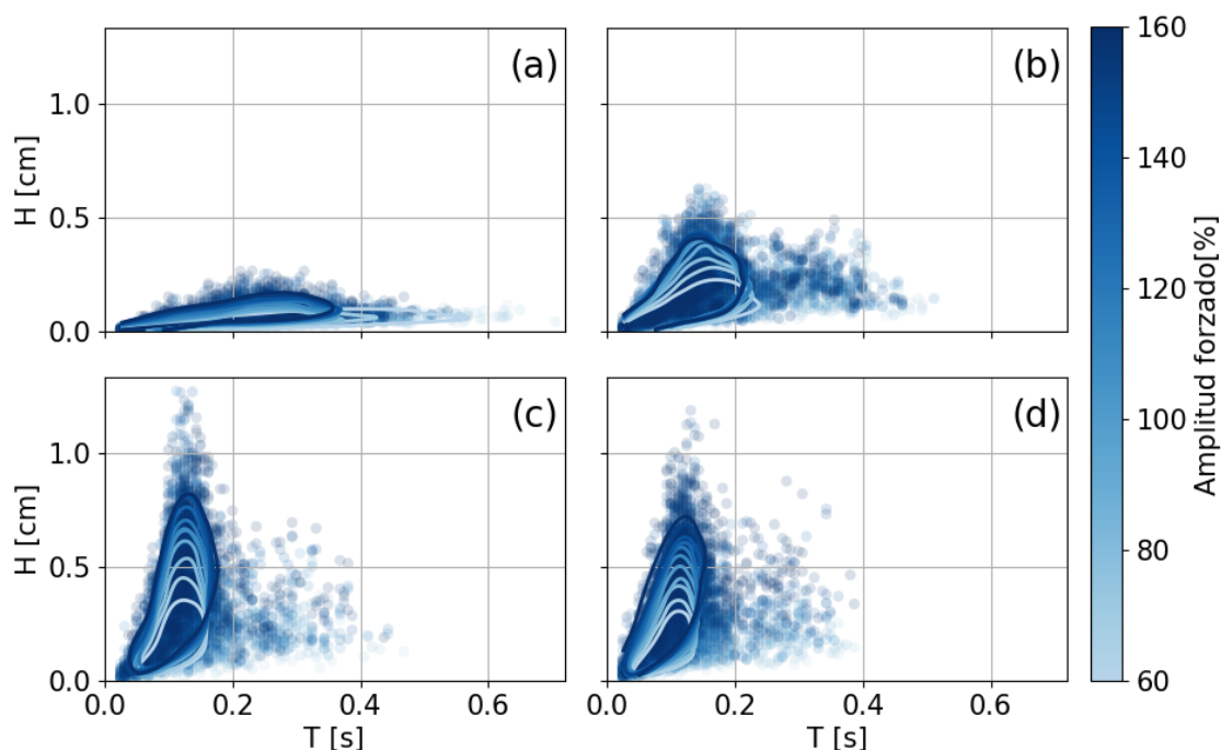
Figura 4.6: Distribución del conjunto de parámetros (T_n, H_n) para las ondas individuales de las distintas señales (a) 0-3 Hz (b) 0-4 Hz (c) 0-5 Hz (d) 0-6 Hz. Los contornos sólidos muestran la región que contiene al 67% de los puntos en cada caso.
