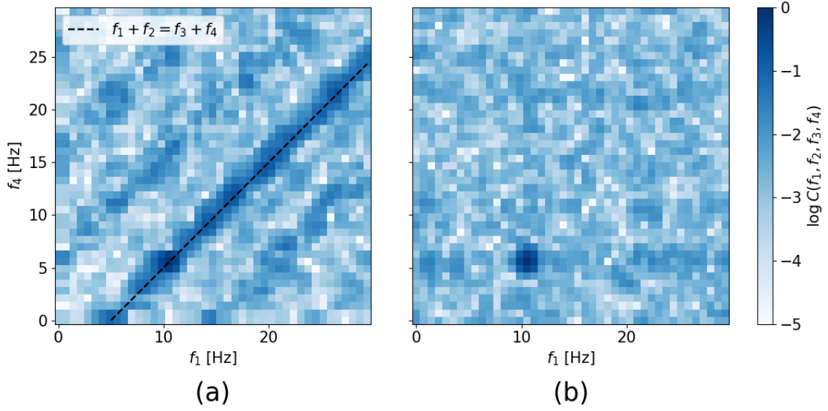
Figura 4.16: (a) Corte de la correlación C(f_1, f_2, f_3, f_4) en escala logarítmica, con f_2 = 5 Hz y f_3 = 10 Hz. La línea (---) muestra la condición de resonancia para cuartetos resonantes. (b) Misma correlación calculada para ruido Gaussiano de la misma longitud y dispersión que la señal.
