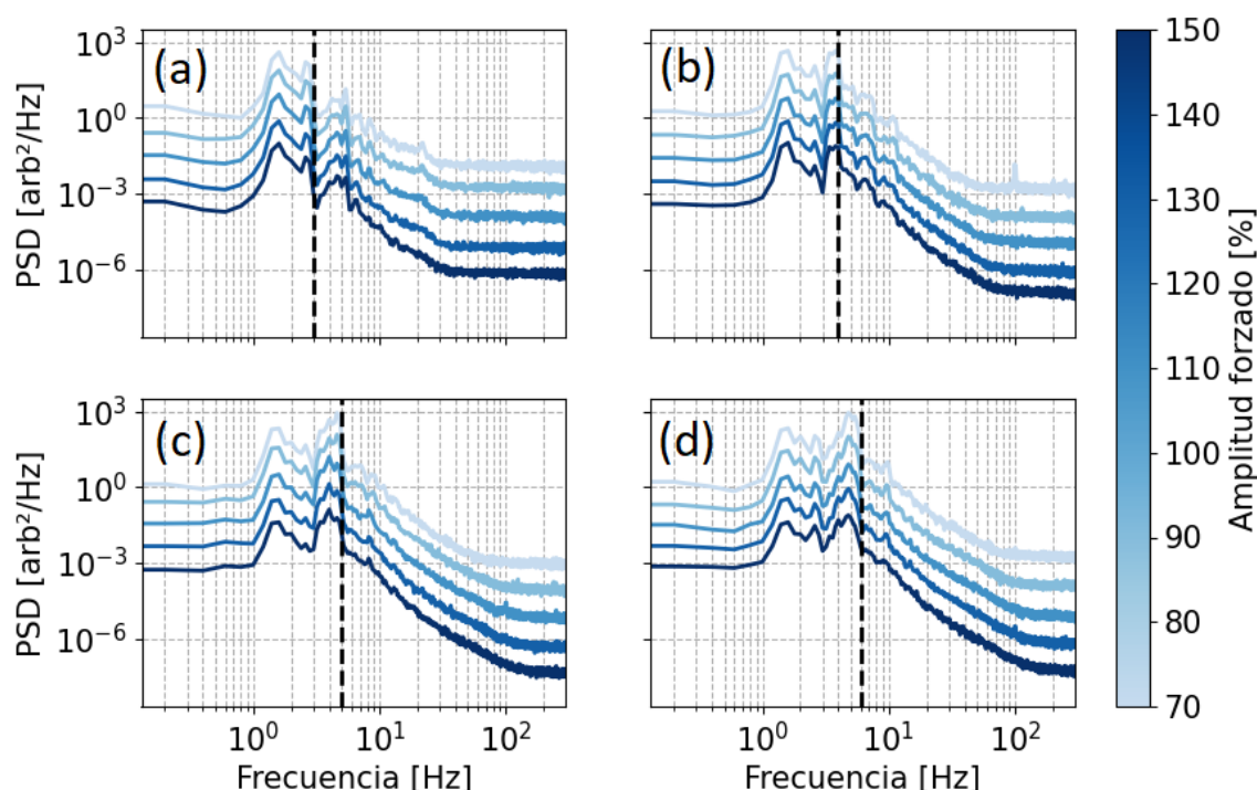
Figura 4.9: PSDs (—) para los distintos juegos de datos (a) 0-3 Hz (b) 0-4 Hz (c) 0-5 Hz (d) 0-6 Hz. Se muestra la frecuencia final del forzado (---) en cada caso. Las curvas se desplazaron verticalmente por claridad.
