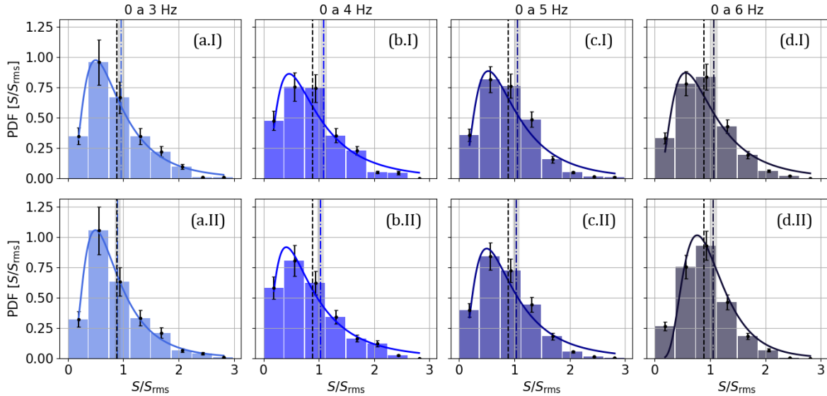
Figura 4.7: PDFs para la pendiente de las ondas normalizada ( S/S_{rms} ) de varias mediciones. Cada columna se corresponde a un rango de frecuencias, siendo (a) 0-3 Hz (b) 0-4 Hz (c) 0-5 Hz y (d) 0-6 Hz. La fila superior (n.I) se corresponde a la amplitud de 80% y la inferior (n.II) a 120%. Para cada una se muestra el ajuste por el modelo log-normal (—), el valor medio obtenido (---) con su incerteza y el valor teórico esperado de \sqrt{\pi}/2 (---).
