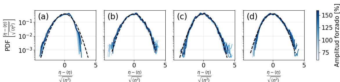
Figura 4.4: PDFs para la altura normalizada (—) de las distintas mediciones (a) 0-3 Hz (b) 0-4 Hz (c) 0-5 Hz y (d) 0-6 Hz. Se muestra, además, la distribución gaussiana de media cero y desviación unidad (---) a modo comparativo.
