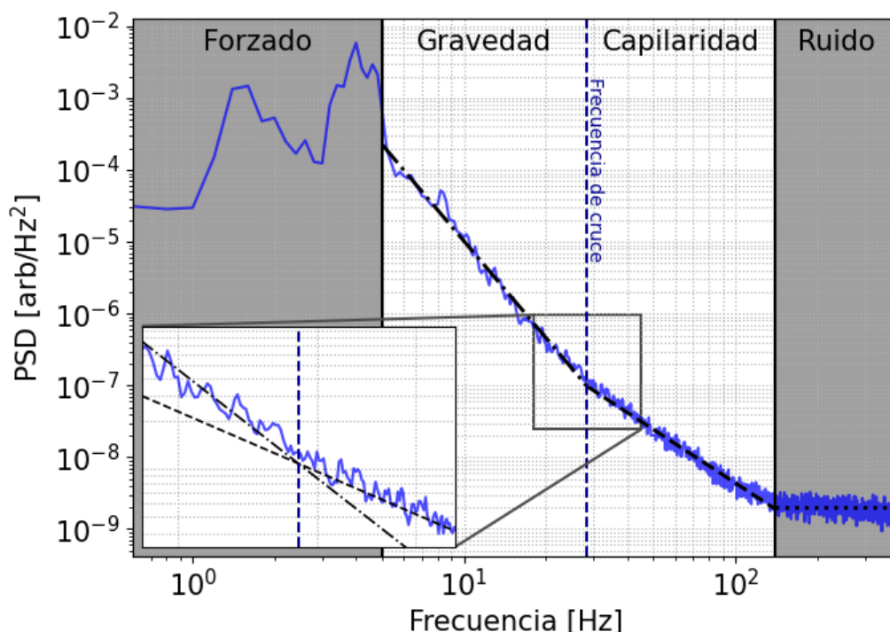
Figura 4.10: Ejemplo de procesamiento de la PSD media (—) para una de las señales. Las regiones más oscuras se corresponden con las escalas de inyección a frecuencias bajas y la de ruido a escalas chicas. La región sin colorear es el rango intermedio que se ajustó por completo mediante una función lineal a tramos continua. Cada tramo del ajuste resultante se muestra con líneas (---) y (-.-.-). Se muestra además la frecuencia de cruce obtenida, marcada verticalmente (-.-.-). Inset: Aumento de la región alrededor de la frecuencia de cruce donde cambia la pendiente de las rectas. Éstas se extendieron para apreciar el cambio de la pendiente en la PSD más claramente.
