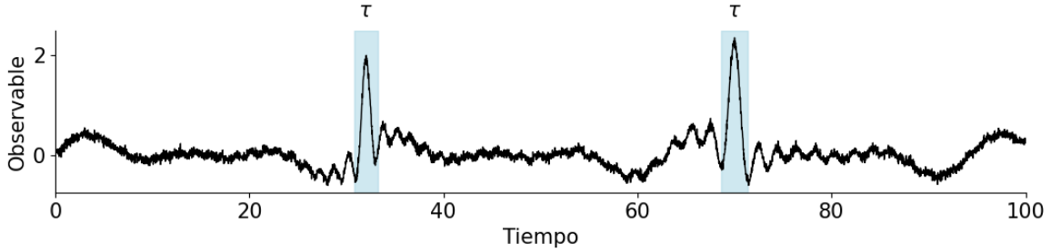
Figura 4.17: Esquema de un observable con comportamiento intermitente en escalas \tau . Adaptada de [40].
