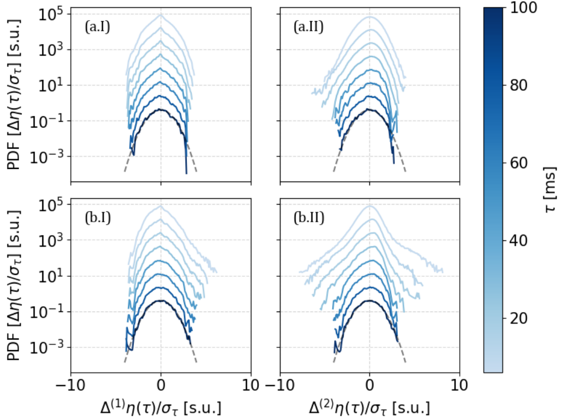
Figura 4.18: PDFs normalizadas (—) para las primeras (n.I) y segundas diferencias (n.II), con diferente delay \tau , de una señal con no linealidad baja (a) y alta (b). Las curvas se desplazaron verticalmente por claridad. Se muestra además para todos los casos la distribución Gaussiana de media cero y desviación unidad como referencia (---).
