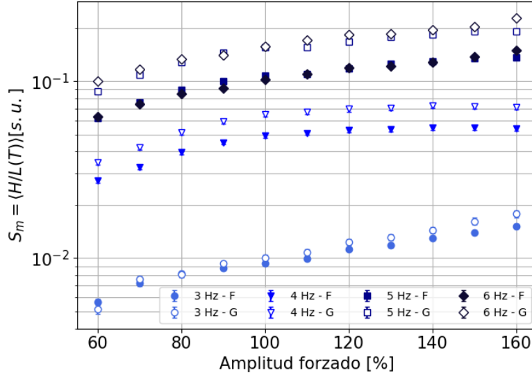
Figura 4.8: Pendiente media de las ondas para las distintas mediciones. Se muestran las aproximaciones utilizando la relación de dispersión de gravedad en profundidad infinita (G) y la completa (F) para obtener la longitud de onda L(T) .
