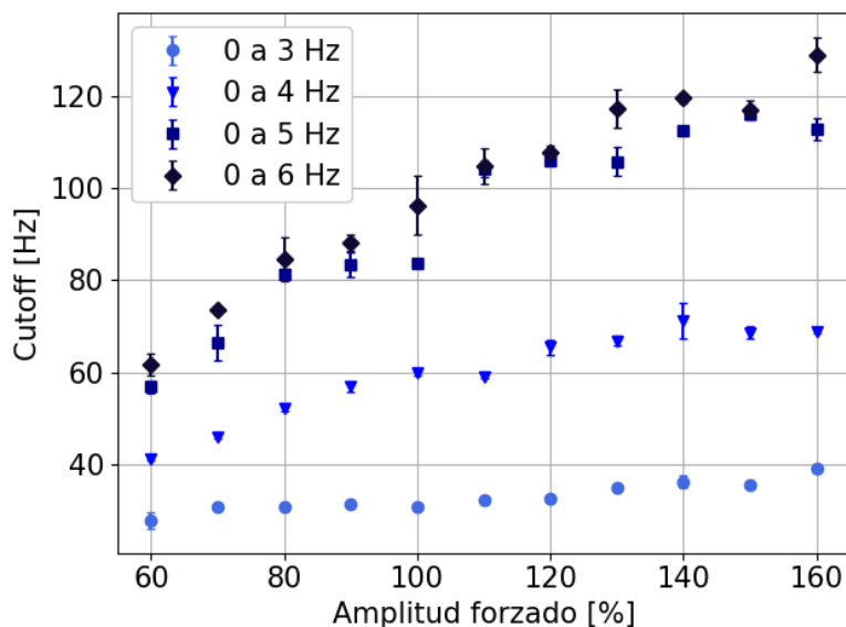
Figura 4.11: Frecuencia de corte del espectro obtenida para las distintas mediciones.
