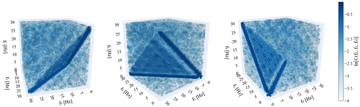
Figura 4.14: Distintas vistas de la correlación C(f_1, f_2, f_3) en escala logarítmica para la señal de 0-6 Hz y amplitud del 100%.
