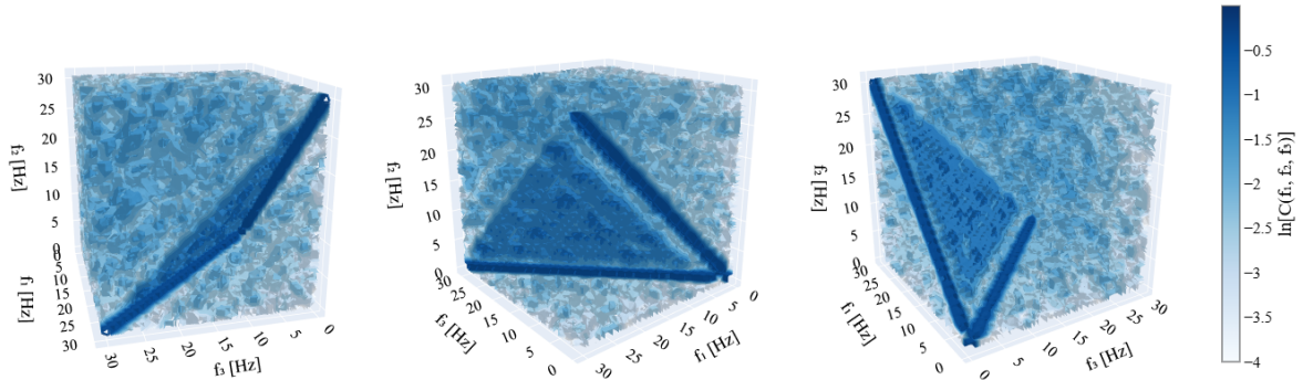
Figura 4.14: Distintas vistas de la correlación C(f_1, f_2, f_3) en escala logarítmica para la señal de 0-6 Hz y amplitud del 100 %.
