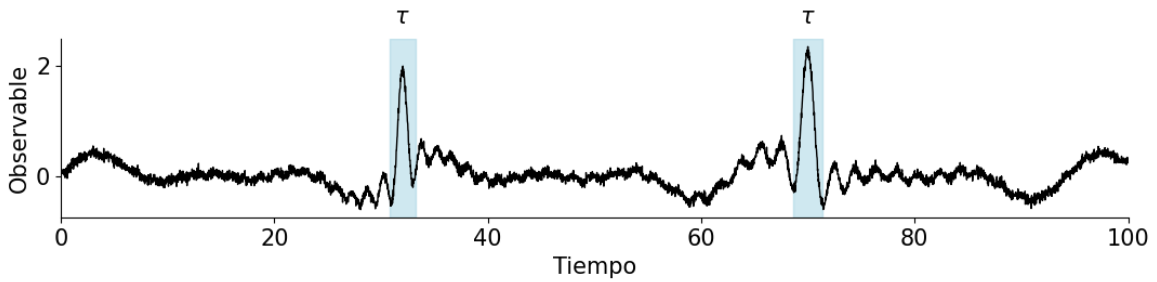
Figura 4.17: Esquema de un observable con comportamiento intermitente en escalas \tau . Adaptada de [41].
