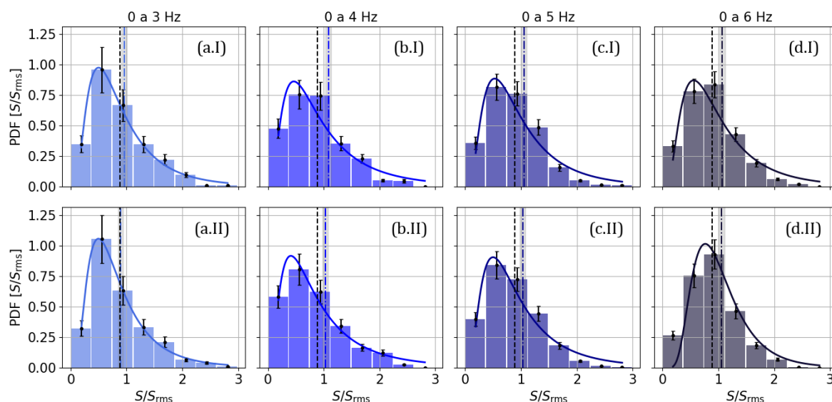
Figura 4.7: PDFs para la pendiente de las ondas normalizada (S/S_{rms}) de varias mediciones. Cada columna se corresponde a un rango de frecuencias, siendo (a) 0-3 Hz (b) 0-4 Hz (c) 0-5 Hz y (d) 0-6 Hz. La fila superior (n.I) se corresponde a la amplitud de 80% y la inferior (n.II) a 120%. Para cada una se muestra el ajuste por el modelo log-normal (—), el valor medio obtenido (---) con su incerteza y el valor teórico esperado de \sqrt{\pi}/2 (---).
