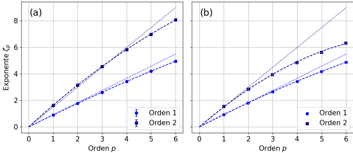
Figura 4.22: Exponentes \zeta_p obtenidos para las funciones de estructura S_p en el rango capilar (●) calculadas con las diferencias de orden uno y dos. (a) Este trabajo. (b) Falcon (2007) [38]. Se muestran además los ajustes realizados (---) por una función cuadrática \zeta_p = c_1 p - c_2 p^2/2 , cuyos resultados se encuentran en la Tabla 4.2, y el escalado esperado por análisis dimensional (.....).
