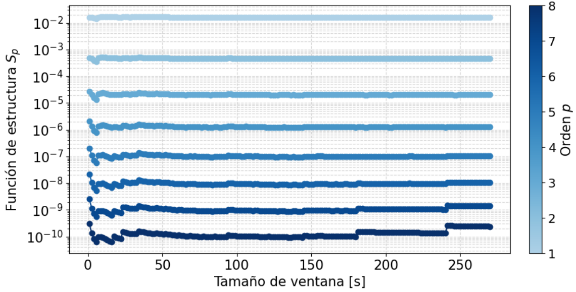
Figura 4.21: Funciones de estructura hasta el orden p = 8 para \tau = 8 ms con una longitud variable de la señal.
