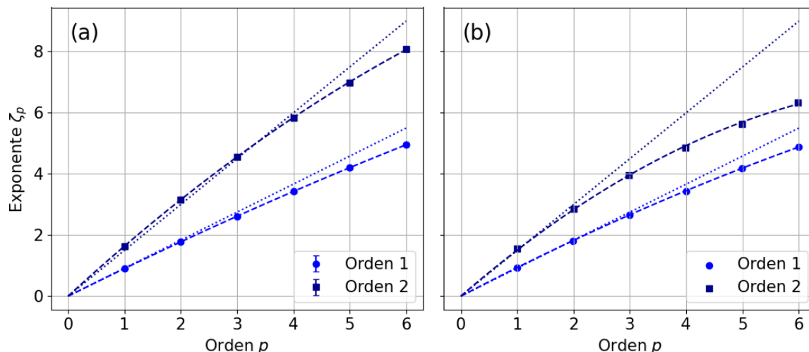
Figura 4.24: Exponentes \zeta_p obtenidos para las funciones de estructura S_p en el rango capilar (●) calculadas con las diferencias de orden uno y dos. (a) Este trabajo. (b) Falcon (2007) [38]. Se muestran además los ajustes realizados (---) por una función cuadrática \zeta_p = c_1 p - c_2 p^2 / 2 , cuyos resultados se encuentran en la Tabla 4.3, y el escalado esperado por análisis dimensional (.....).
