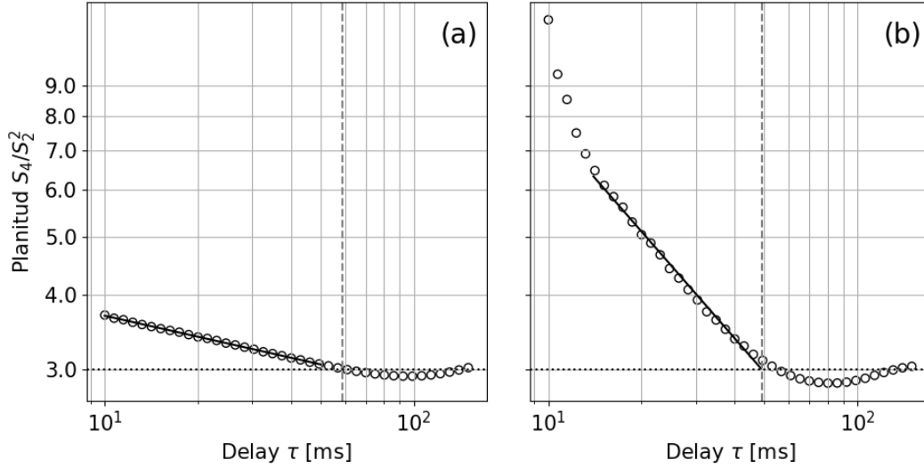
Figura 4.23: Planitud ( \circ ) en función del delay \tau para (a) las primeras diferencias y (b) las segundas diferencias. En ambos casos se muestra además un ajuste lineal para el rango donde se observa un comportamiento lineal (—). Las líneas punteadas (---) muestran el punto donde el ajuste interseca el valor 3, que se tomará como el tiempo de correlación. Los valores obtenidos son los de la Tabla 4.2.
