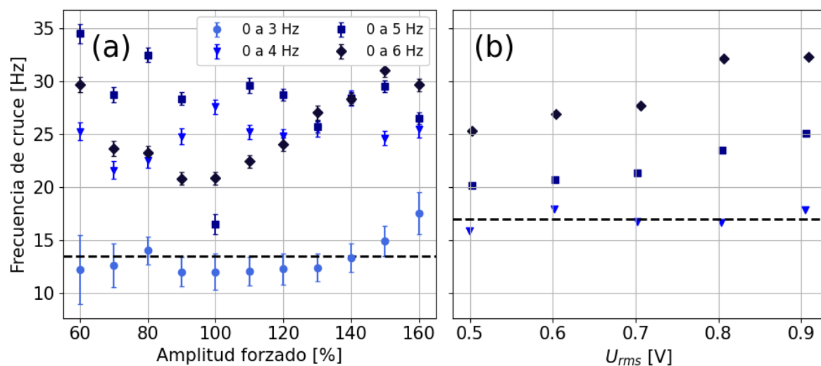
Figura 4.13: (a) Frecuencia de cruce de los regímenes de la PSD. La línea horizontal (— — —) muestra la predicción teórica para el agua destilada, de 13.5 Hz aproximadamente. (b) Resultados de la literatura para un experimento análogo en mercurio [14]. Aquí la frecuencia de cruce teórica está en 17 Hz aproximadamente.
