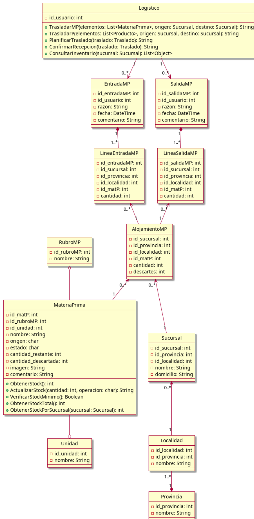
Figura 4.26: Diagrama de clases - Vista traslado de materias primas
