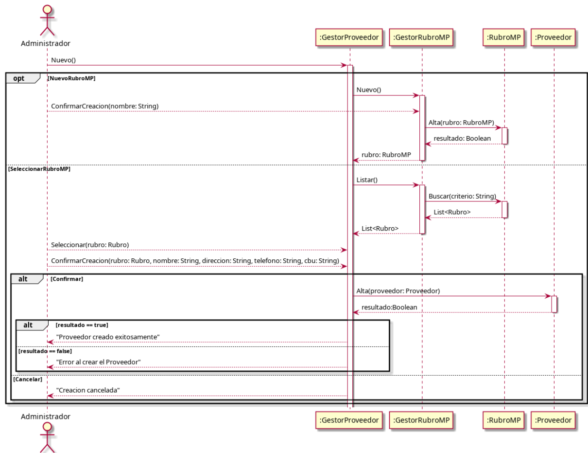
Figura 4.45: Diagrama de secuencia — CU10 - Nuevo proveedor
