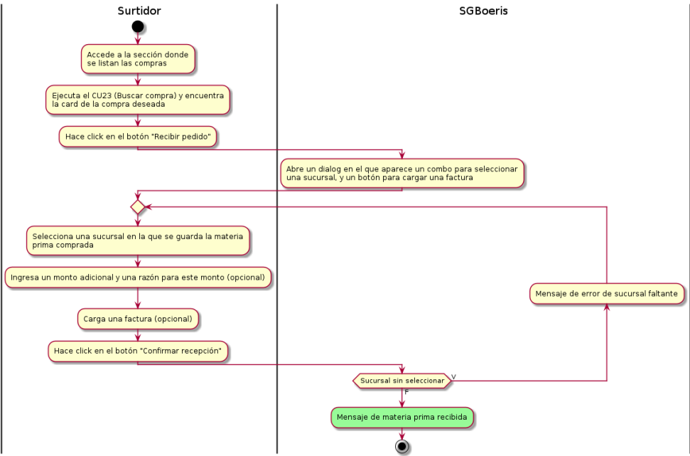
Figura 4.15: Diagrama de actividad — CU27 - Recibir compra MP
