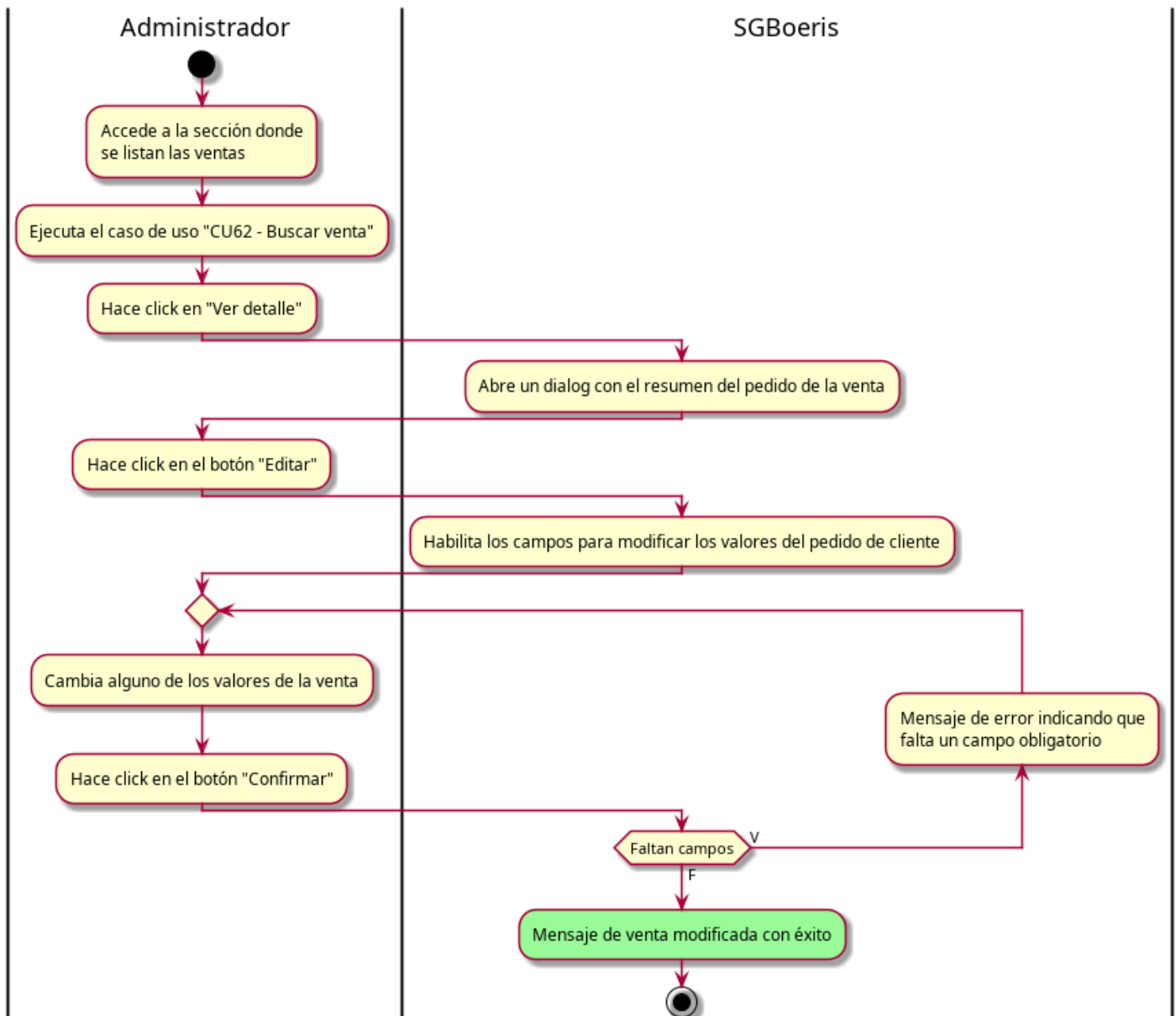
Figura 8.5: Diagrama de actividad — CU61 - Modificar venta
