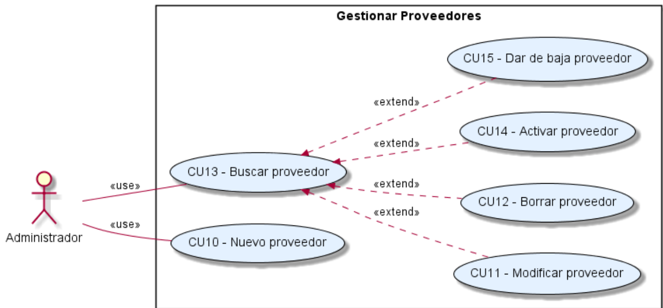
Figura 4.6: Diagrama de casos de uso para la gestión de proveedores
