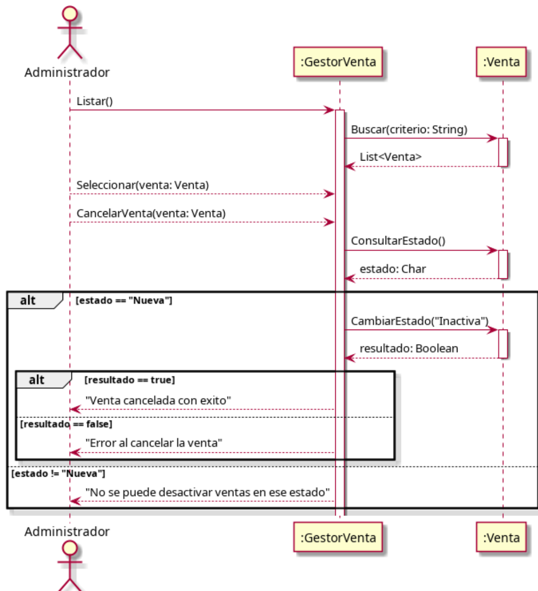
Figura 4.58: Diagrama de secuencia — CU68 - Cancelar venta
