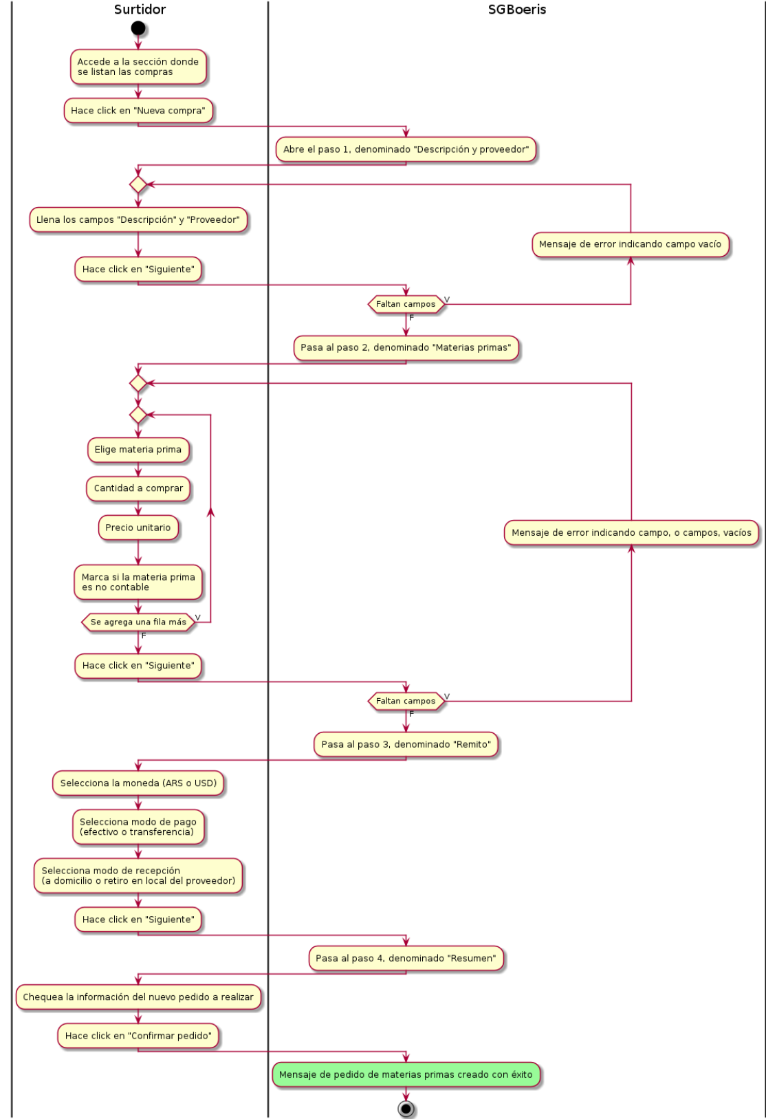
Figura 4.14: Diagrama de actividad — CU22 - Nueva compra MP
