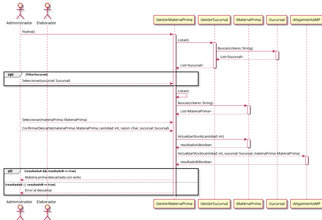
Figura 4.50: Diagrama de secuencia — CU42 - Descartar materia prima
