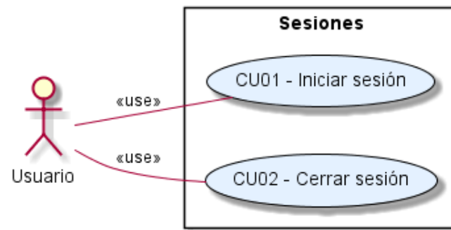
Figura 4.4: Diagrama de casos de uso para sesiones
