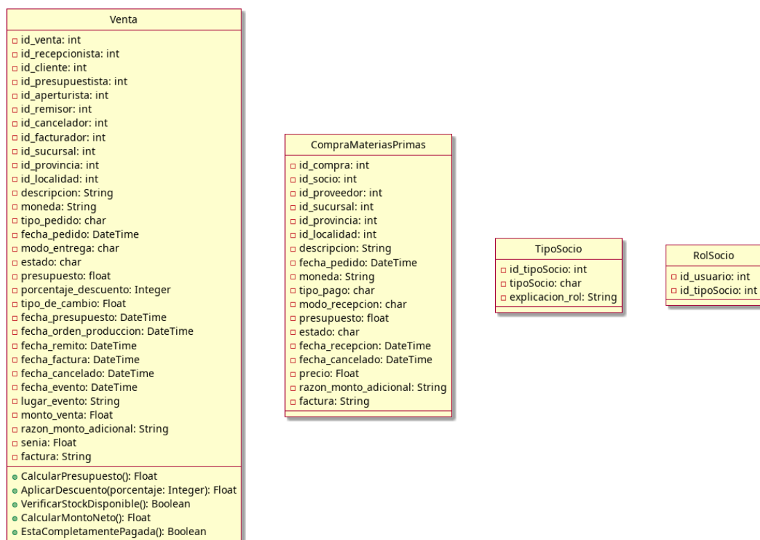
Figura 4.32: Diagrama de clases - Ficha técnica de clases (parte 2)
