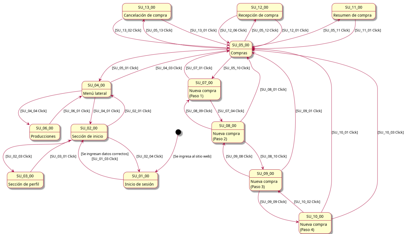
Figura 4.60: Diagrama de transición de escenarios - Surtidor
