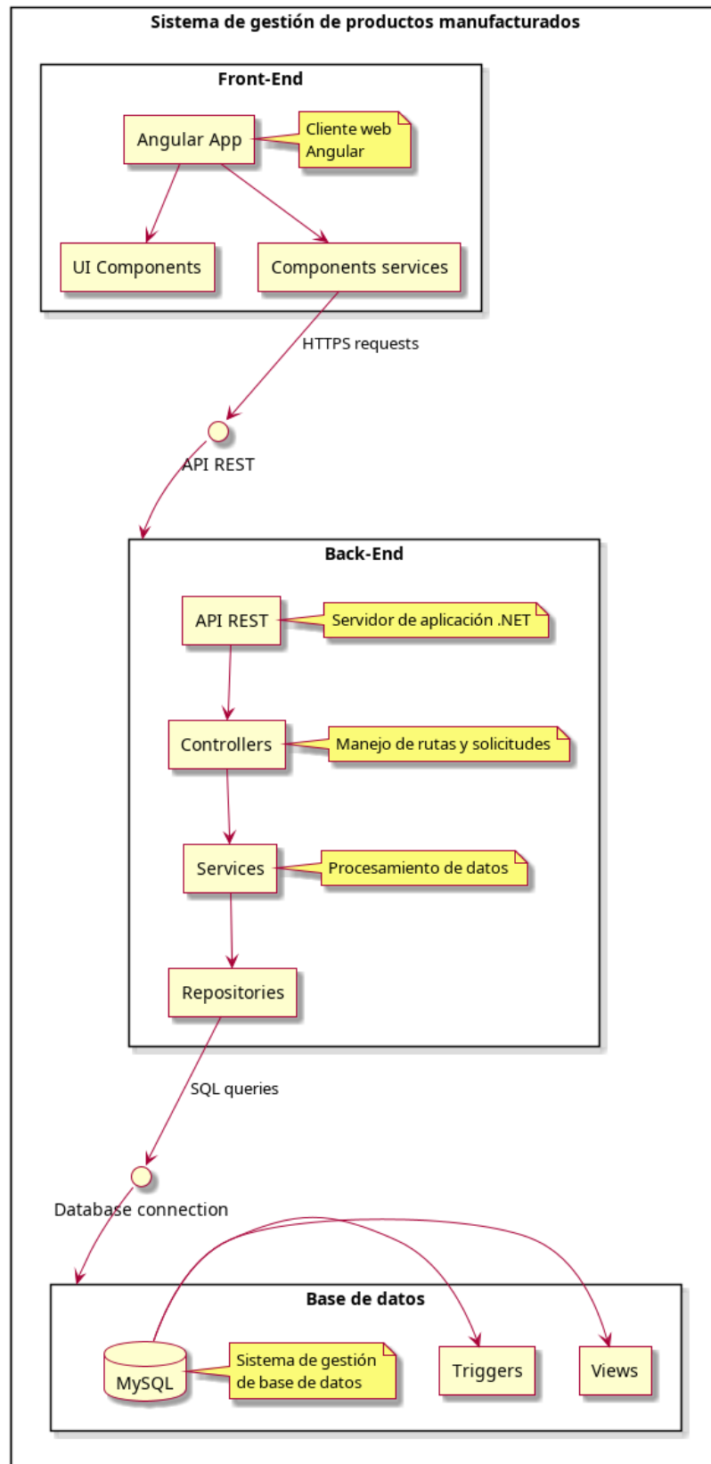
Figura 5.1: Arquitectura de tres capas
