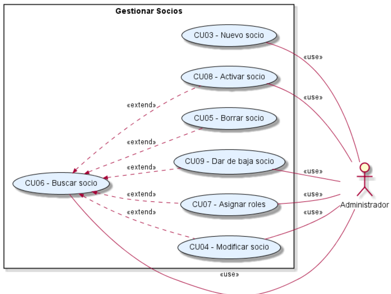
Figura 4.5: Diagrama de casos de uso para la gestión de socios
