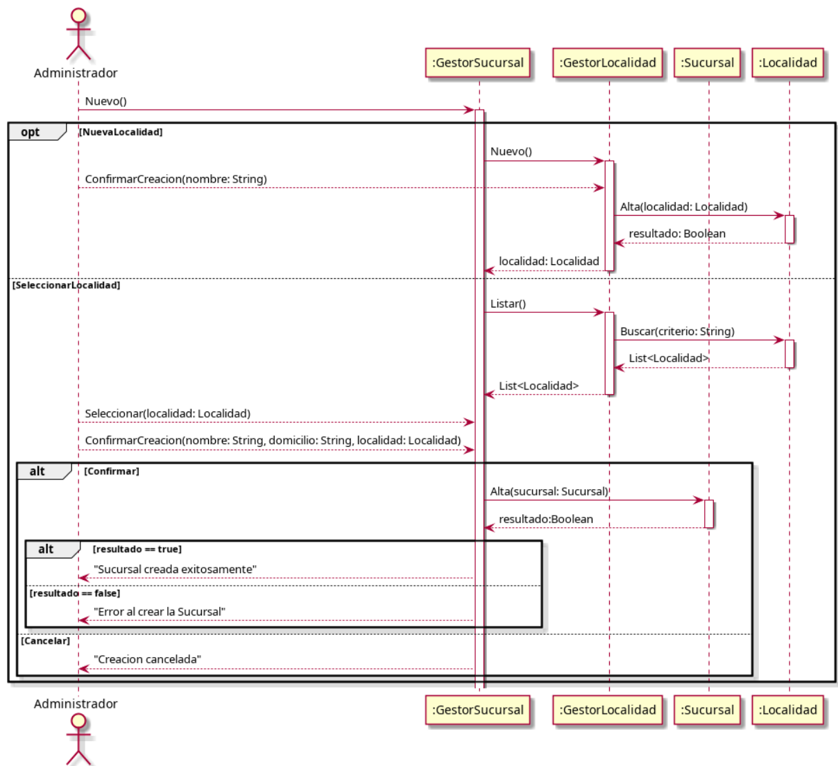
Figura 4.46: Diagrama de secuencia — CU16 - Nueva sucursal
