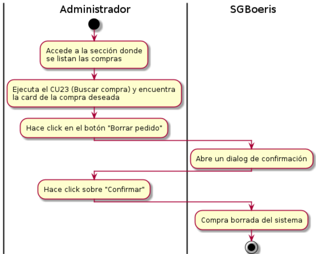
Figura 8.4: Diagrama de actividad — CU24 - Borrar compra MP
