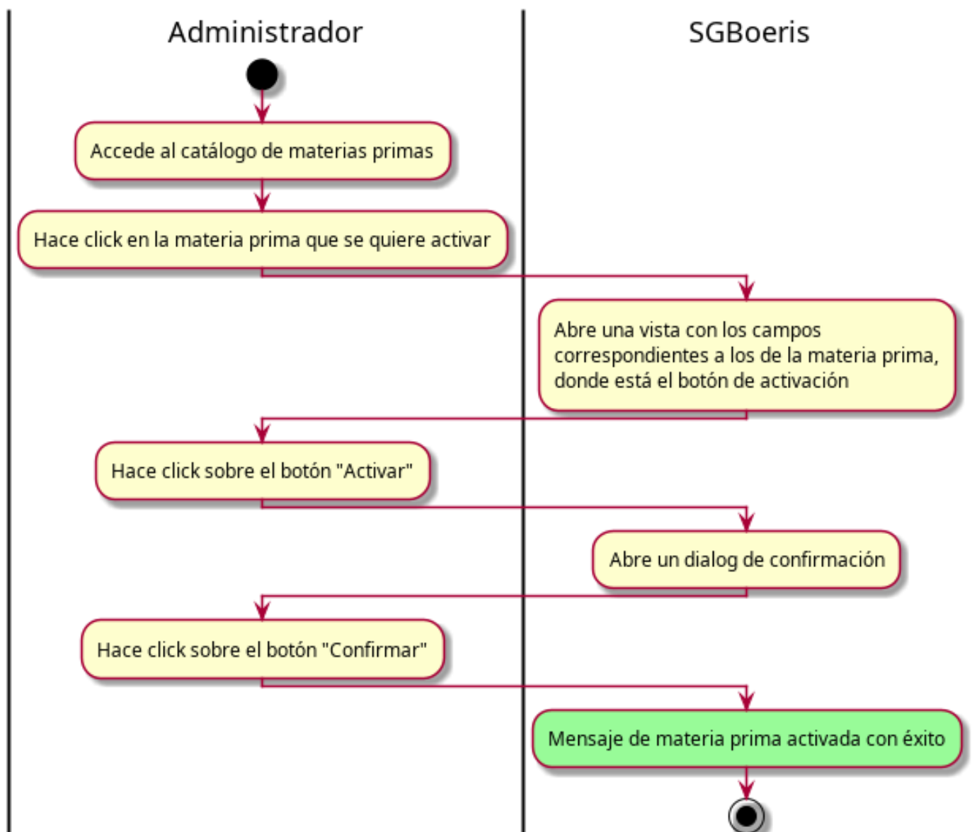
Figura 8.12: Diagrama de actividad — CU43 - Activar materia prima
