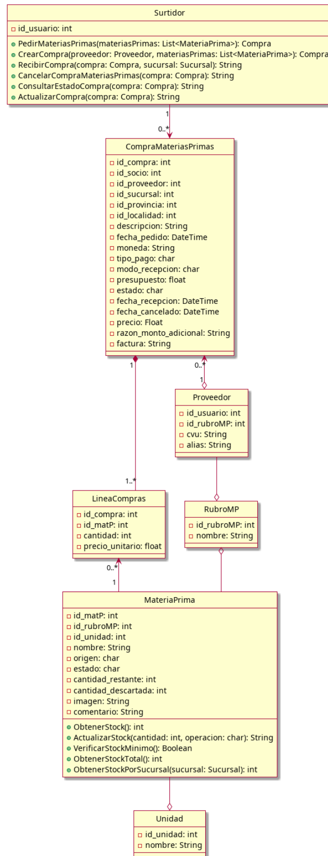
Figura 4.24: Diagrama de clases - Vista compras
