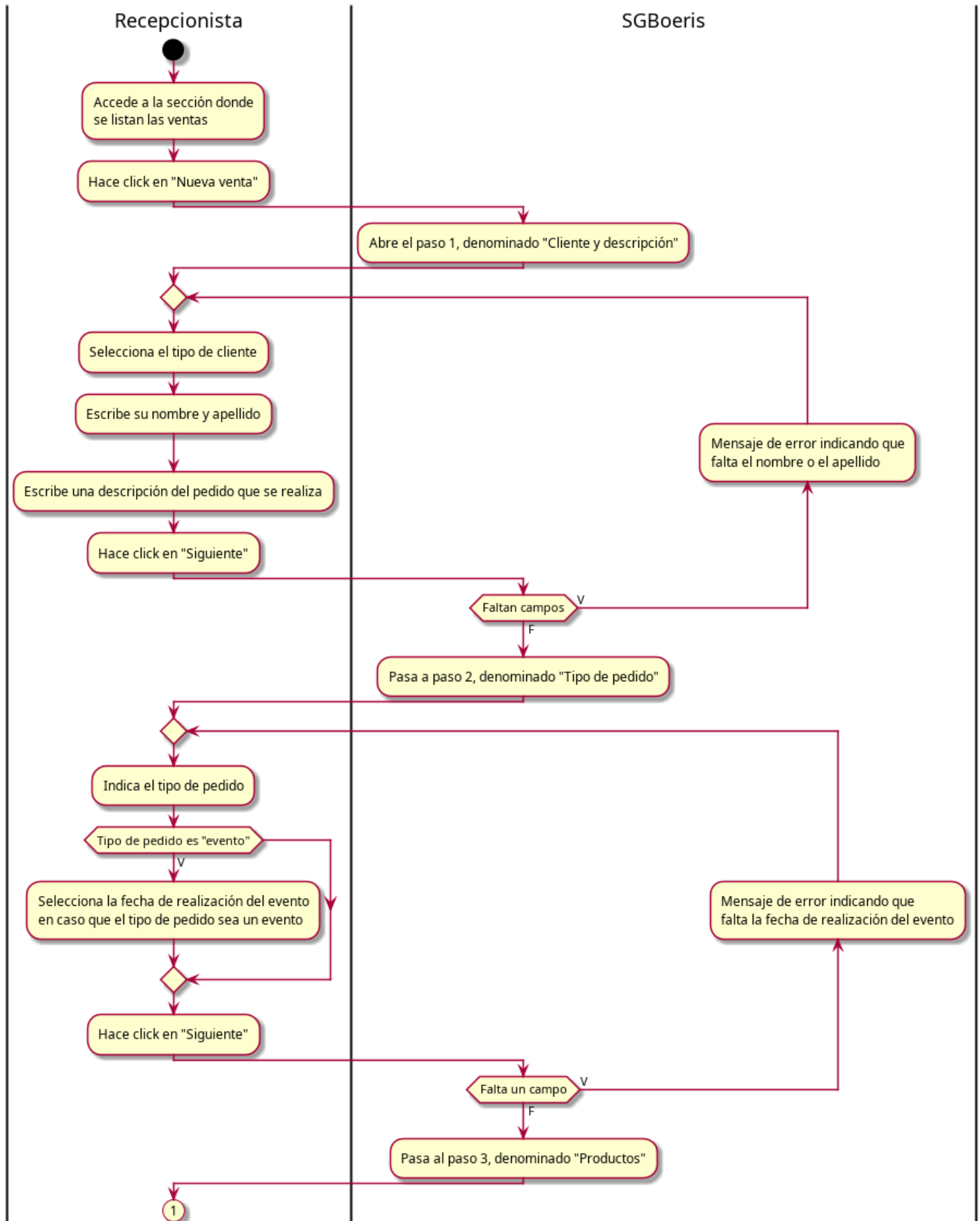
Figura 4.16: Diagrama de actividad — CU60 - Nueva venta (Parte 1)
