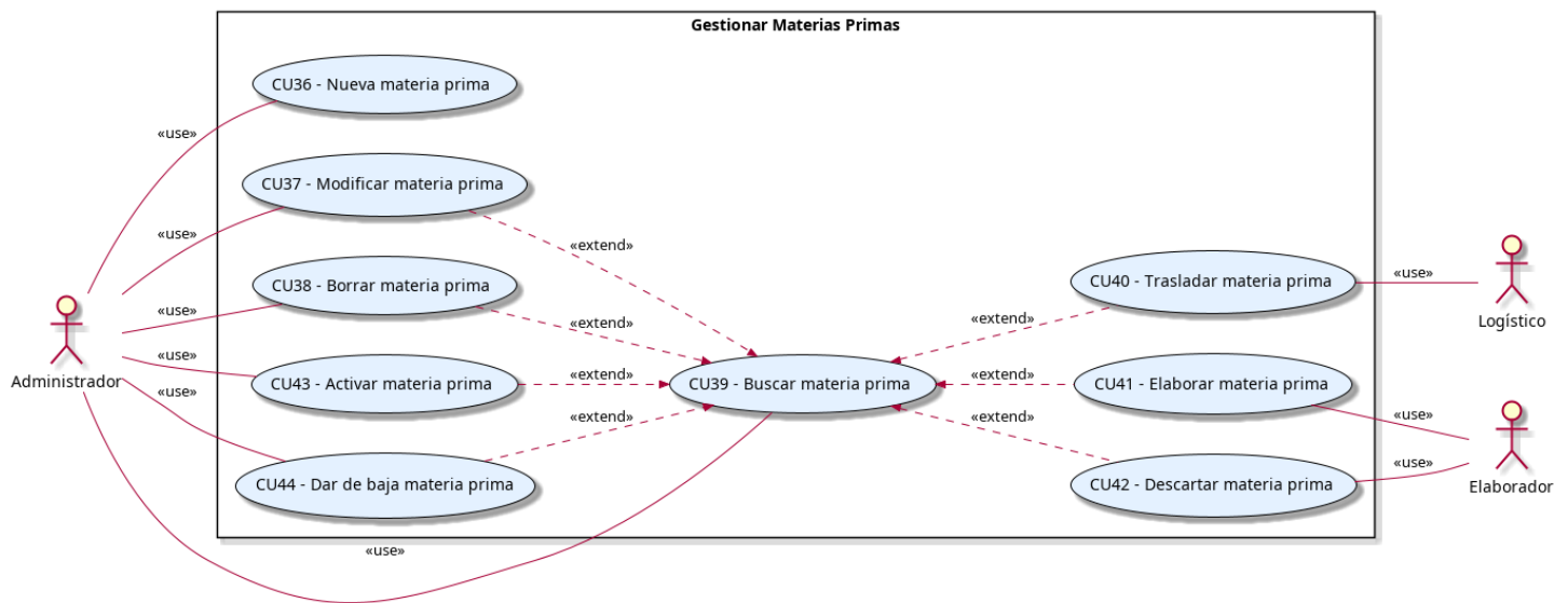
Figura 4.10: Diagrama de casos de uso para la gestión de materias primas
