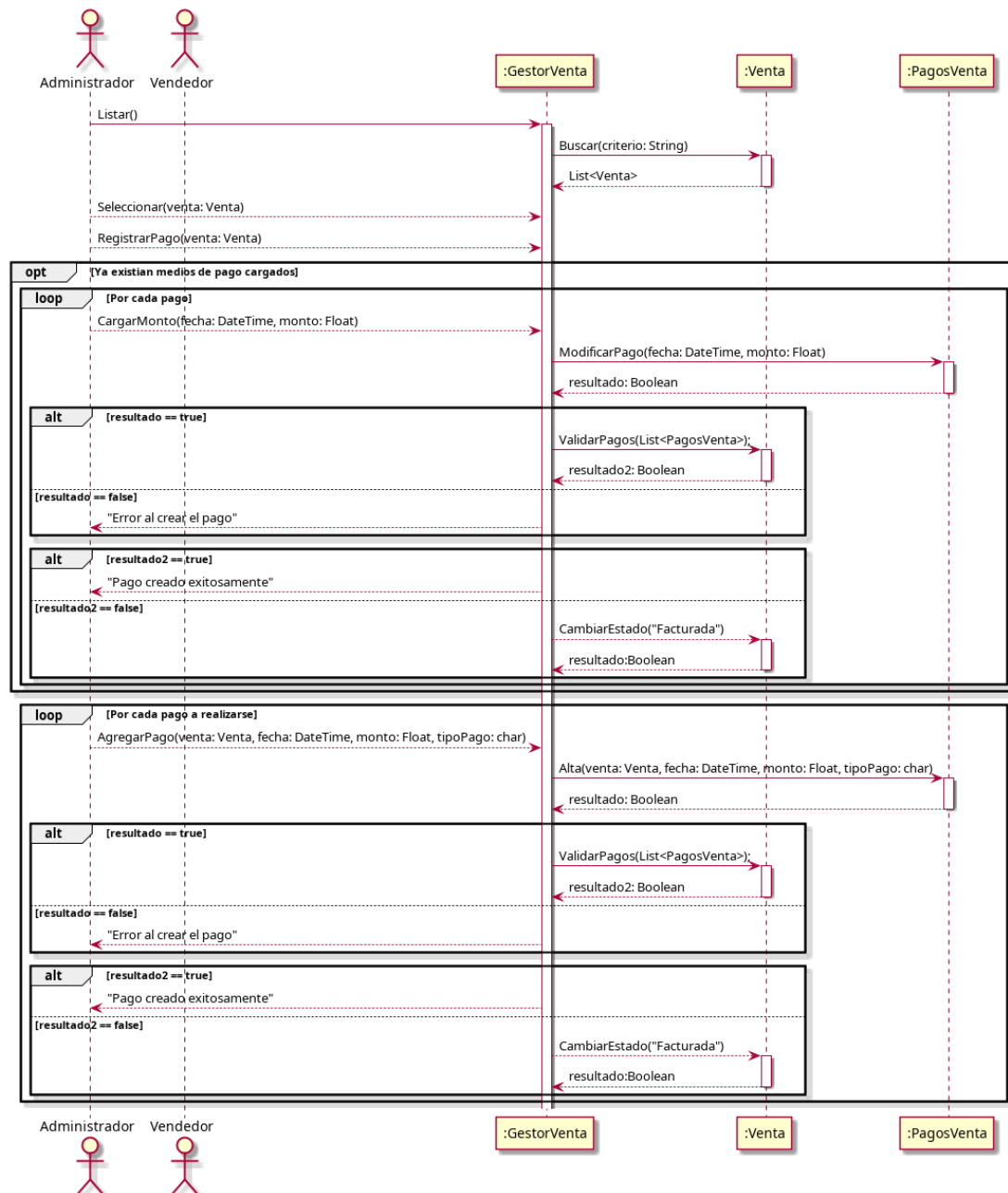
Figura 4.57: Diagrama de secuencia — CU67 - Recibir pago
