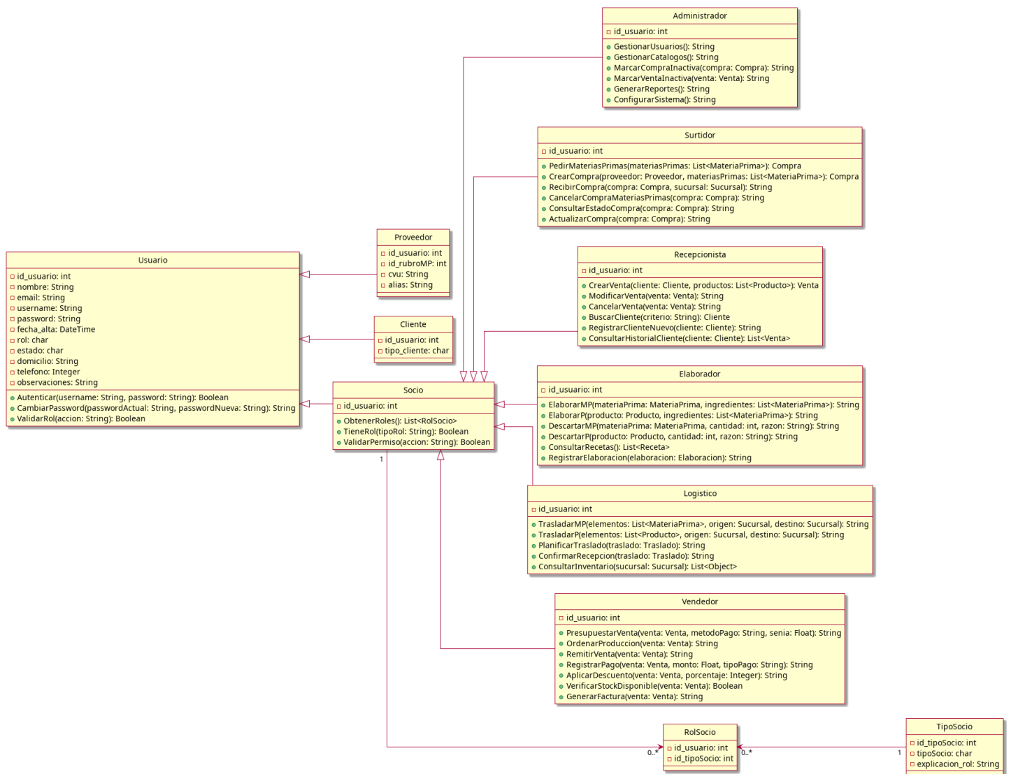
Figura 4.23: Diagrama de clases - Vista sistema
