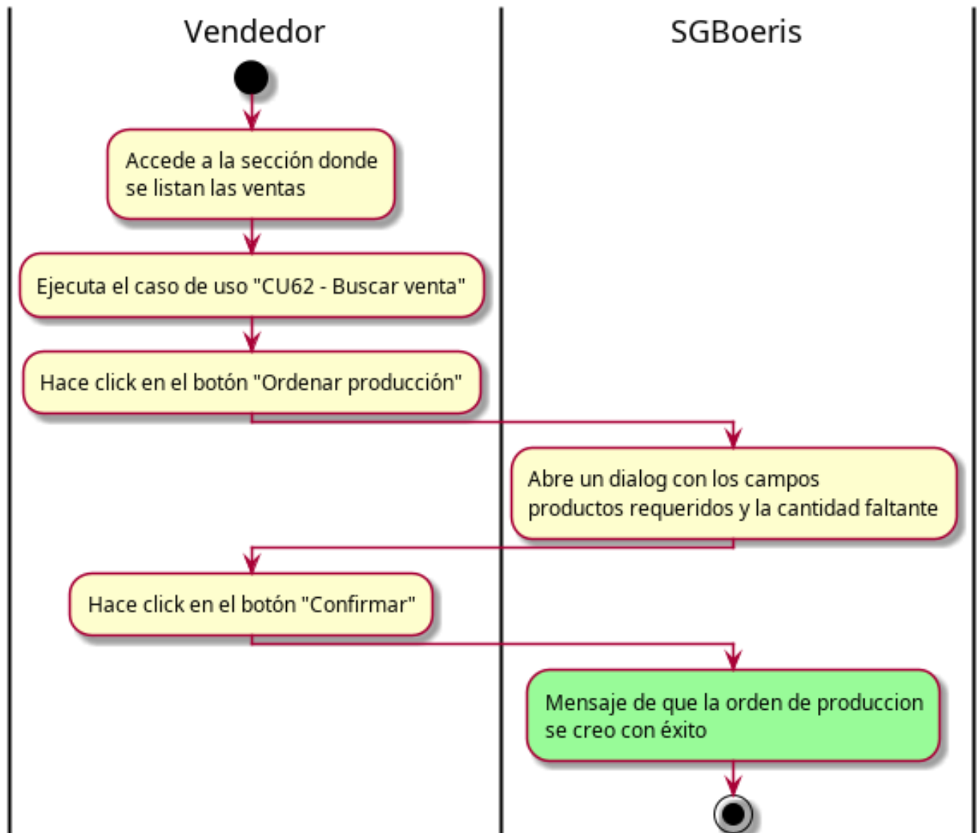
Figura 4.19: Diagrama de actividad — CU65 - Ordenar producción venta
