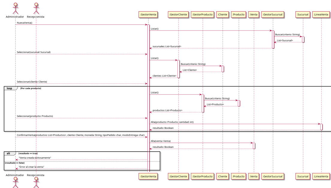
Figura 4.53: Diagrama de secuencia — CU60 - Nueva venta
