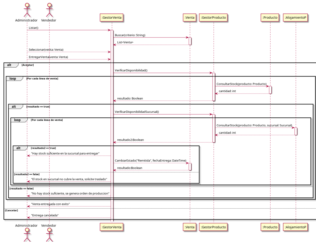
Figura 4.56: Diagrama de secuencia — CU66 - Remitir venta
