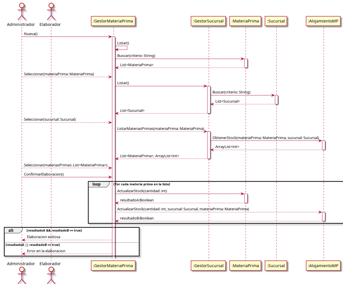
Figura 4.49: Diagrama de secuencia — CU41 - Elaborar materia prima
