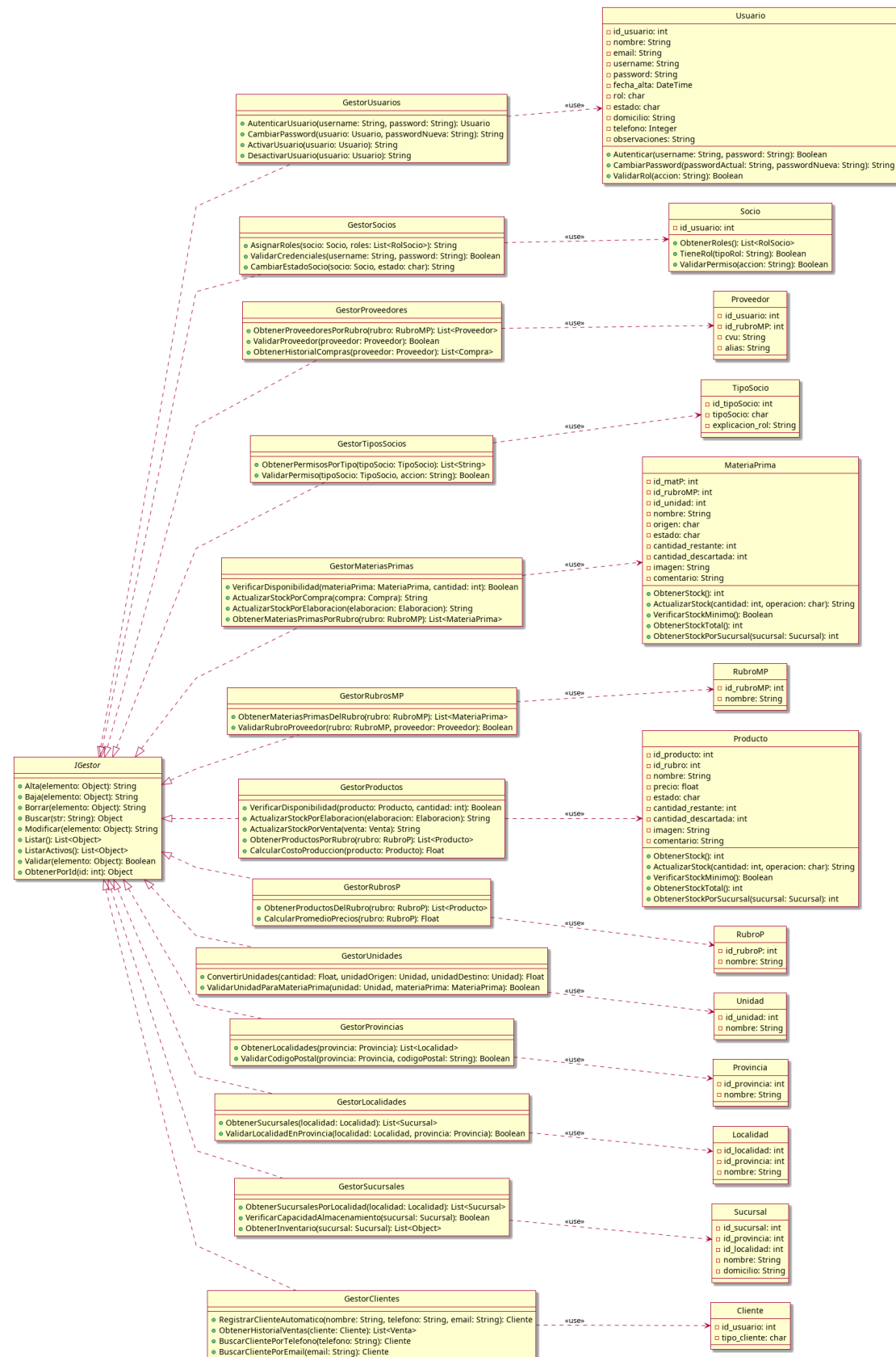
Figura 4.30: Diagrama de clases - Vista canónica
