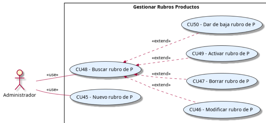
Figura 4.11: Diagrama de casos de uso para la gestión de rubros de productos
