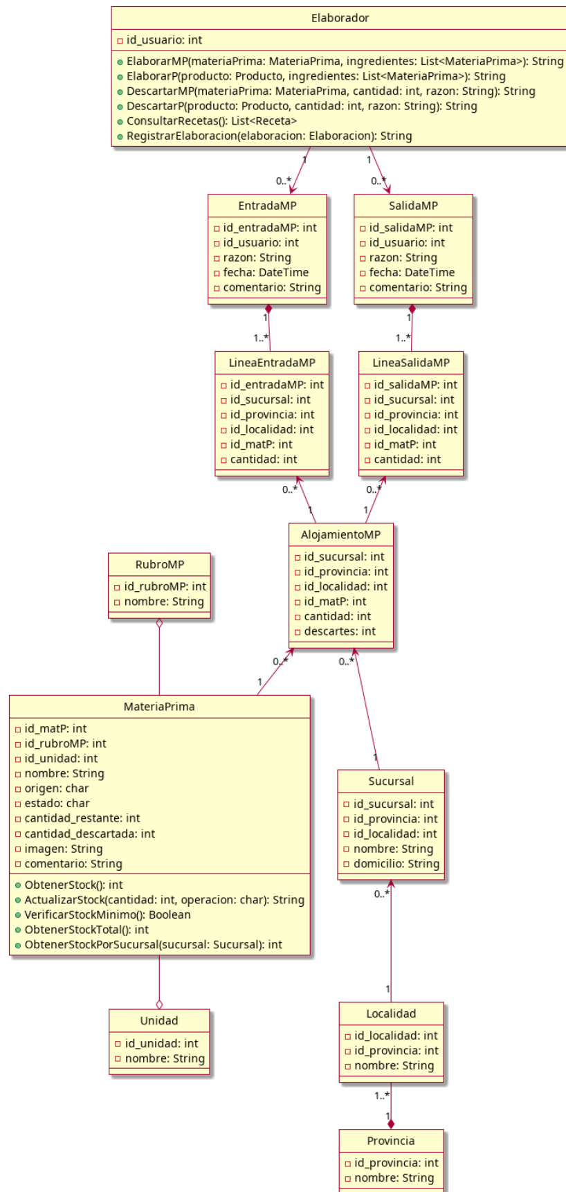
Figura 4.25: Diagrama de clases - Vista elaboración de materias primas
