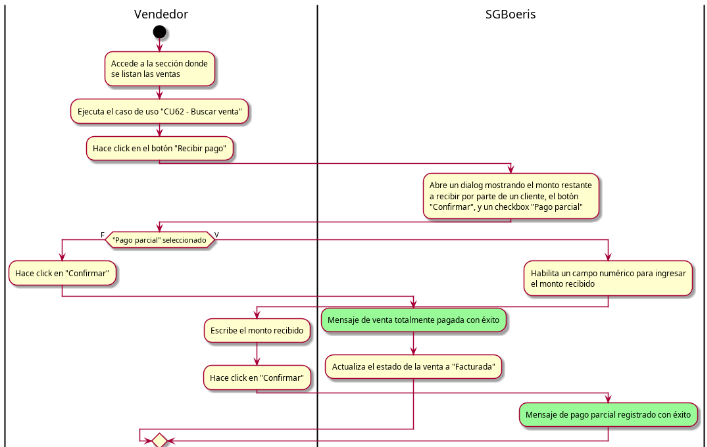
Figura 4.21: Diagrama de actividad — CU67 - Recibir pago
