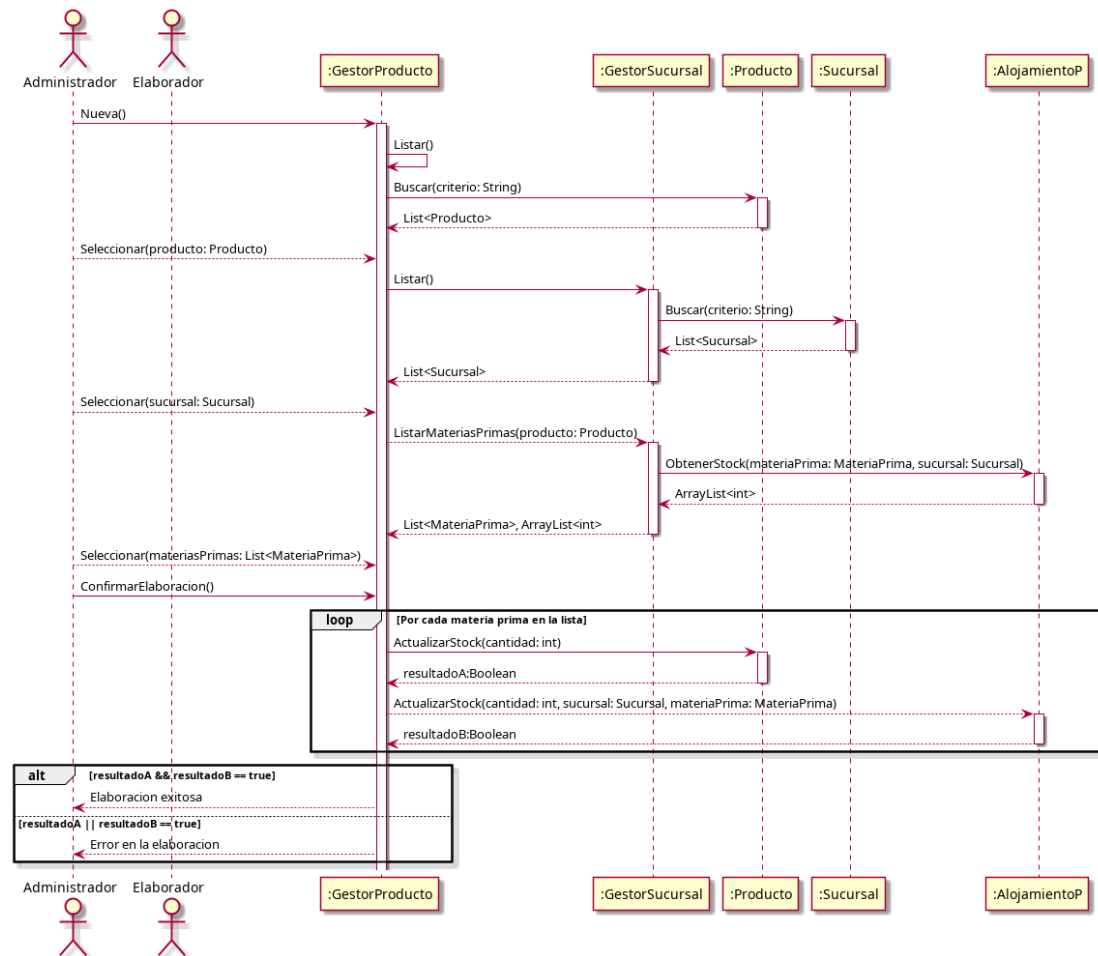
Figura 4.51: Diagrama de secuencia — CU56 - Elaborar producto
