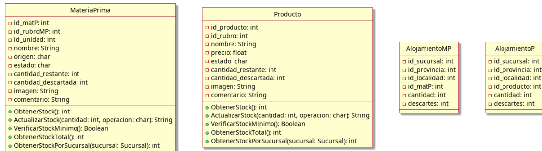
Figura 4.35: Diagrama de clases - Ficha técnica de clases (parte 5)
