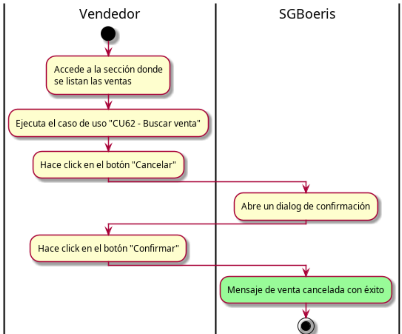
Figura 8.7: Diagrama de actividad — CU68 - Cancelar venta
