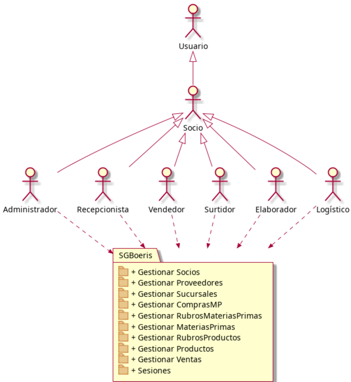
Figura 4.1: Diagrama de contexto.
