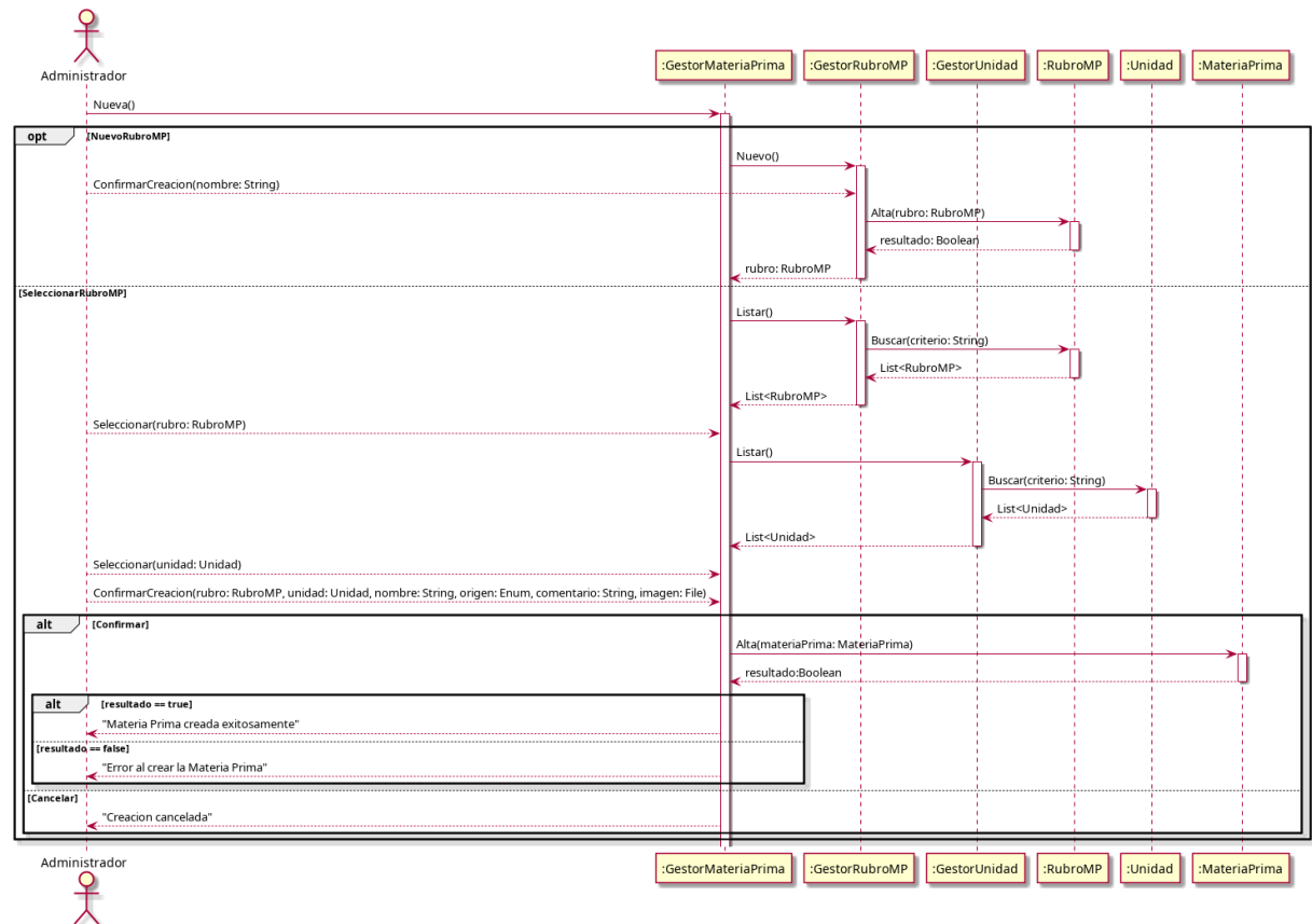
Figura 4.43: Diagrama de secuencia — CU36 - Nueva materia prima
