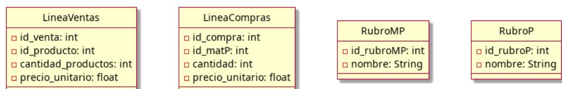
Figura 4.33: Diagrama de clases - Ficha técnica de clases (parte 3)
