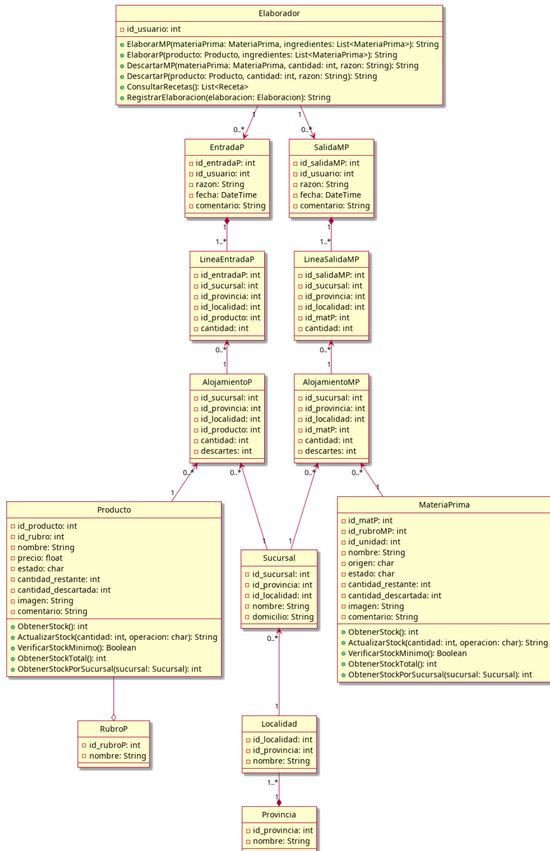
Figura 4.27: Diagrama de clases - Vista elaboración de productos
