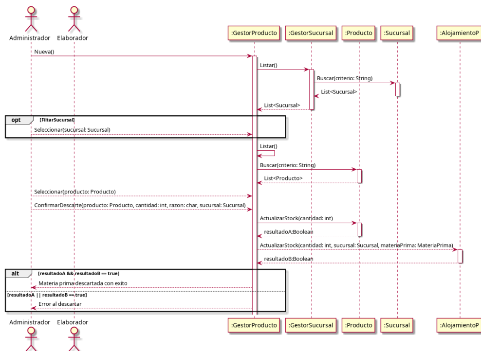
Figura 4.52: Diagrama de secuencia — CU57 - Descartar producto
