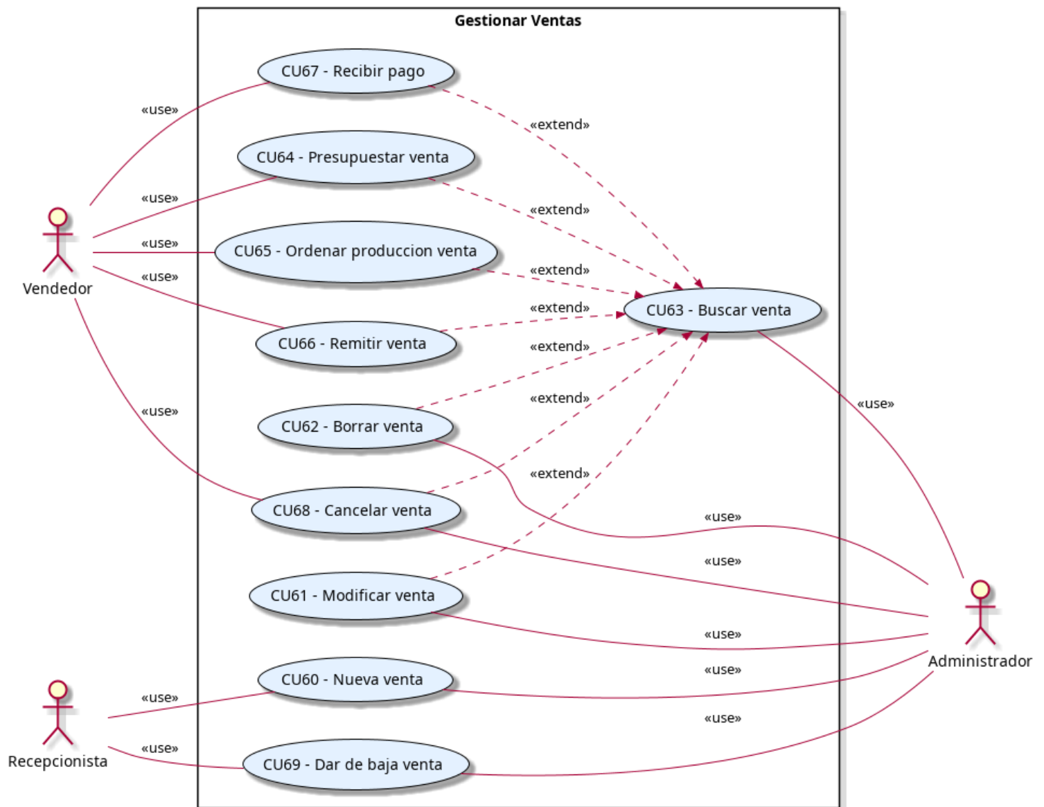
Figura 4.13: Diagrama de casos de uso para la gestión de ventas
