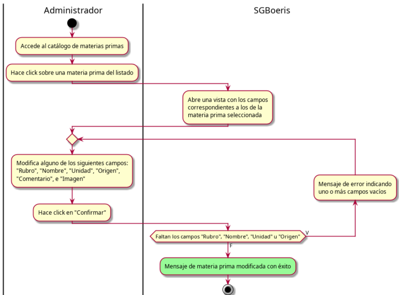
Figura 8.10: Diagrama de actividad — CU37 - Modificar materia prima
