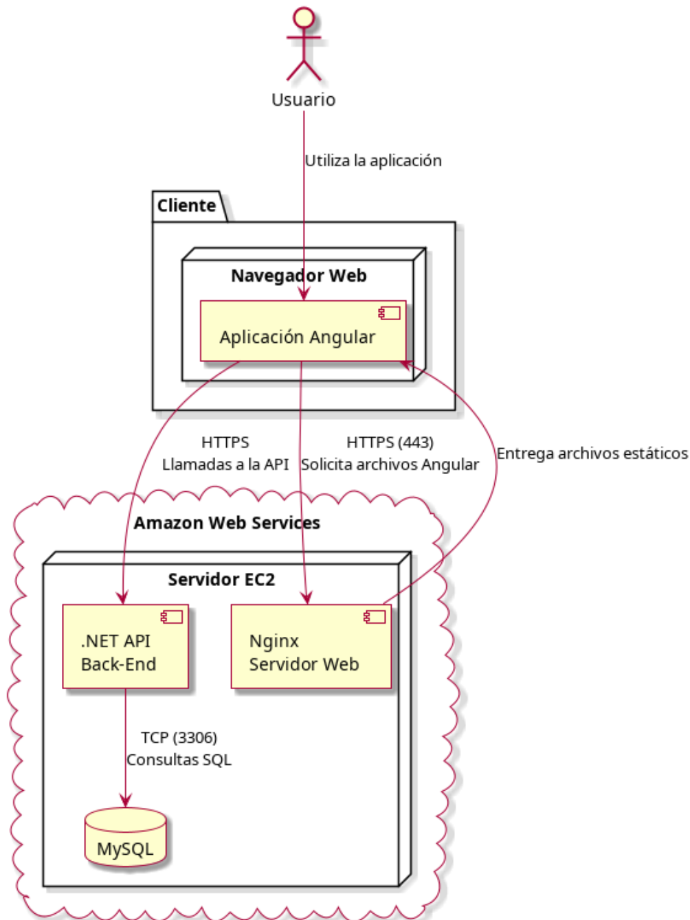
Figura 5.3: Diagrama de despliegue - Aplicación en AWS
