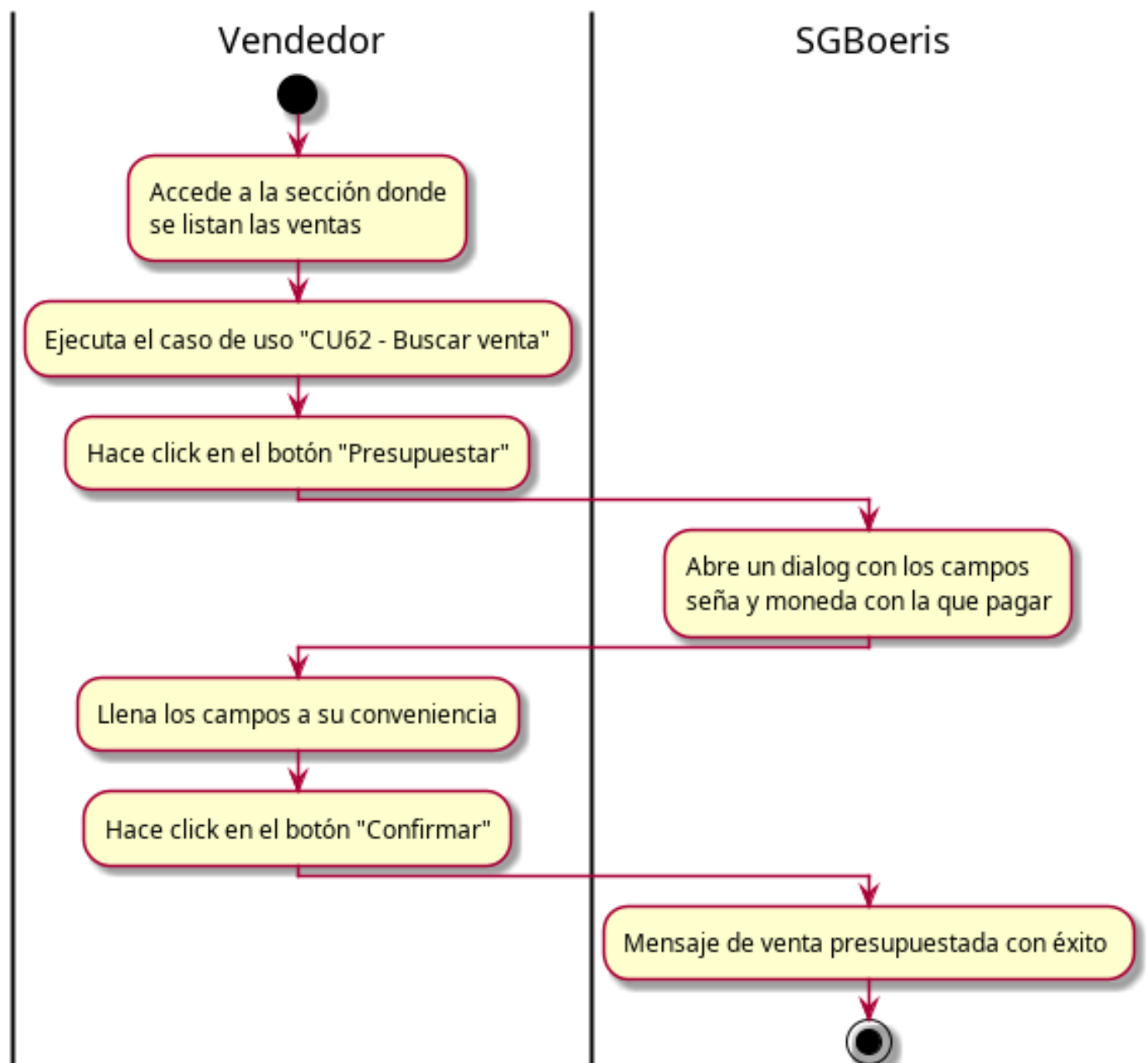
Figura 4.18: Diagrama de actividad — CU64 - Presupuestar venta
