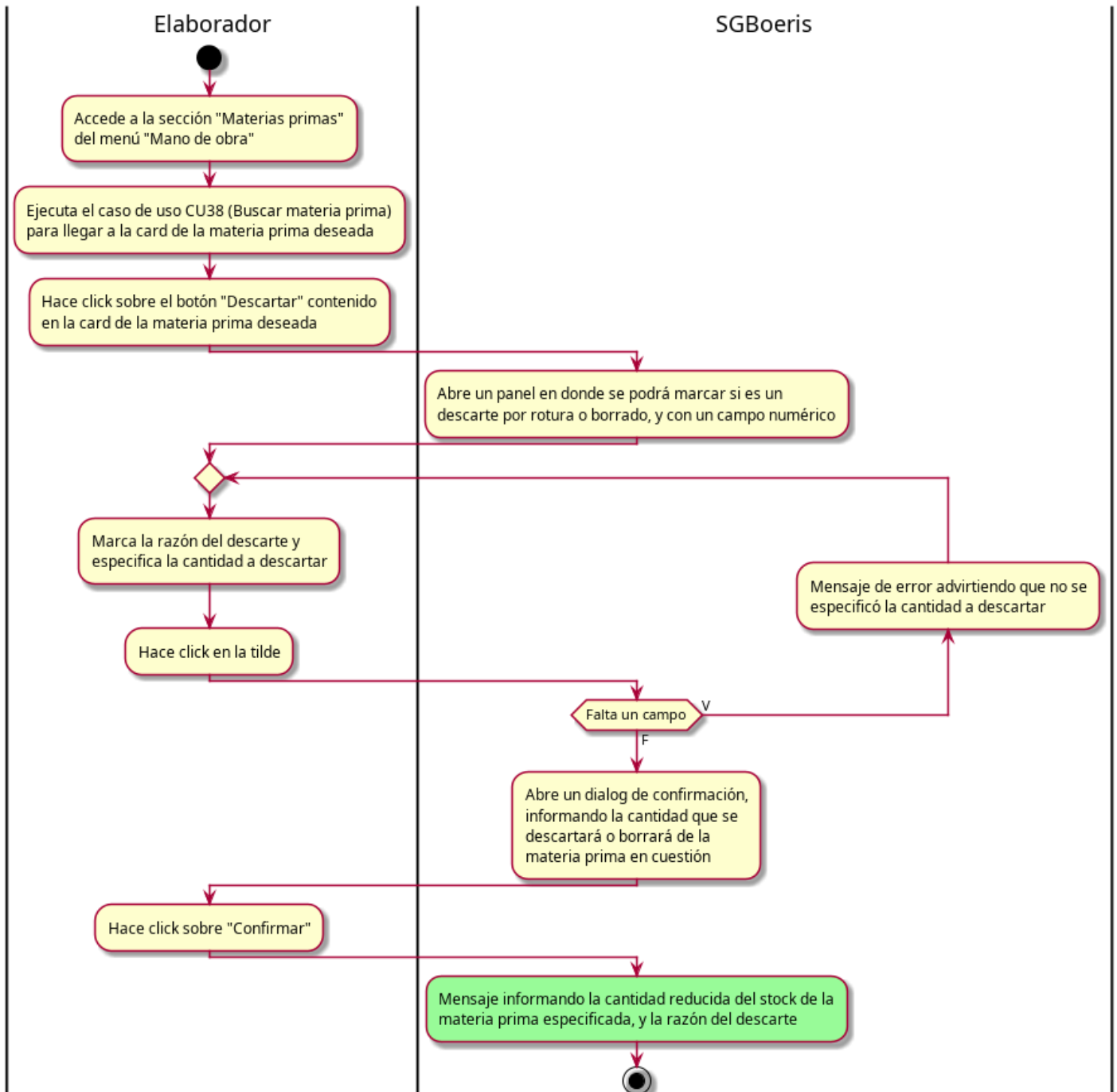
Figura 8.16: Diagrama de actividad — CU42 - Descartar materia prima
