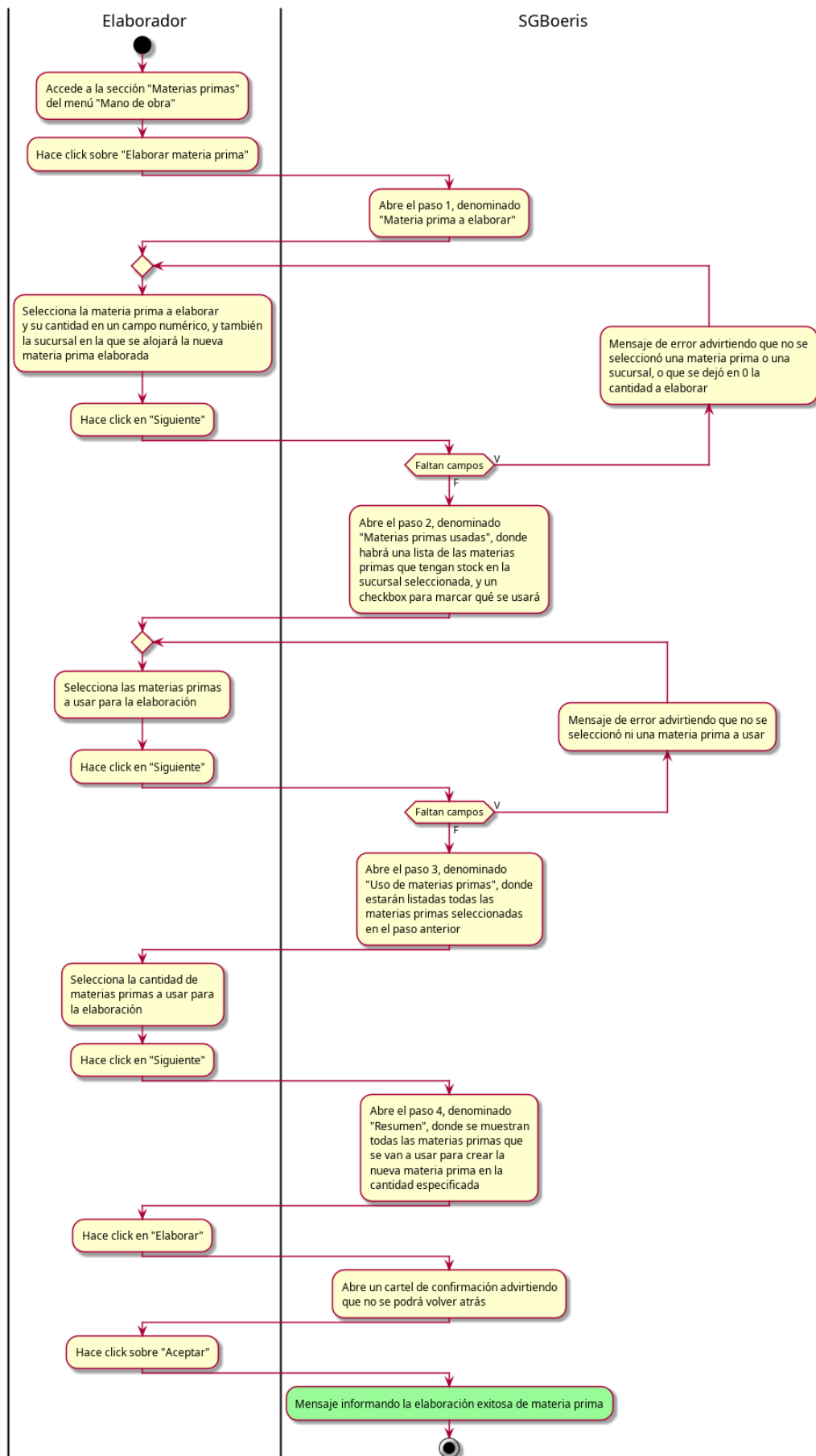
Figura 8.15: Diagrama de actividad — CU41 - Elaborar materia prima
