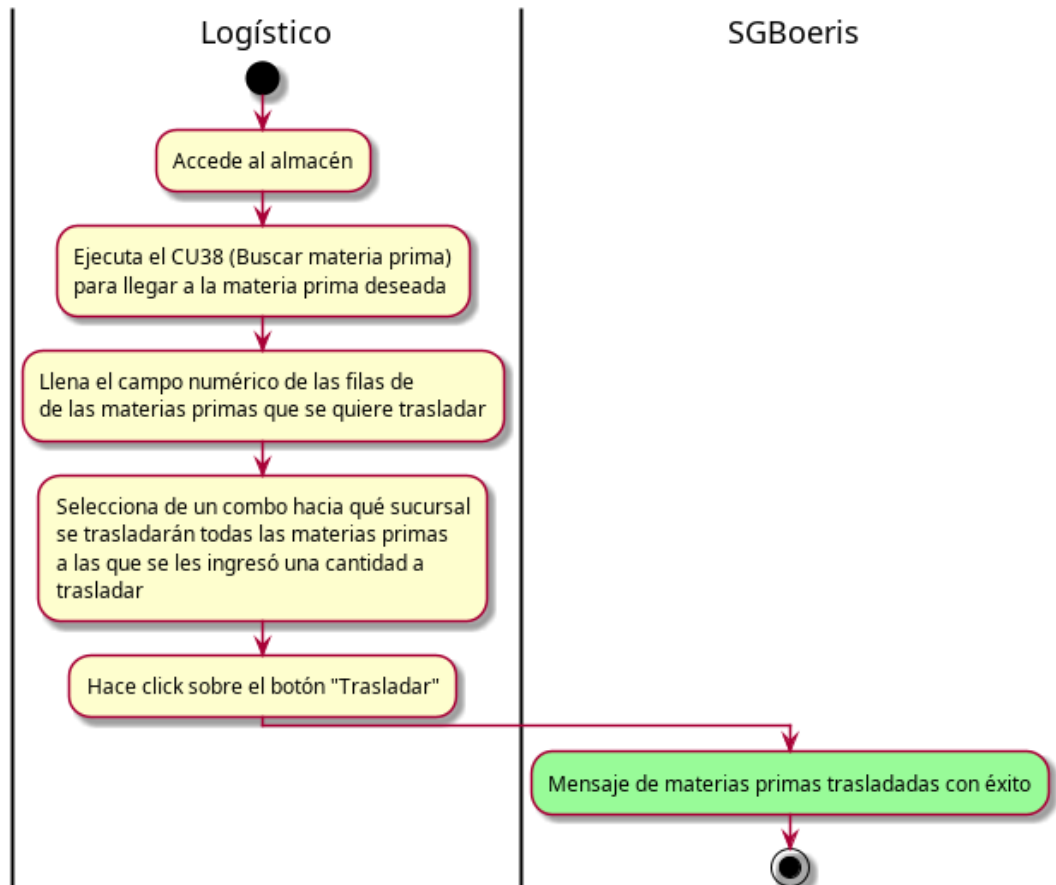
Figura 8.14: Diagrama de actividad — CU40 - Trasladar materia prima
