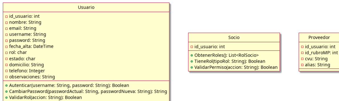
Figura 4.31: Diagrama de clases - Ficha técnica de clases (parte 1)
