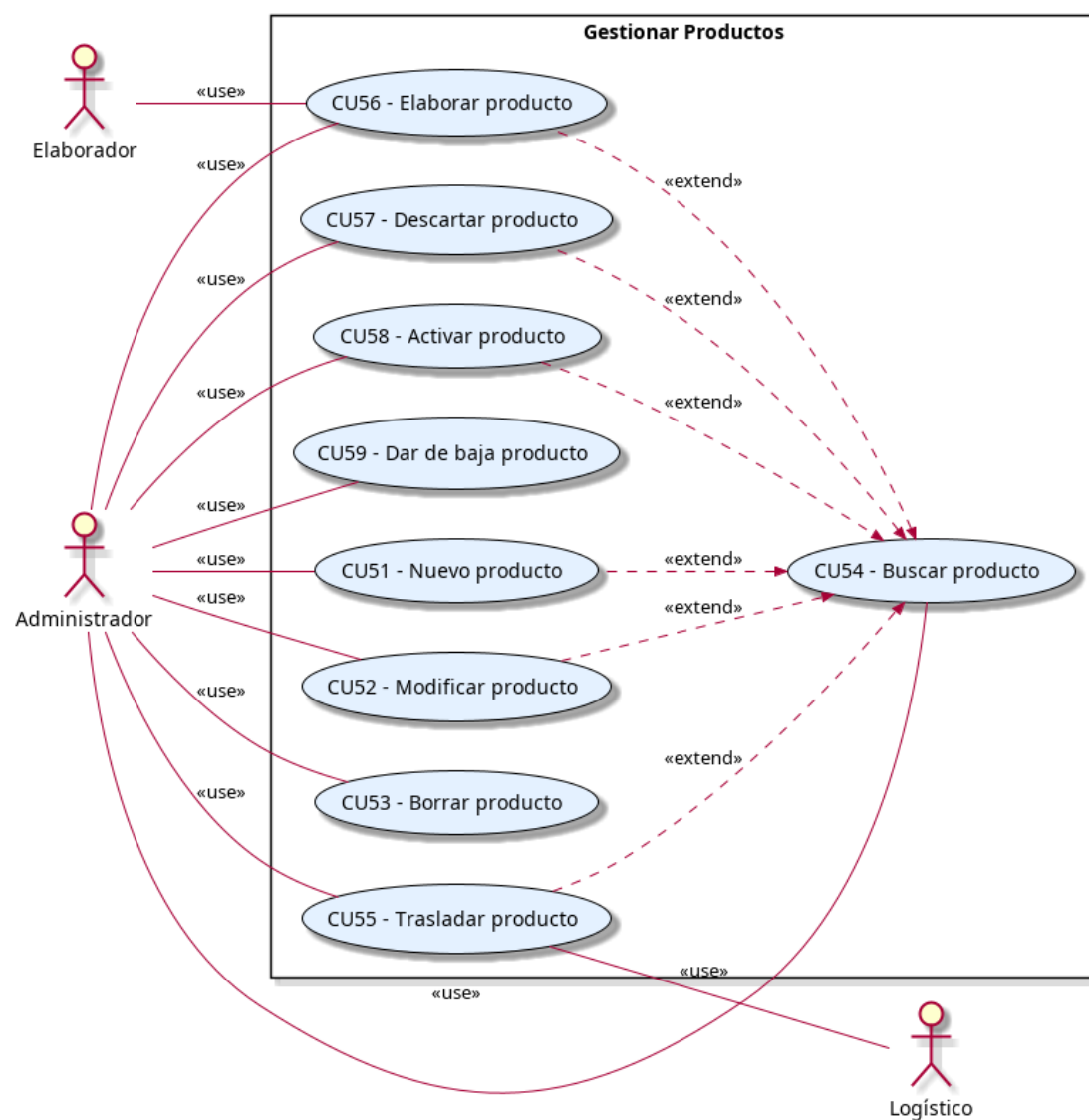
Figura 4.12: Diagrama de casos de uso para la gestión de productos
