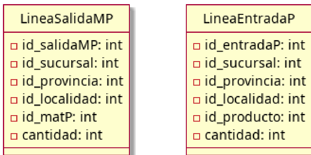
Figura 4.37: Diagrama de clases - Ficha técnica de clases (parte 7)
