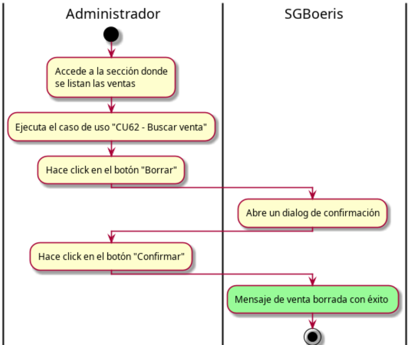
Figura 8.6: Diagrama de actividad — CU62 - Borrar venta
