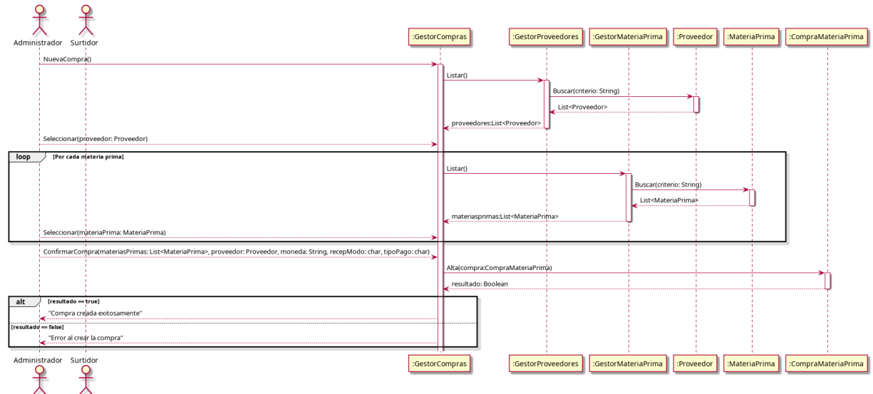
Figura 4.47: Diagrama de secuencia — CU22 - Nueva compra
