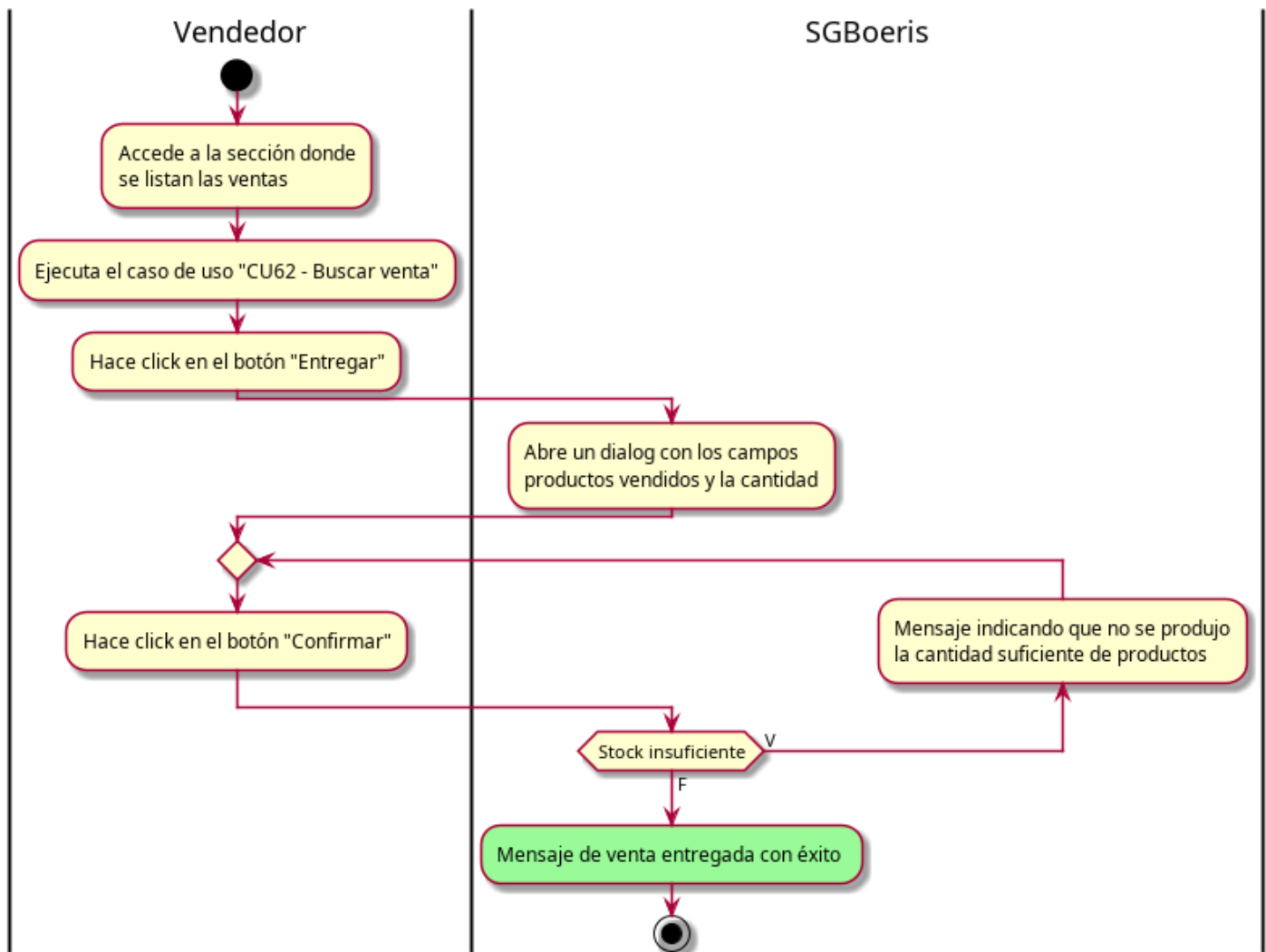
Figura 4.20: Diagrama de actividad — CU66 - Remitir venta
