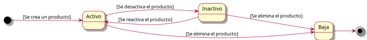
Figura 4.41: Diagrama de transición de estados - Producto
