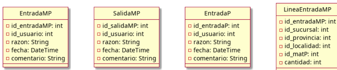
Figura 4.36: Diagrama de clases - Ficha técnica de clases (parte 6)
