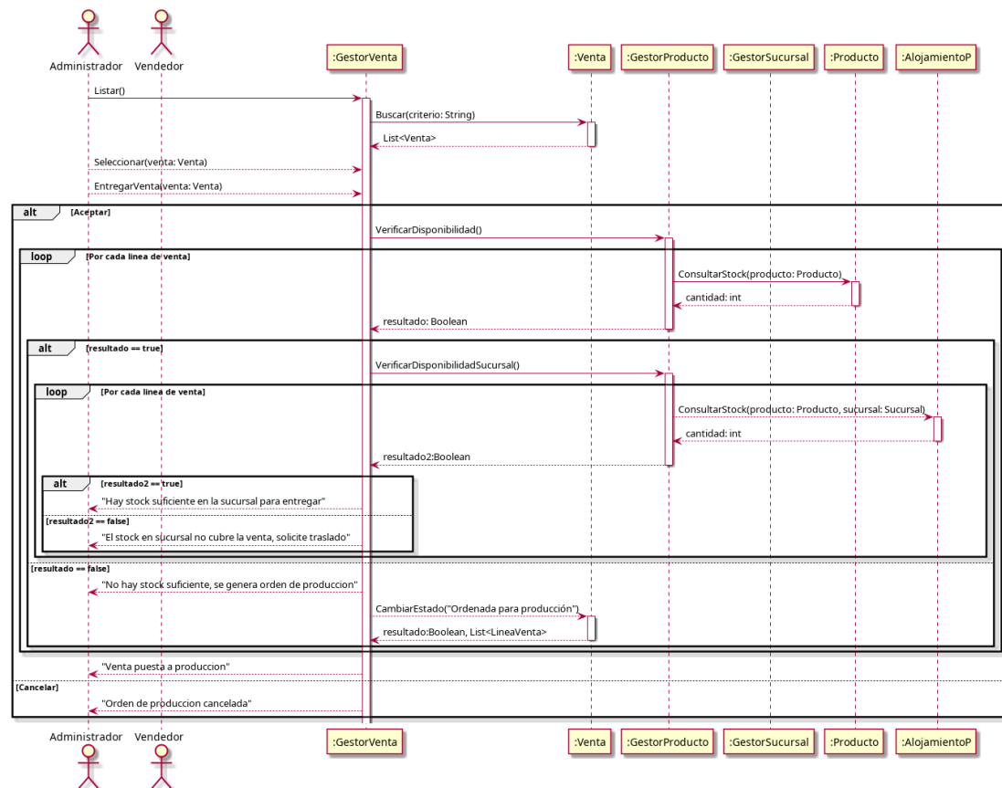
Figura 4.55: Diagrama de secuencia — CU65 - Ordenar producción venta
