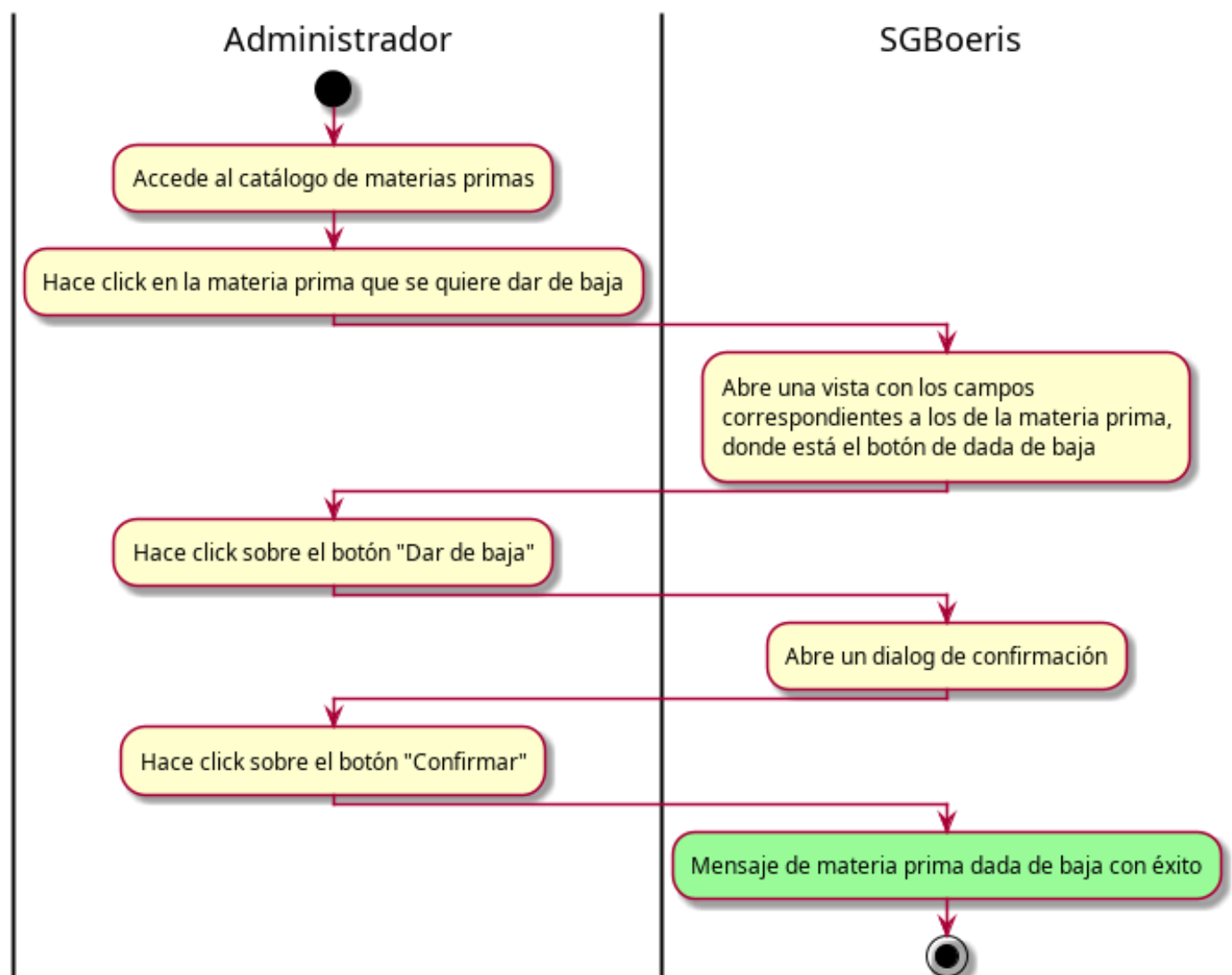
Figura 8.13: Diagrama de actividad — CU44 - Dar de baja materia prima
