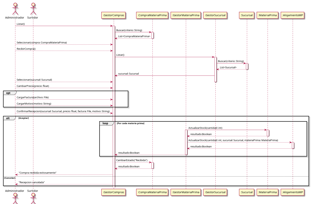
Figura 4.48: Diagrama de secuencia — CU27 - Recibir compra
