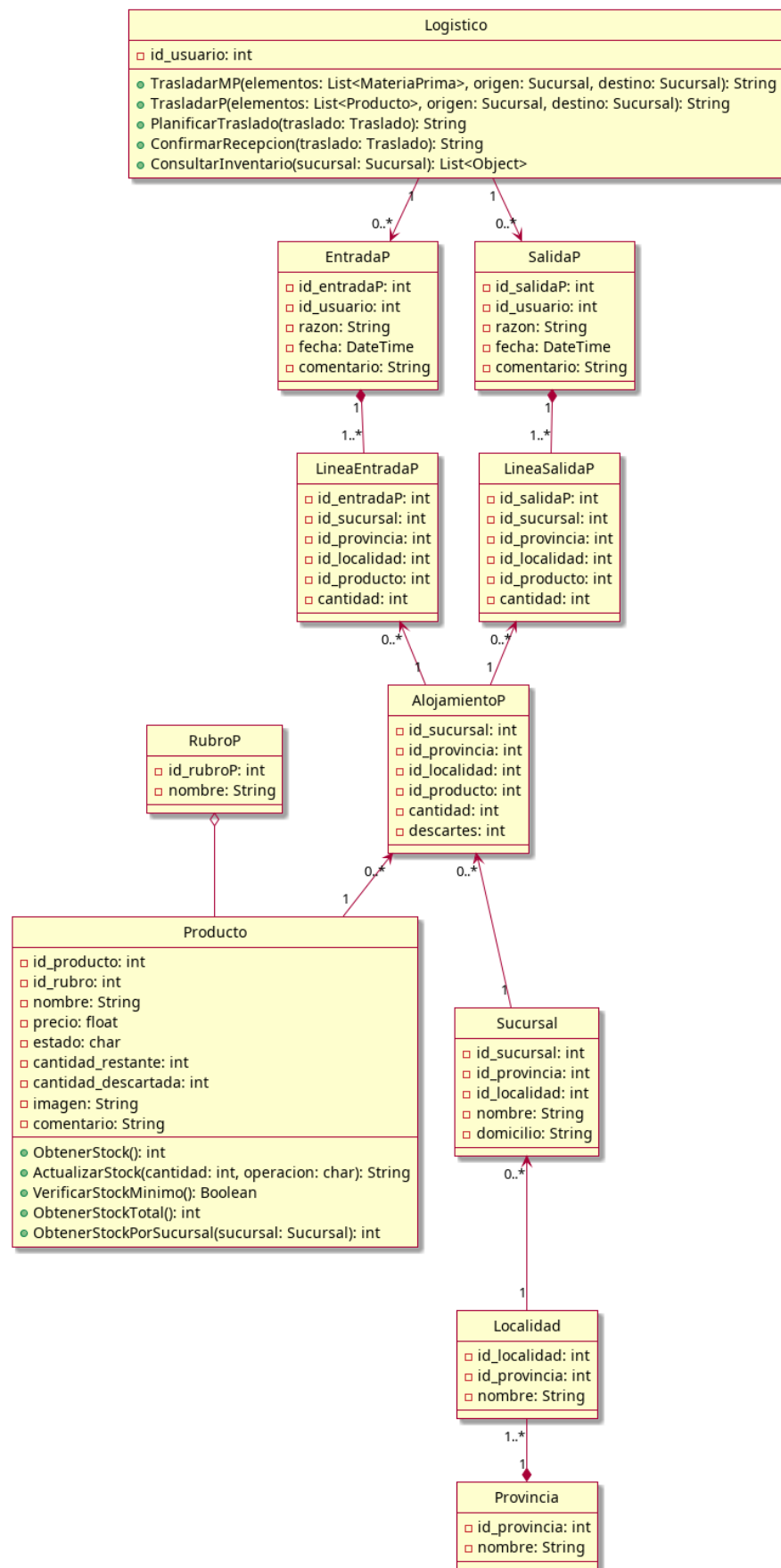
Figura 4.28: Diagrama de clases - Vista traslado de productos
