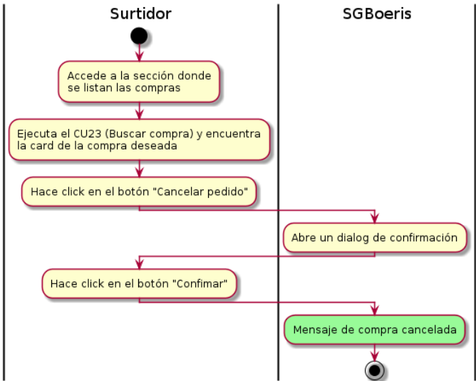
Figura 8.2: Diagrama de actividad — CU26 - Cancelar compra MP
