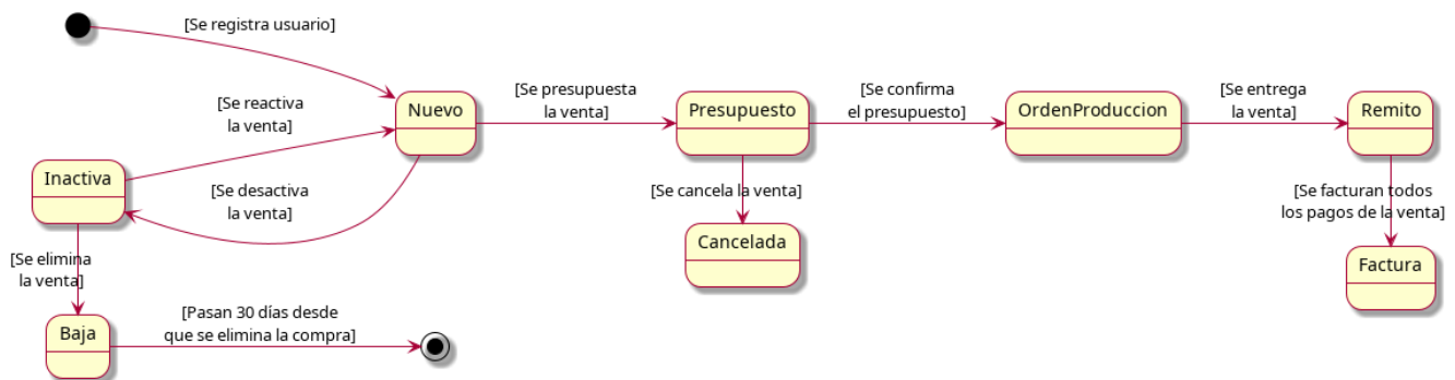
Figura 4.42: Diagrama de transición de estados - Venta
