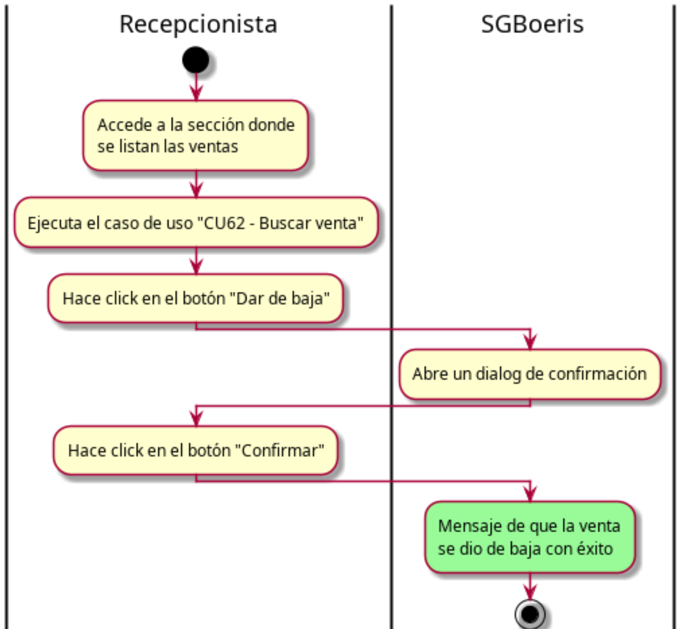
Figura 8.8: Diagrama de actividad — CU70 - Dar de baja venta
