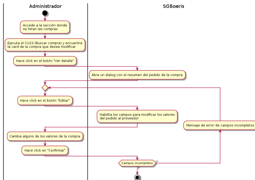
Figura 8.1: Diagrama de actividad — CU23 - Modificar compra MP
