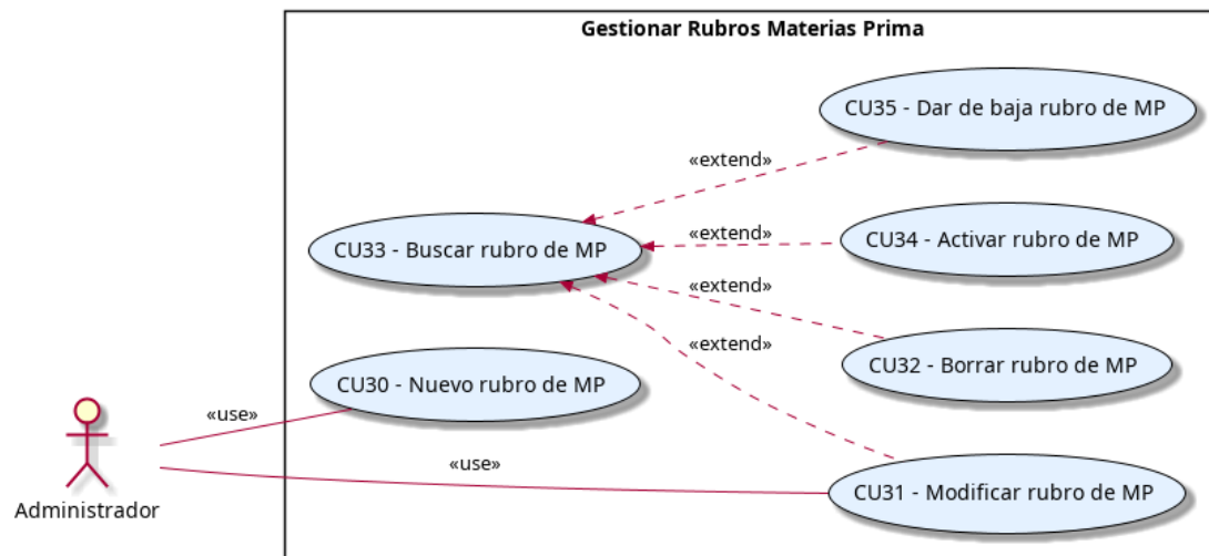
Figura 4.9: Diagrama de casos de uso para la gestión de rubros de materias primas
