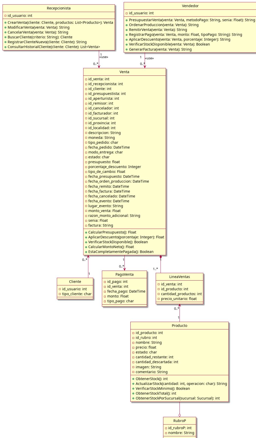
Figura 4.29: Diagrama de clases - Vista ventas
