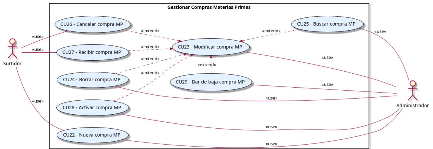
Figura 4.8: Diagrama de casos de uso para la gestión de compras de materias primas
