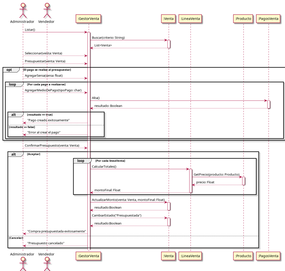
Figura 4.54: Diagrama de secuencia — CU64 - Presupuestar venta
