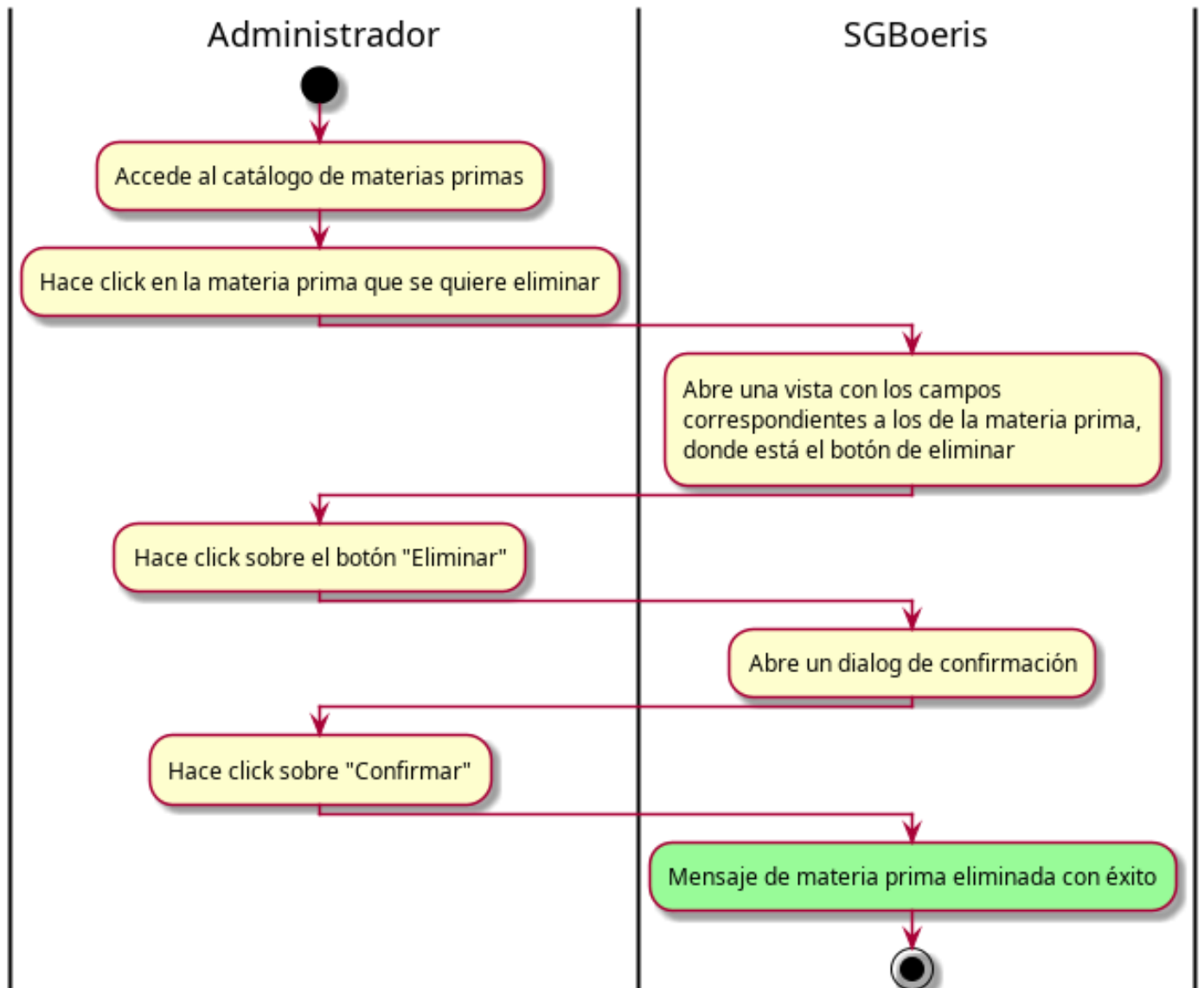
Figura 8.11: Diagrama de actividad — CU38 - Borrar materia prima
