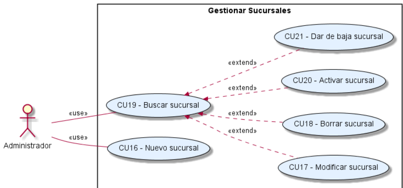
Figura 4.7: Diagrama de casos de uso para la gestión de sucursales
