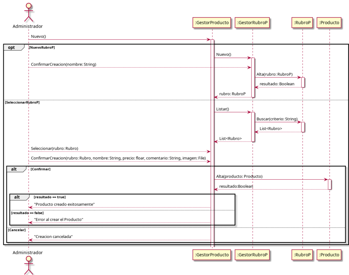
Figura 4.44: Diagrama de secuencia — CU51 - Nuevo producto
