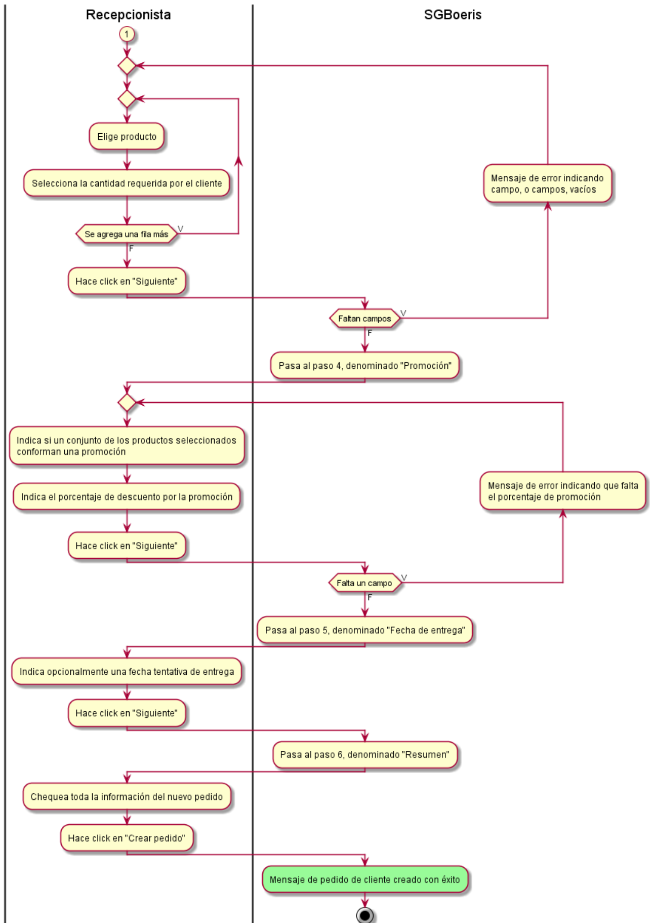
Figura 4.17: Diagrama de actividad — CU60 - Nueva venta (Parte 2)
