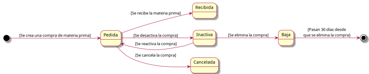
Figura 4.39: Diagrama de transición de estados - Compra
