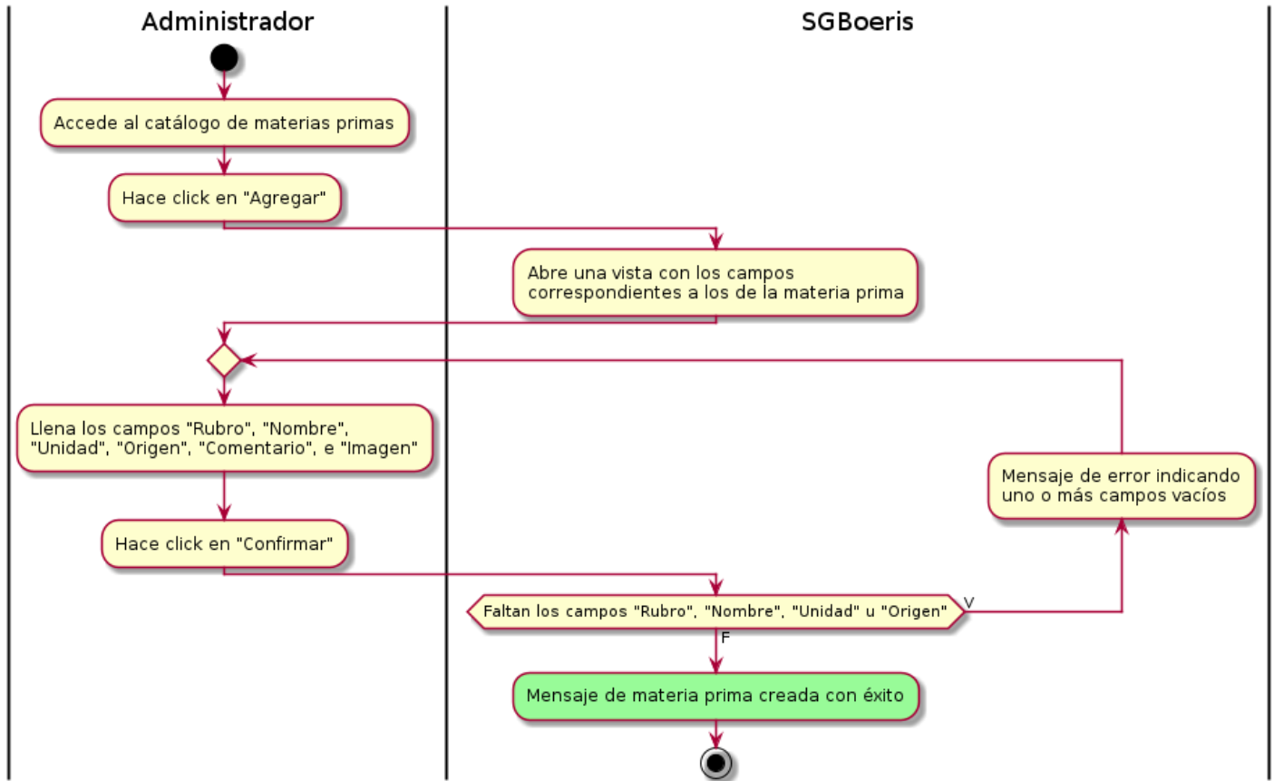
Figura 8.9: Diagrama de actividad — CU36 - Nueva materia prima
