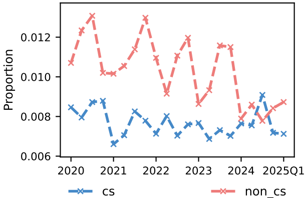
Python Variable - UPPERCASE
