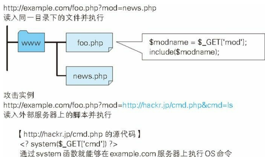
图：远程文件包含漏洞的攻击案例
