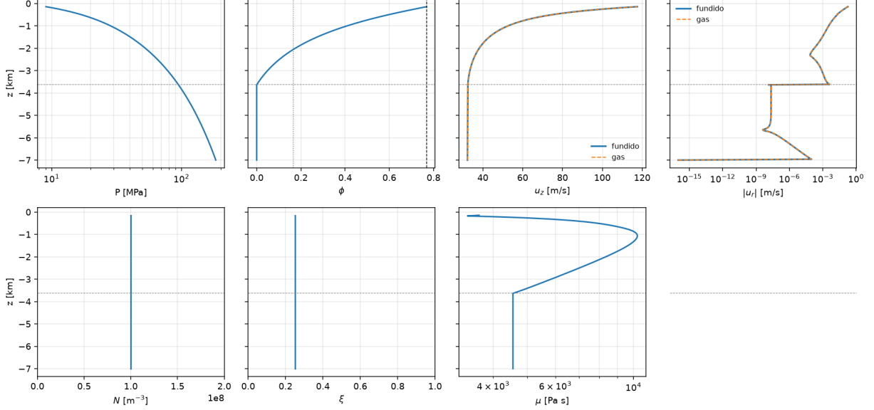
Figura 4: Columna hasta la fragmentación. La línea horizontal marca z_{\text{sat}} . P , |u_r| y \mu van en escala logarítmica. Fundido y gas coinciden porque todavía no hay deslizamiento. La marcha se detiene en \varphi_{\text{crit}} .
