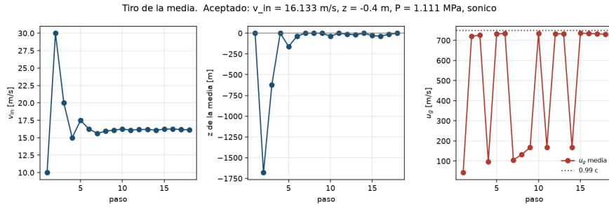
Figura 4: Tiro de \bar{u}_g . v_{\text{in}} = 16,133 m/s, boca en z = -0,44 m con P = 1,11 MPa y \bar{u}_g = 730 m/s.
