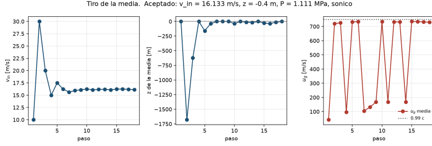
Figura 3: Tiro de \bar{u}_g . v_{in} = 16,133 m/s, boca en z = -0,44 m con P = 1,11 MPa y \bar{u}_g = 730 m/s.
