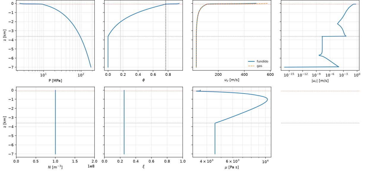
Figura 4: Entrada \bar{u} = 15,5 \text{ m/s} . La línea gris es z_{\text{sat}} y la punteada es z_f . Antes de fragmentar, fundido y gas coinciden. Después, n va sin \xi y u_g se separa. |u_r| existe solo mientras q(r) no está congelado.
