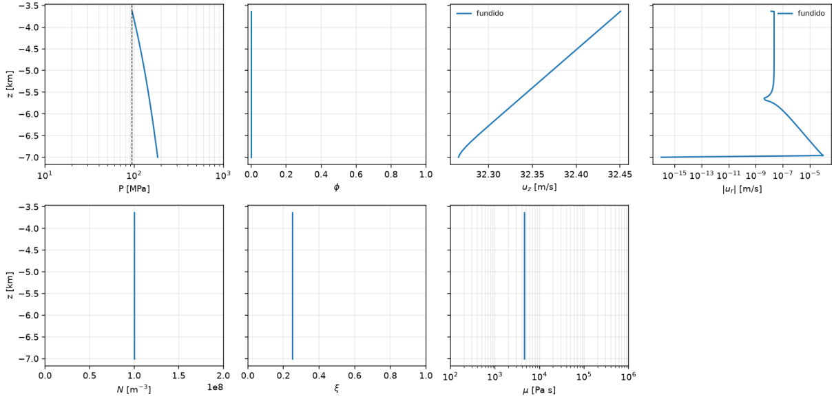
Figura 2: Tramo sin exsolución. La profundidad está en el eje vertical. P , |u_r| y \mu van en escala logarítmica horizontal. \varphi = 0 , N = 10^8 m ^{-3} y \xi = \xi_0 = 0,25 . El gas no entra: no hay curva de u_g .
