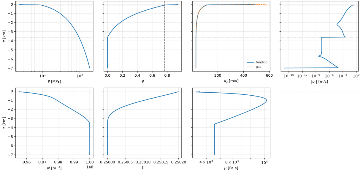
Figura 4: Entrada \bar{u} = 15,5 m/s. La línea gris es z_{\text{sat}} y la punteada es z_f . Antes de fragmentar, fundido y gas coinciden. Después, n va sin \xi y u_g se separa. |u_r| existe solo mientras q(r) no está congelado.
