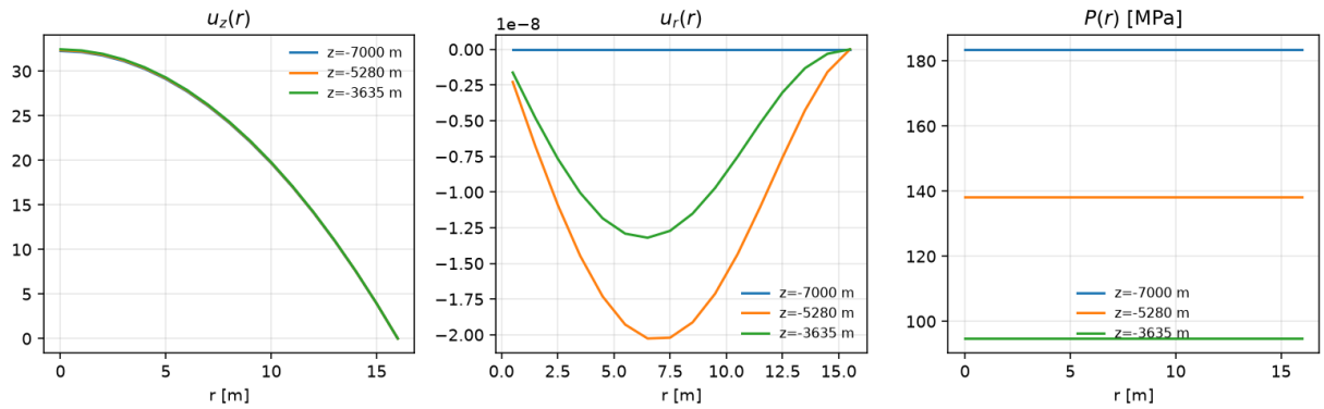
Figura 3: Perfiles en la base, a media altura y al llegar a P_{\text{sat}} . u_r queda en el ruido de la malla y P es uniforme en r .
