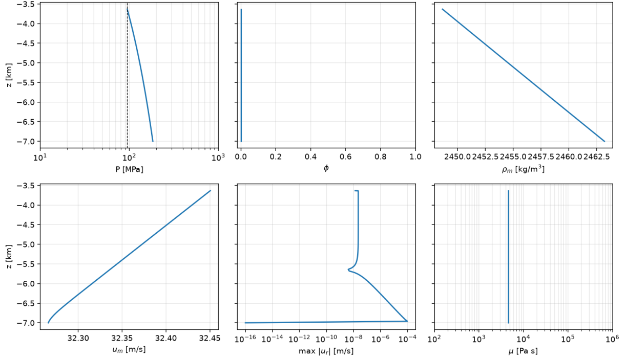
Figura 2: Tramo sin exsolución, con la profundidad en el eje vertical. P , |u_{m,r}| y \mu van en escala logarítmica horizontal. \varphi = 0 en todo el tramo: todavía no hay gas. P baja de 184 a 95 MPa y \mu queda en 4,5 \times 10^3 Pa s.
