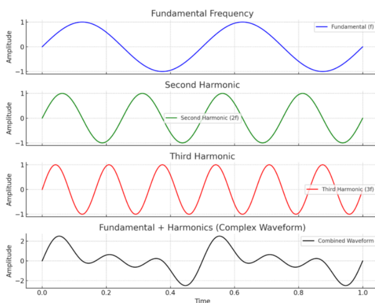
Figura 3 – Esta imagem ilustra como ondas simples se combinam para formar uma forma de onda complexa . Fonte: Yogesh Aryal(2026).
