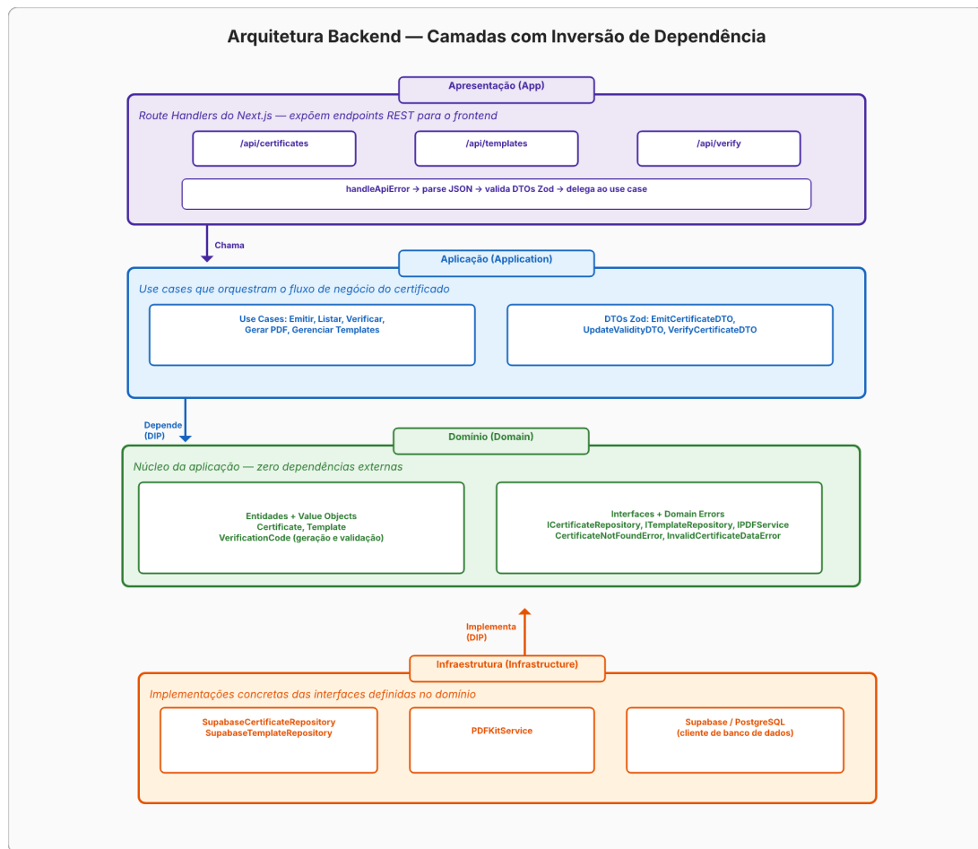
Figura 3 – Arquitetura do Backend — Quatro camadas (App, Application, Domain, Infrastructure) com DTOs, Value Objects e fluxo de dependências
