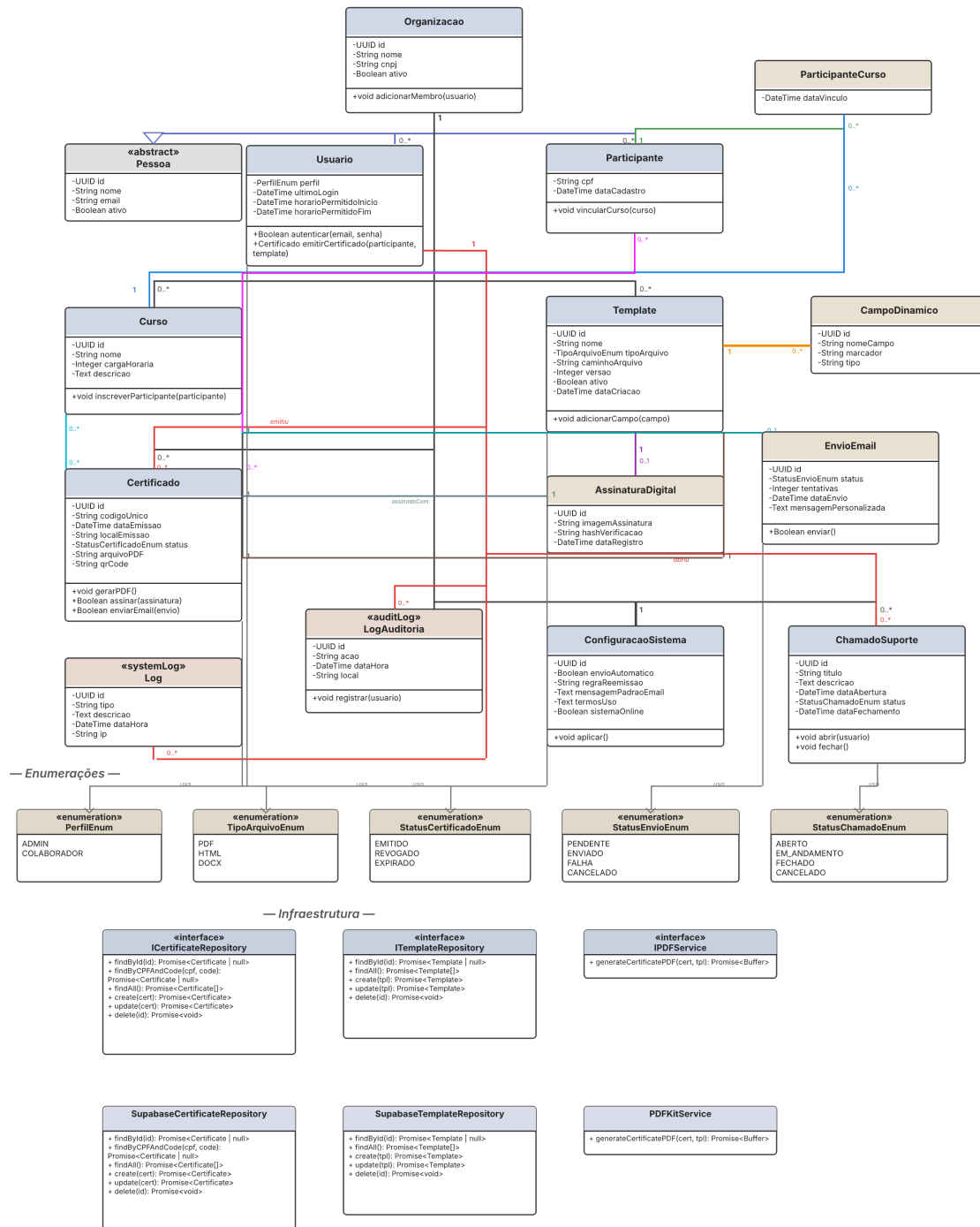
Diagrama de Classes — Sistema de Certificados — Domínio —
