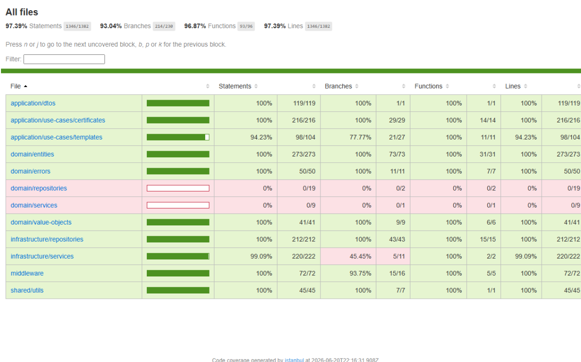
Figura 19 – Relatório de cobertura dos testes — backend
