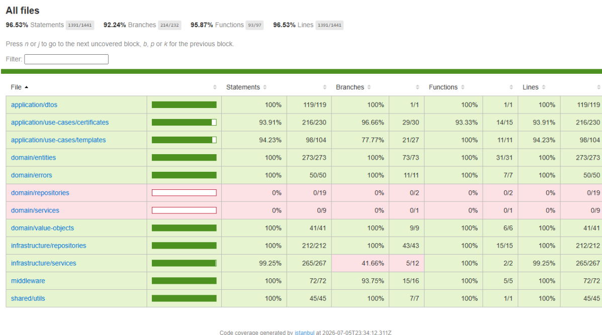
Figura 19 – Relatório de cobertura dos testes — backend
