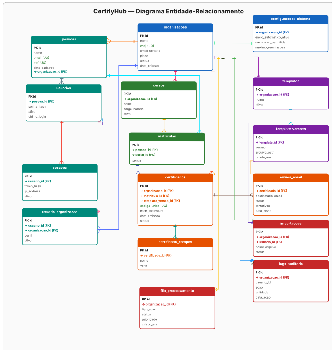
Figura 5 – Diagrama Entidade-Relacionamento (DER) do Banco de Dados
