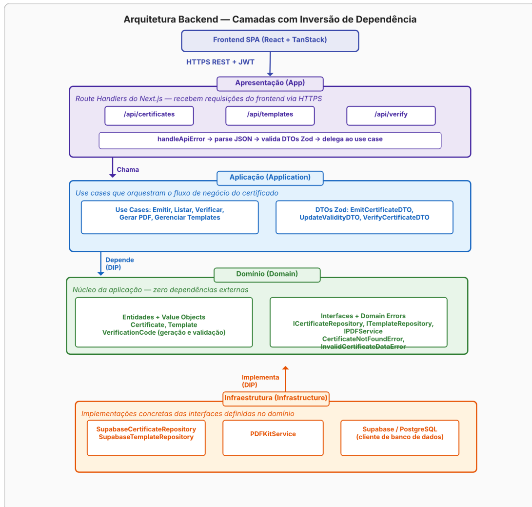
Figura 3 – Arquitetura do Backend — Quatro camadas (App, Application, Domain, Infraestrutura) com DTOs, Value Objects e fluxo de dependências
