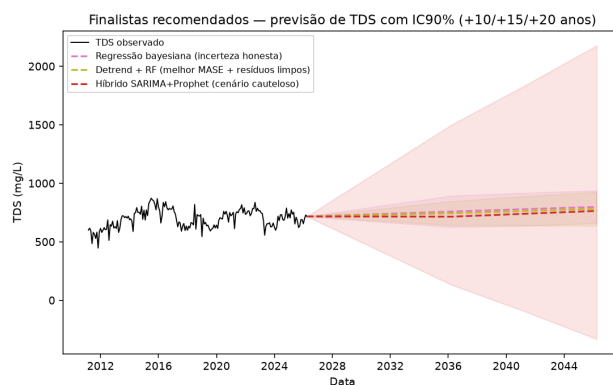
Figure 23: Finalistas recomendados – regressão bayesiana, Detrend+RF e híbrido SARIMA+Prophet – com IC90% para +10/+15/+20 anos.
