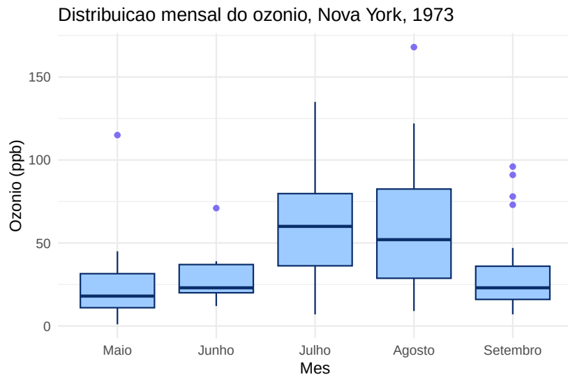
Figure 1: Distribuição do ozônio em cada mês.
