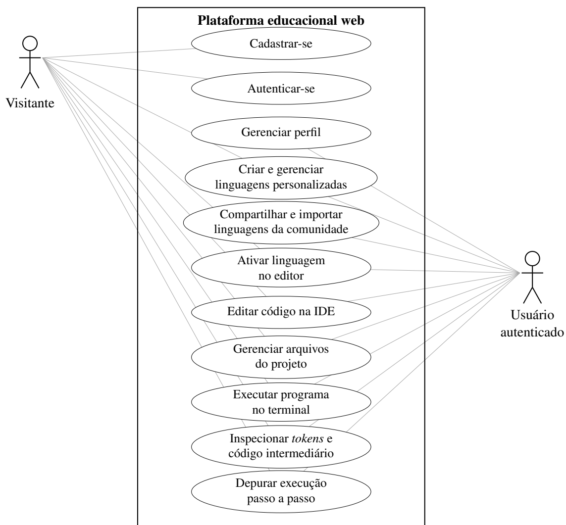
Figura 3.1 – Casos de uso: acesso e ambiente de desenvolvimento.
