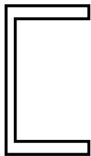
Pos. 6 Kufe: U 80 - 690 (2 Stk.) Walzprofil U80 DIN 1026 — Zukaufteil, kein Blechzuschnitt
