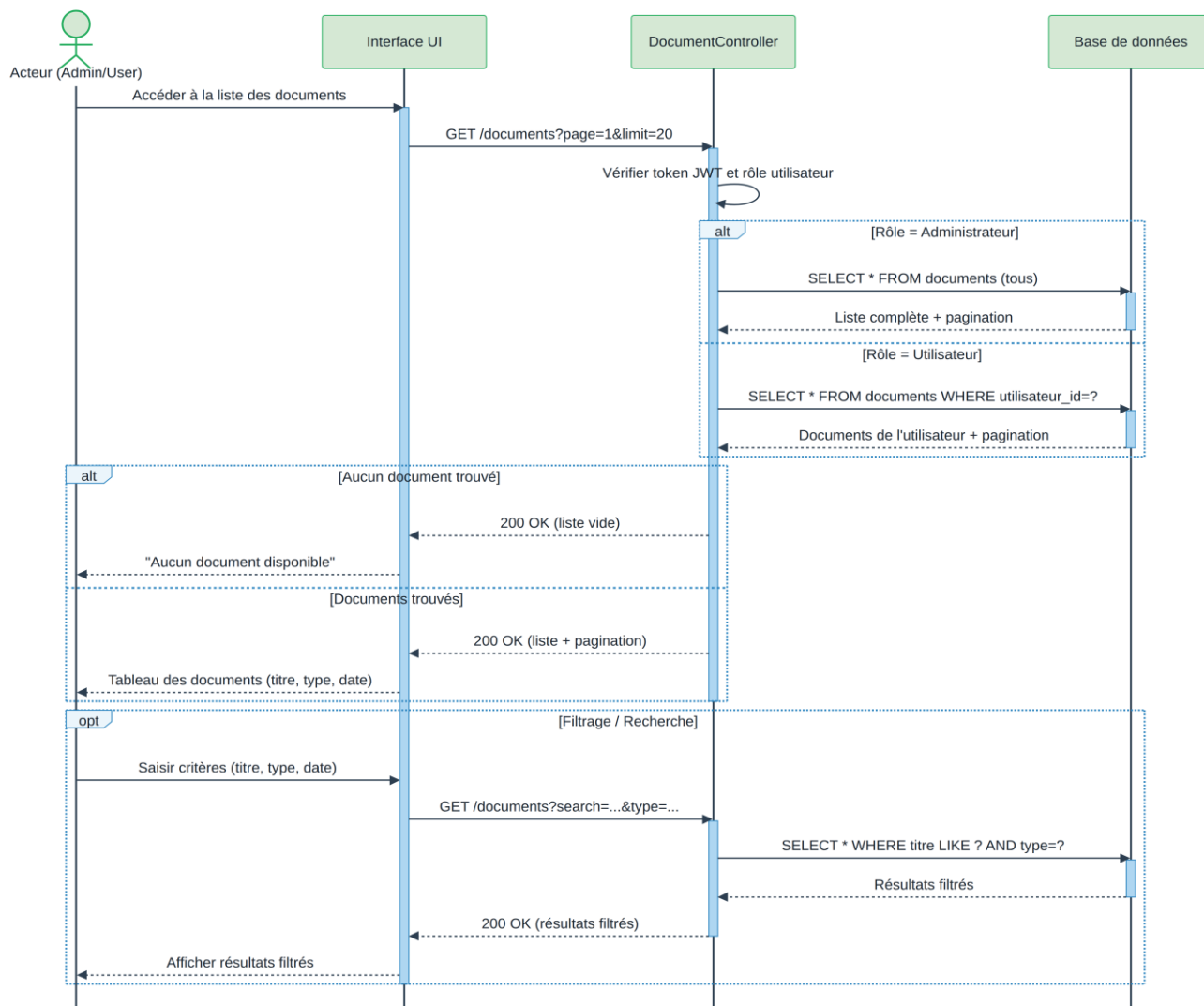
Figure 10: Diagramme de séquence Consulter les documents
