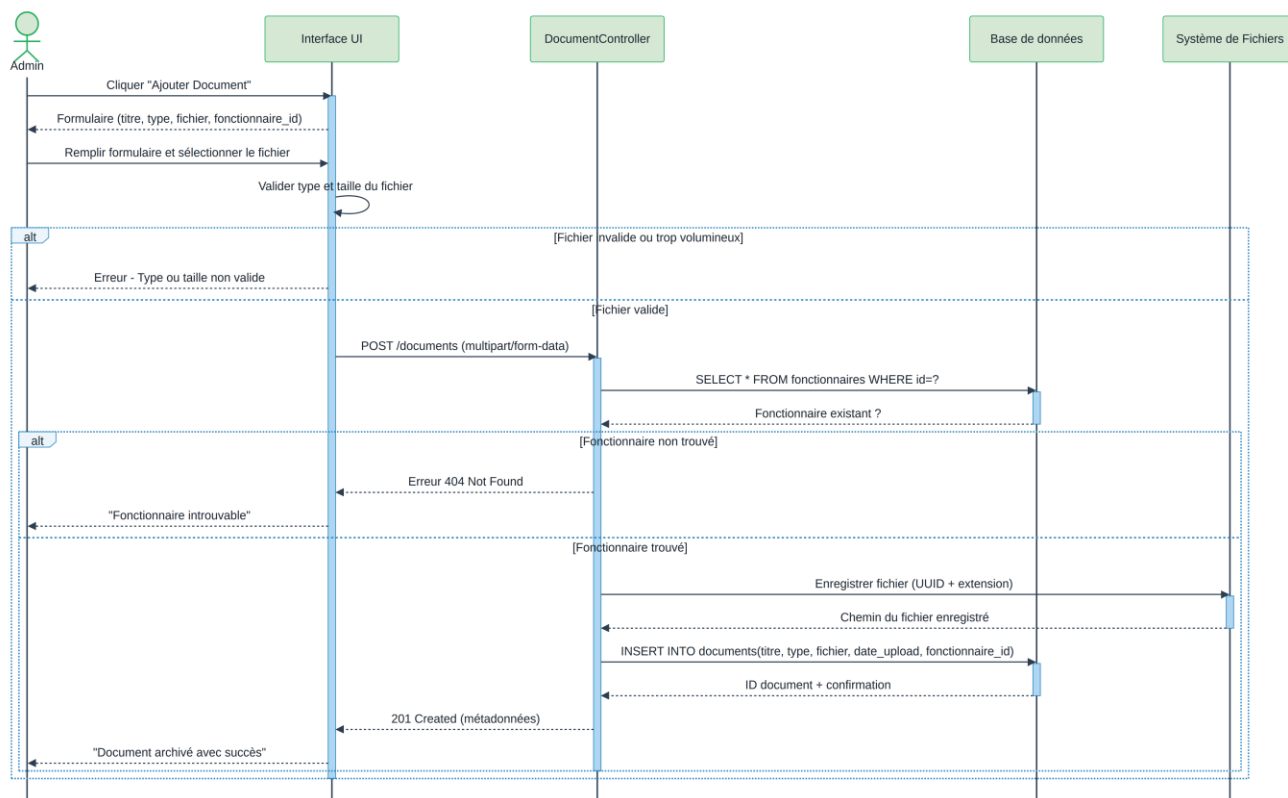
Figure 9: Diagramme de séquence Archiver un document
