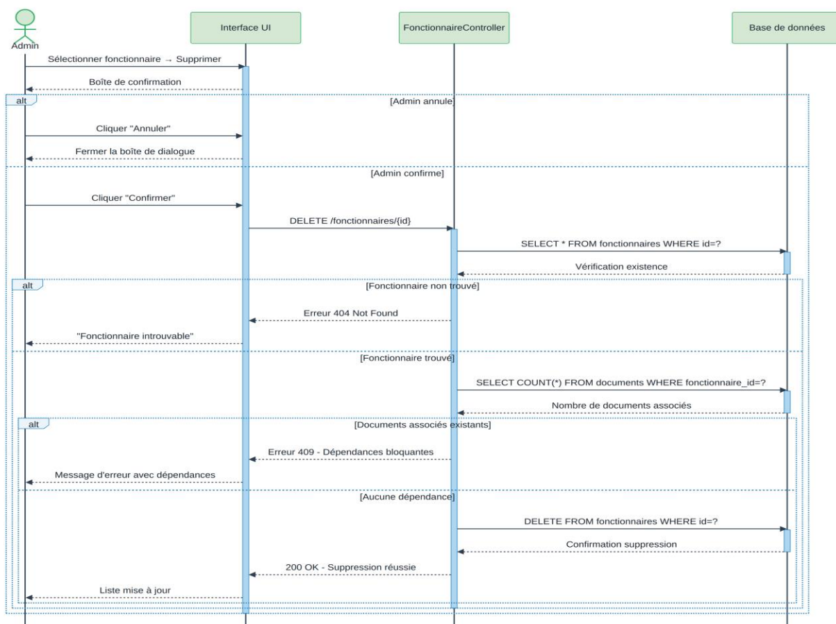
Figure 8: Diagramme de séquence Supprimer un fonctionnaire
