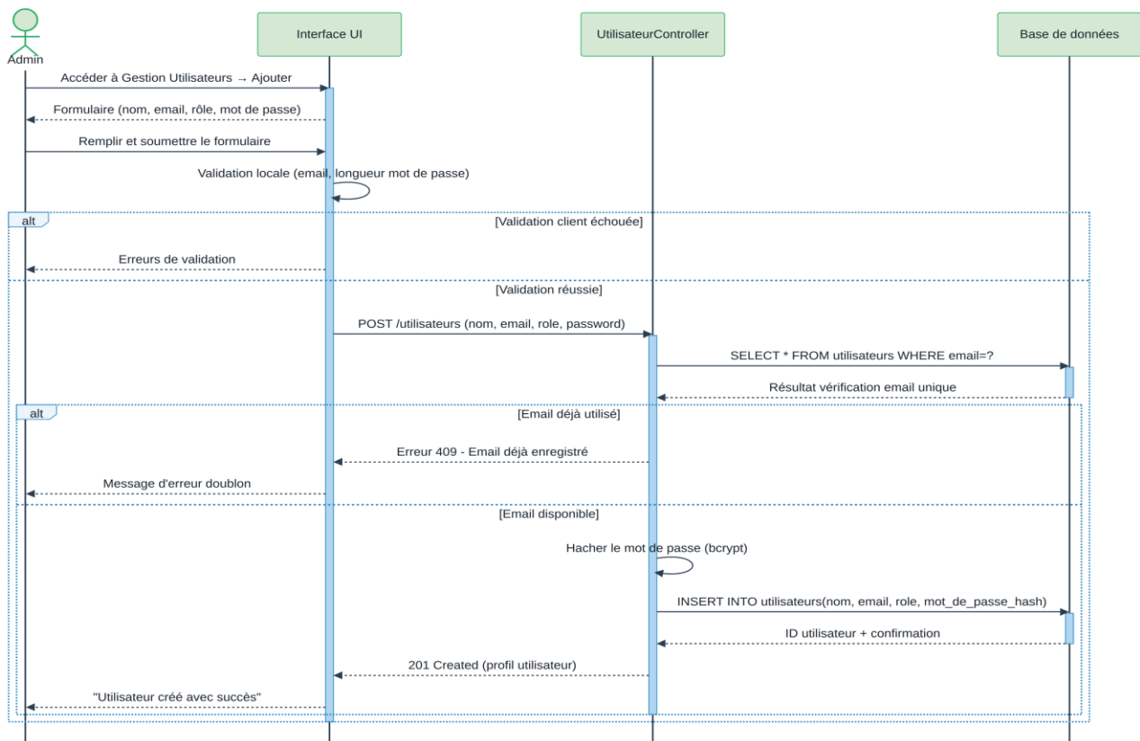
Figure 12: Diagramme de séquence Ajouter un utilisateur
