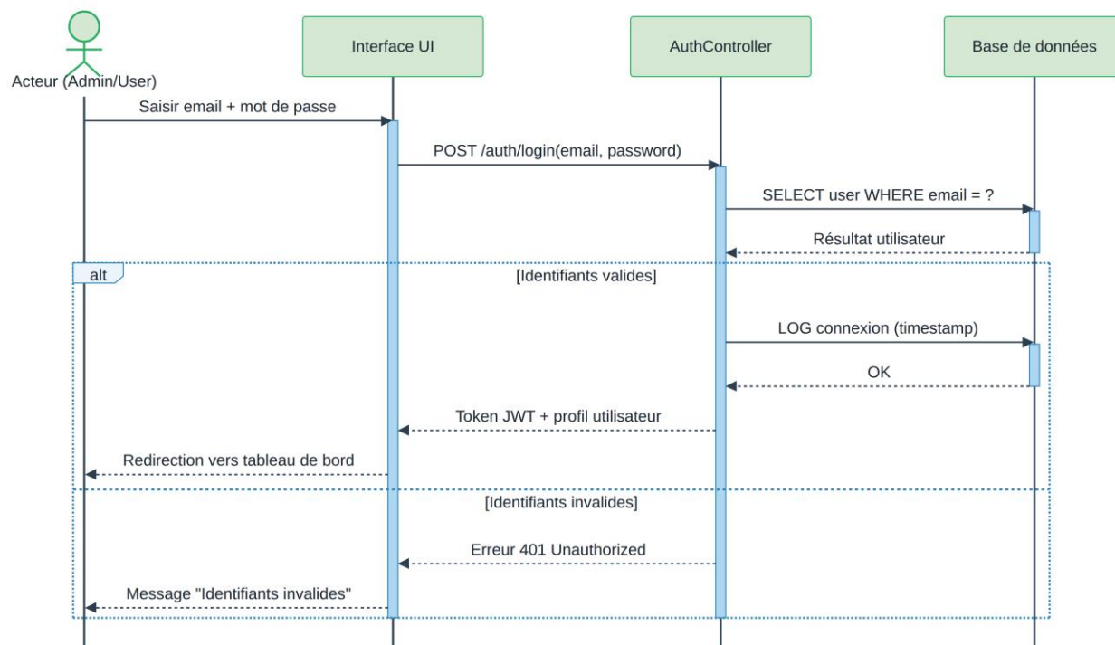
Figure 5: Diagramme de séquence de login
