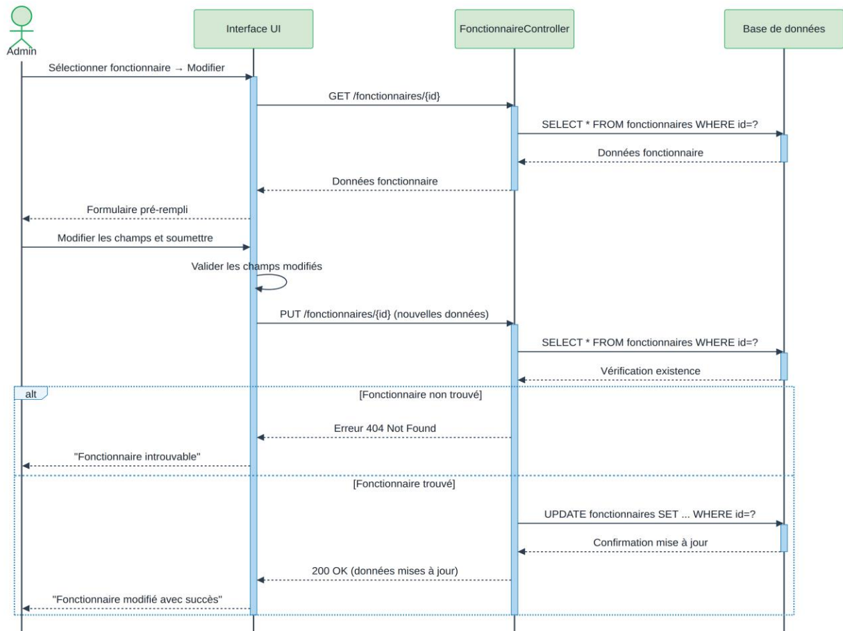
Figure 7: Diagramme de séquence Modifier un fonctionnaire
