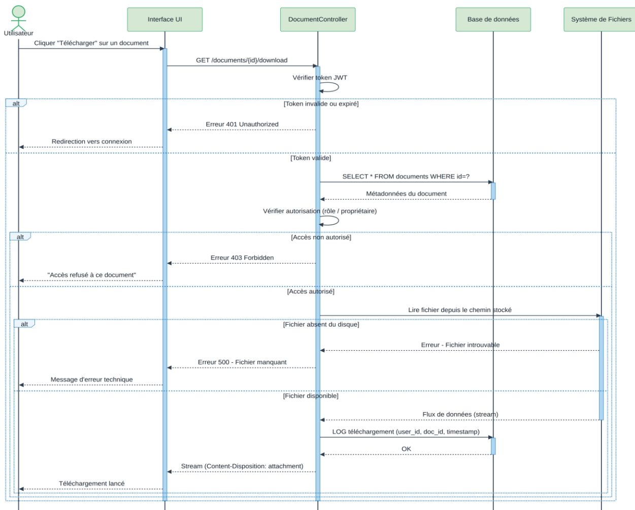
Figure 11: Diagramme de séquence Télécharger un document
