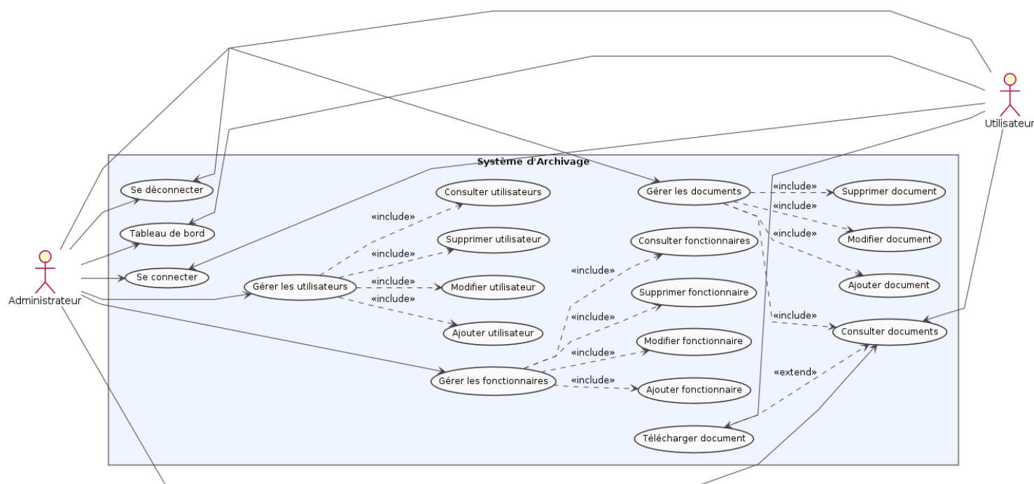
Figure 4: Diagramme de cas d'utilisation
