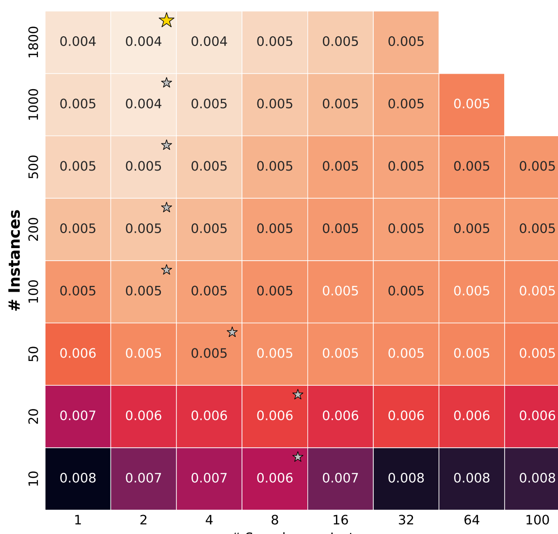
Wasserstein
