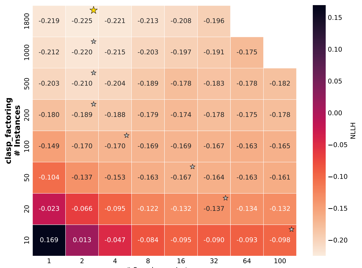
NLLH
