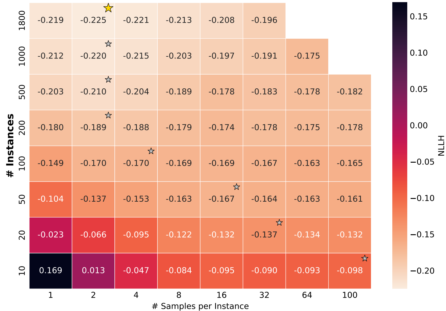
clasp_factoring (NLLH)
