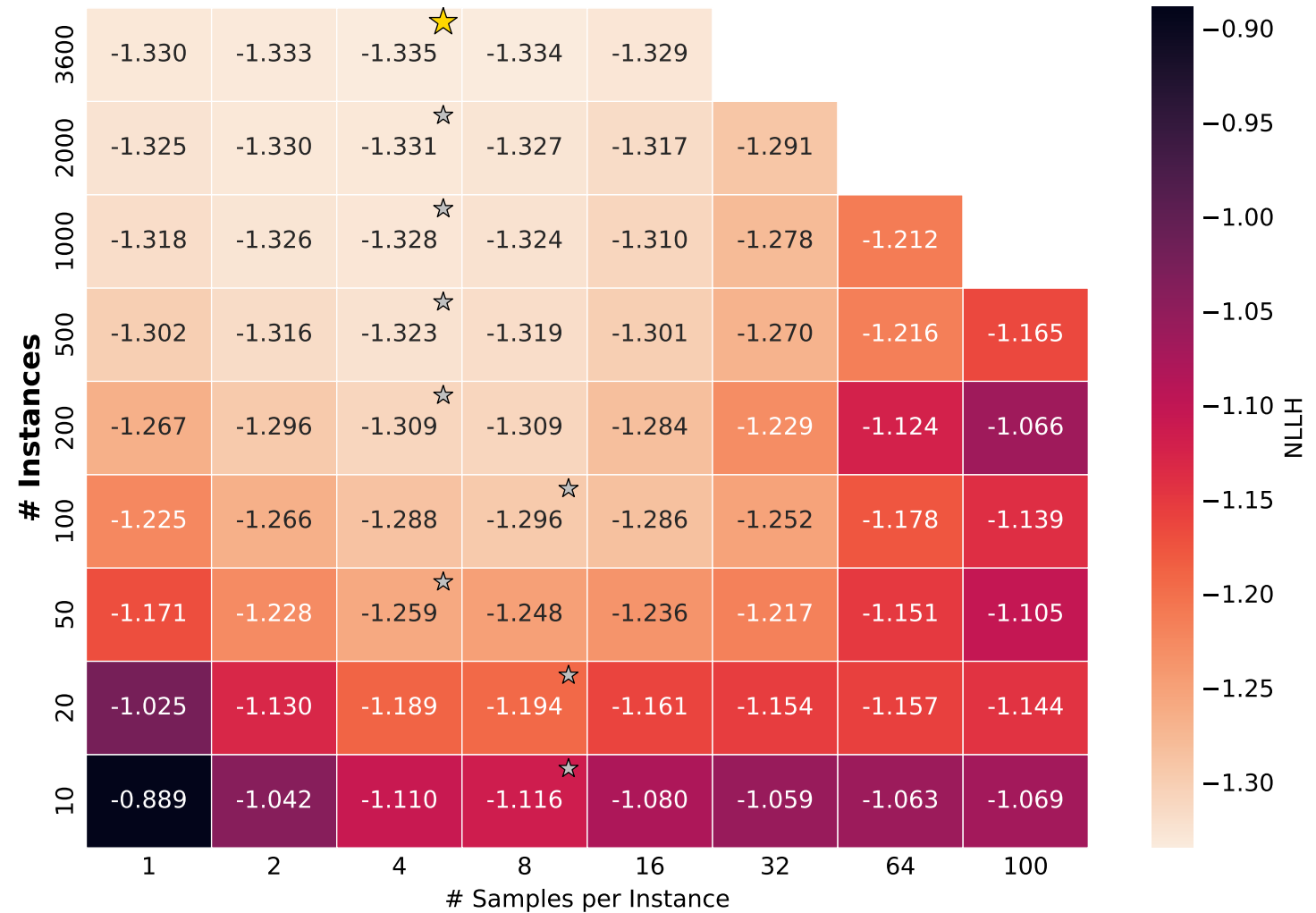
lpg-zeno (NLLH)
