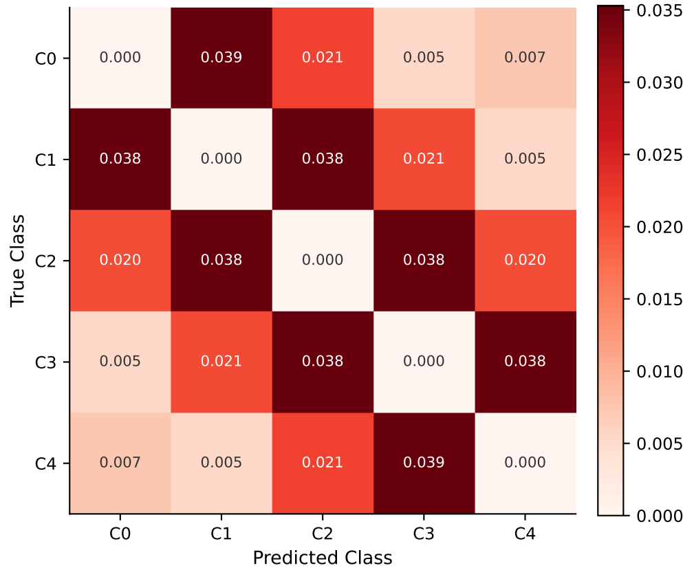
TabPFN RankCode
