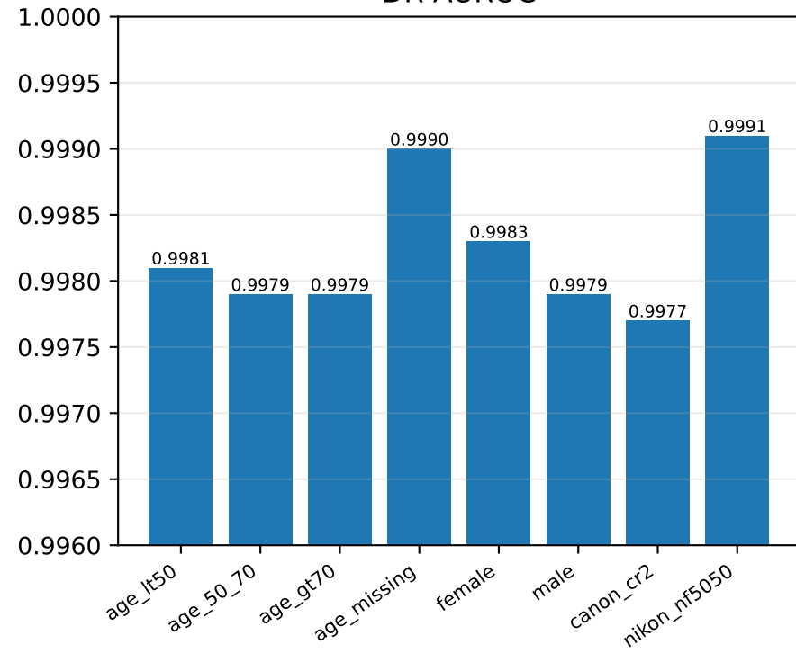
DR AUROC
