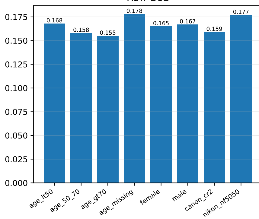
Raw ECE
