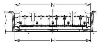
K-K (SCALE 1:1)
