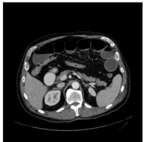
CT slice (224×224)
