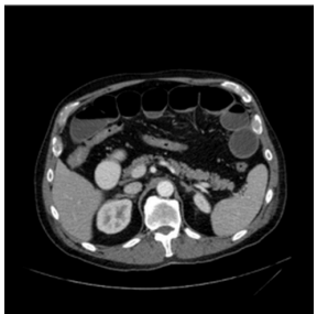
CT slice (224×224)
