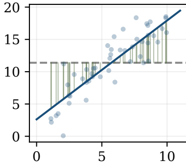
SS_{\text{reg}} : explained
