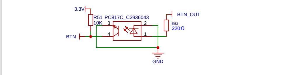
BUTTON DECOUPLER
