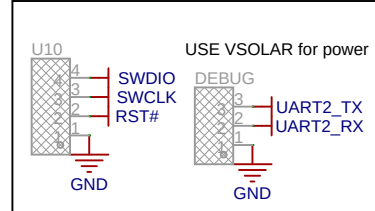
STLINK_PORT
