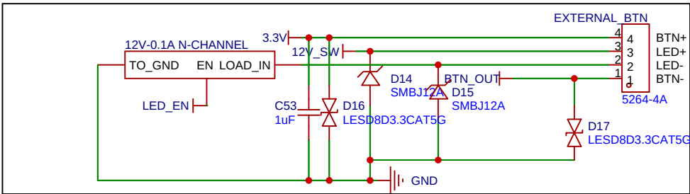
BUTTON DECOUPLER
