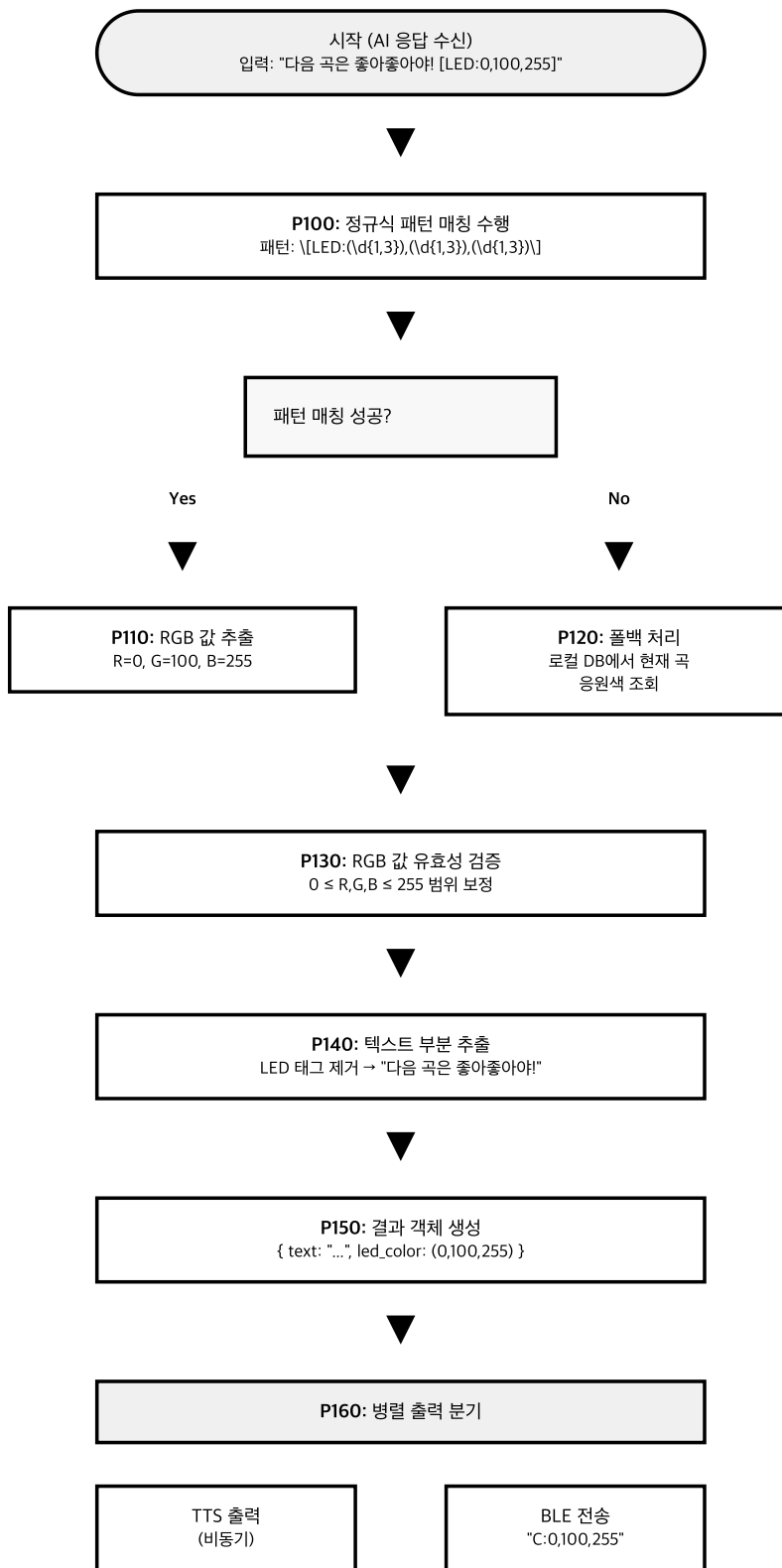
【도 5】 AI 응답 파싱 알고리즘 흐름도
