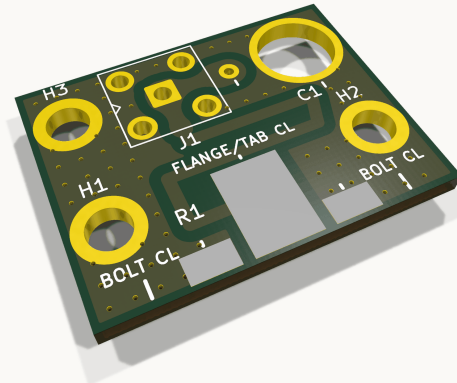
RF-TERM-150W 2 LAYERS · 26 × 20 MM · 6 FOOTPRINTS PACKAGE READY
