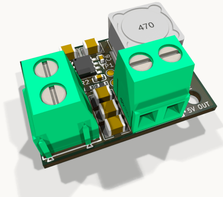
BB-BUCK 2 LAYERS · 35 × 25 MM · 20 FOOTPRINTS
