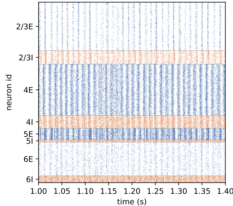
NEST
