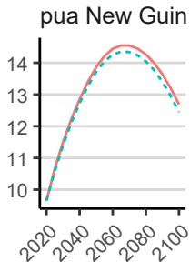
SSP1
