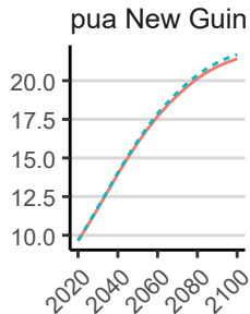
SSP4
