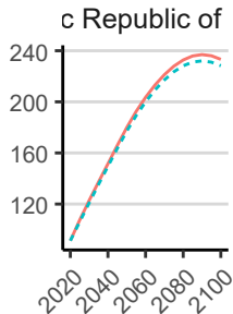
SSP1
