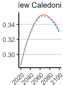
SSP1
