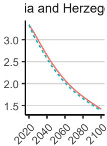
SSP5
