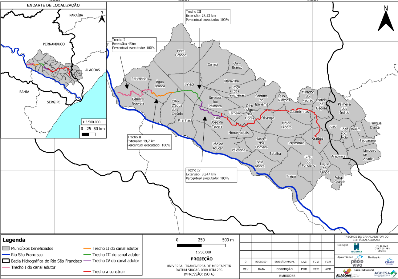
Figura 4.3 – Trechos construídos do Canal Adutor do Sertão Alagoano
