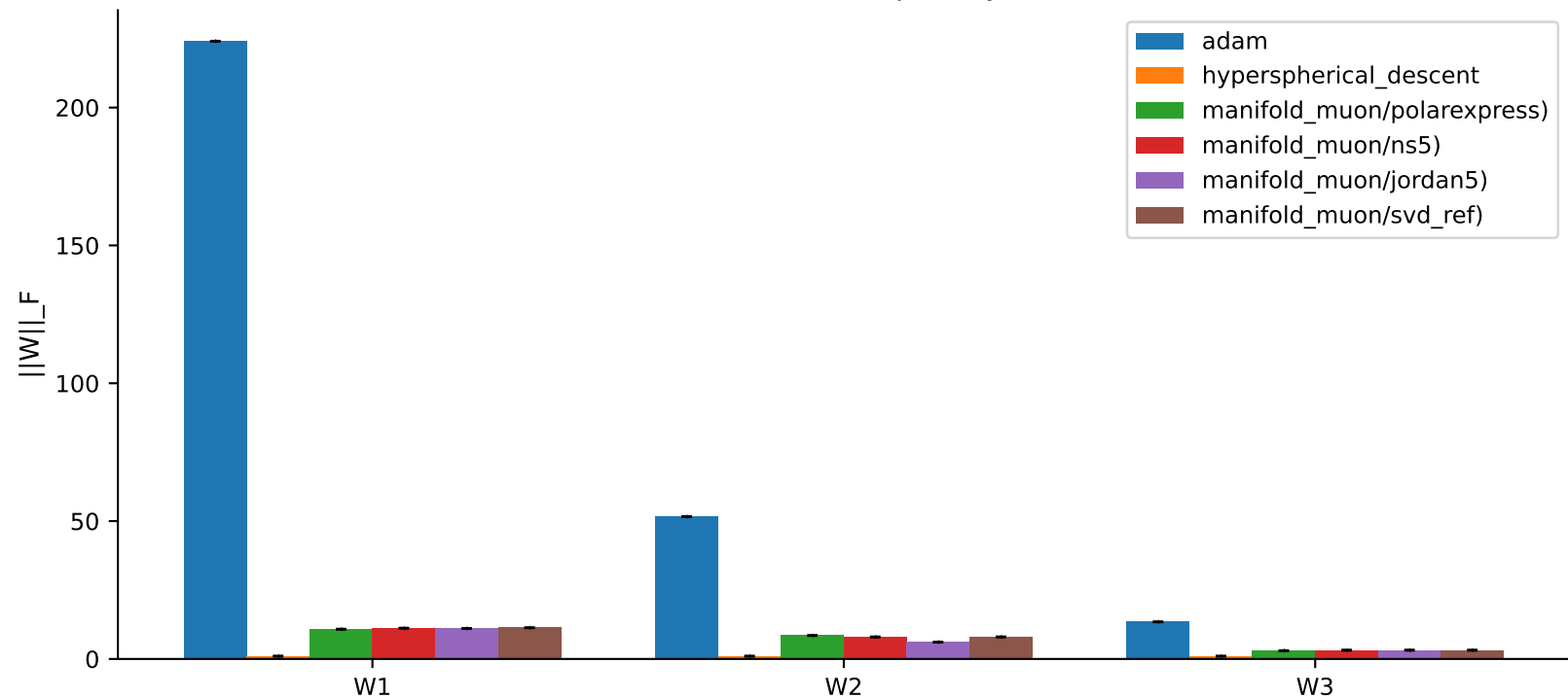
Frobenius Norms per Layer
