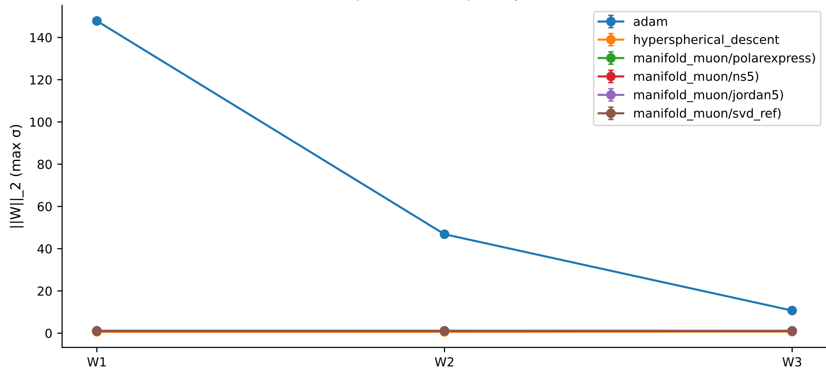
Spectral Norms per Layer
